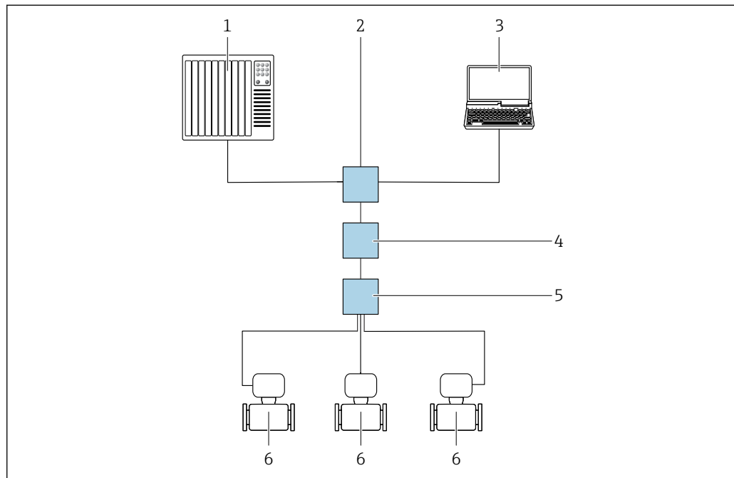
図 20 Modbus TCP over Ethernet-APL プロトコル経由のリモート操作オプション（アクティブ）
