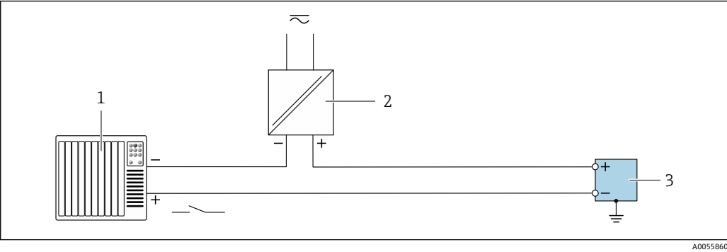
図 14 ステータス入力の接続例
