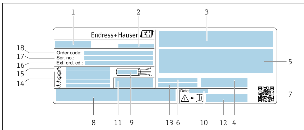
図 2 変換器の銘板の例
