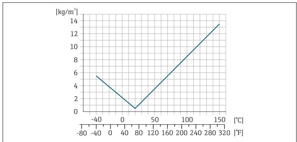
图 41 现场密度校正，例如在+20 °C (+68 °F)时
