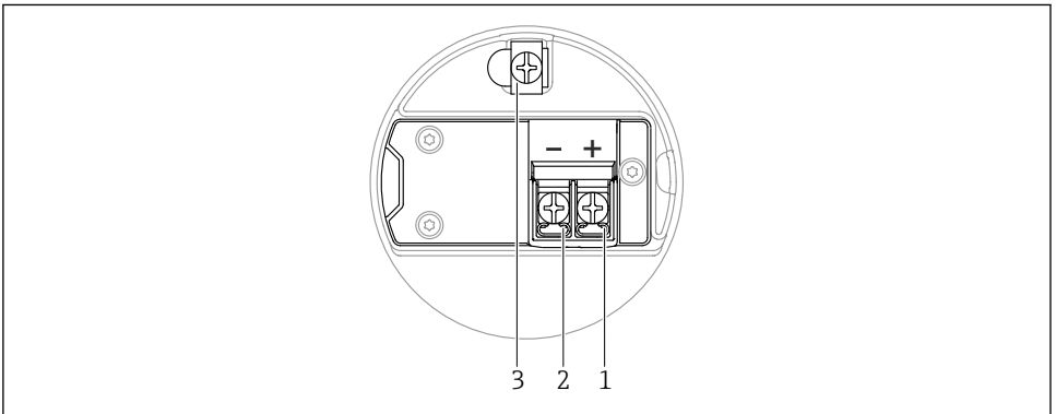
2 연결부의 연결 단자 및 접지 단자
