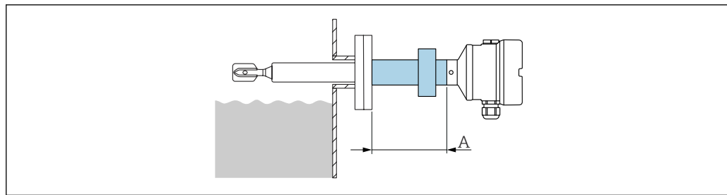
図 40 伸長パイプ用の耐圧防爆対応ガスタイトフィードスルー。測定単位 mm (in)
