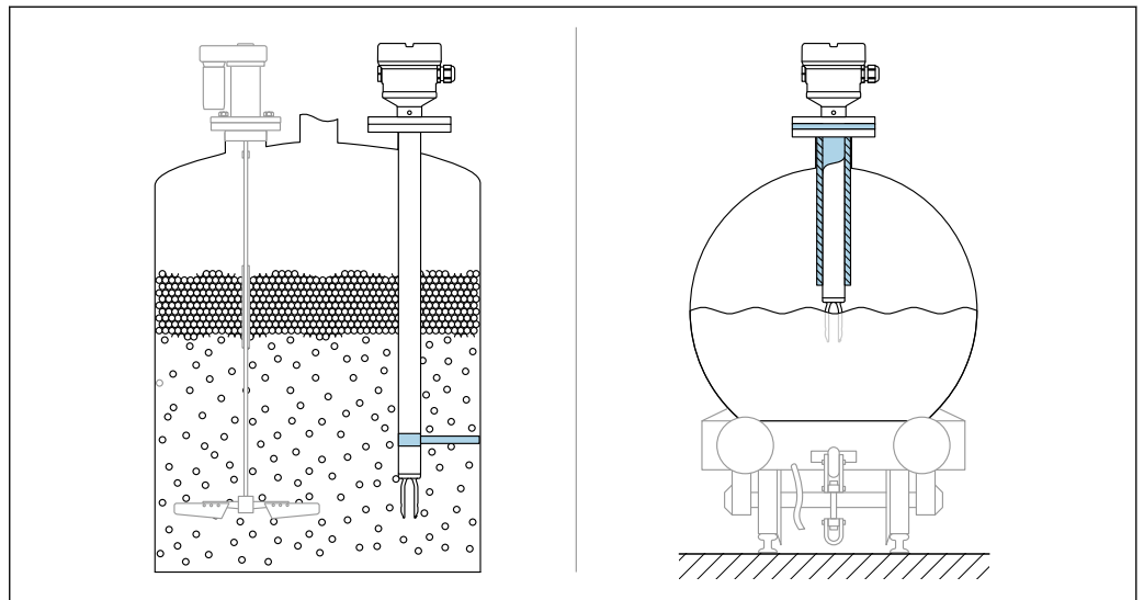
図 31 動的負荷が発生する場合のサポートの例
