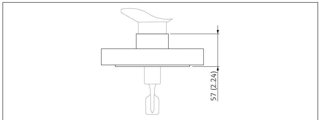
図 44 フランジ付きプロセス接続 (最大高さ仕様)。測定単位 mm (in)
