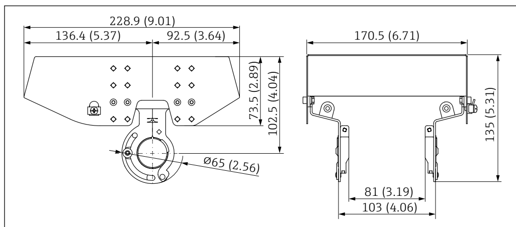
図 52 保護カバー、SUS 316L 相当、XW112 の寸法。測定単位 mm (in)
