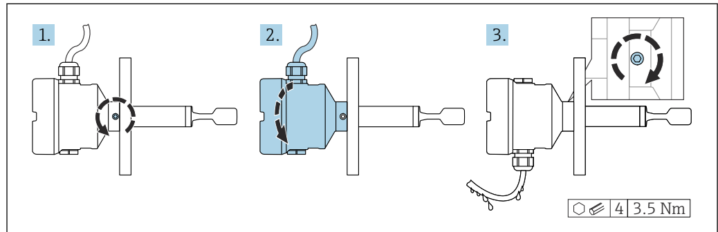
図 29 外部のロックネジおよびドリッブループ付きハウジング
