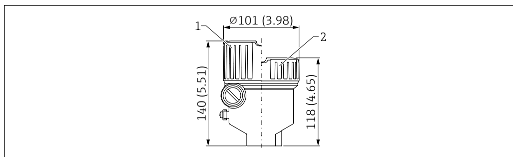
36 シングルコンパートメントハウジング、アルミニウム、コーティングの寸法（Ex d/XP、粉塵防爆仕様）。測定単位 mm (in)
