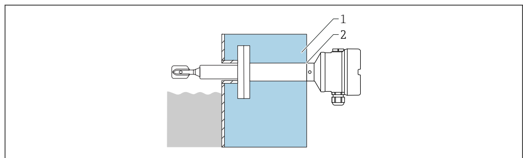
図 30 断熱材付きタンクへの設置（例：温度セパレータを使用した場合）
