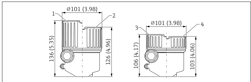
図 35 シングルコンパートメントハウジング、アルミニウム、コーティングの寸法。測定単位 mm (in)
