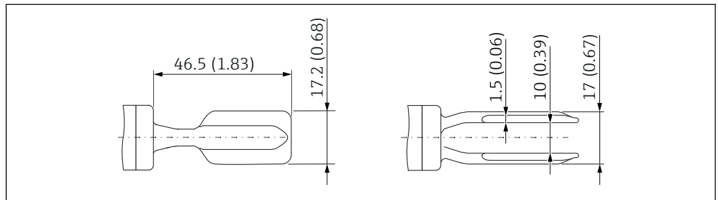
図 43 エナメルコーティング仕様の音叉部。測定単位 mm (in)
