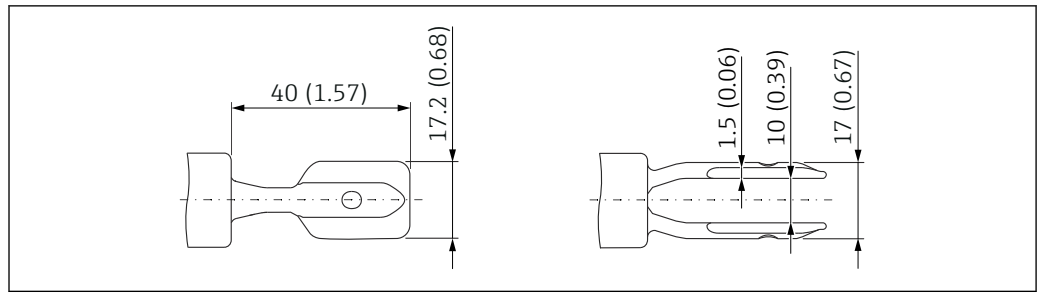
図 42 プラスチックコーティング仕様の音叉部 (ECTFE、PFA)。測定単位 mm (in)
