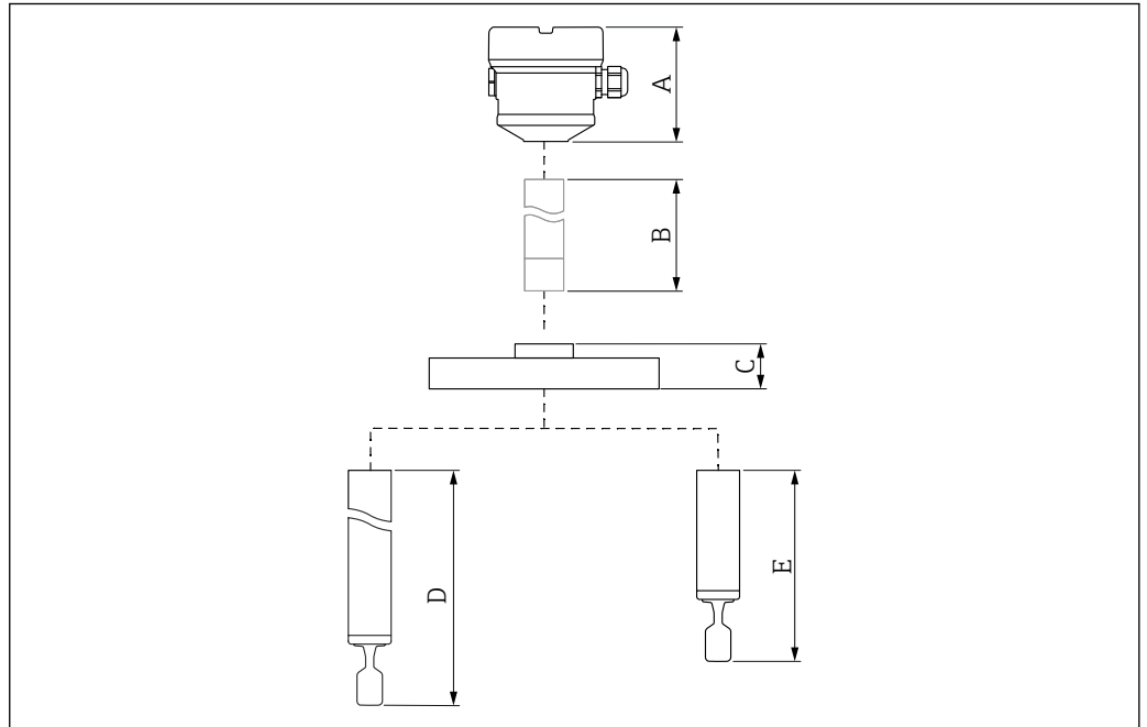
図 33 本体高さを計算するための構成品
