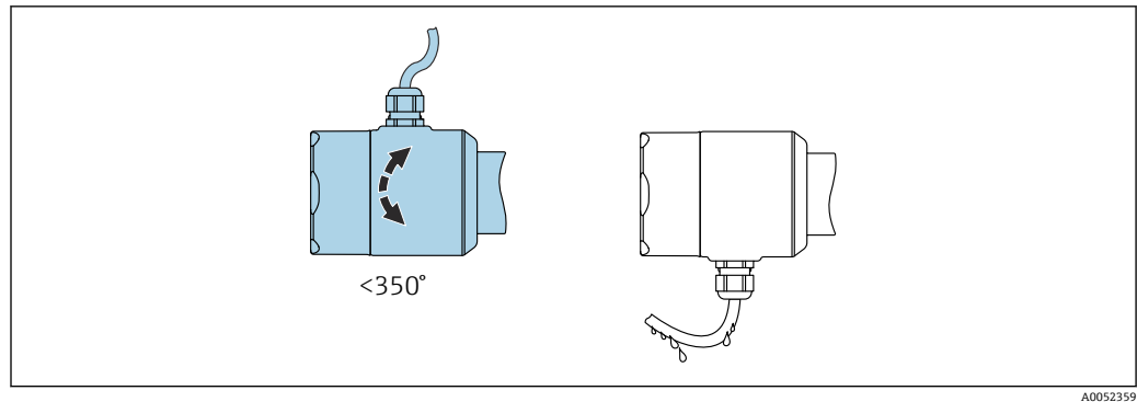
図 28 ロックネジのないドリッブループ付きハウジング
