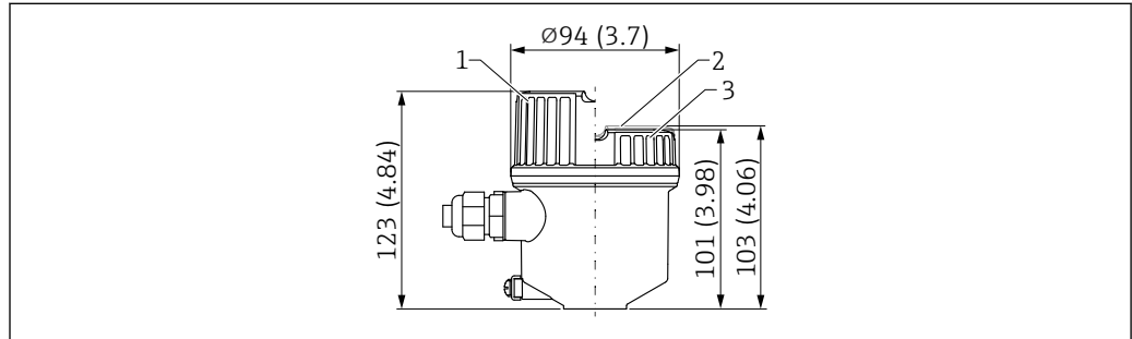
図 34 シングルコンパートメントハウジング、プラスチックの寸法。測定単位 mm (in)
