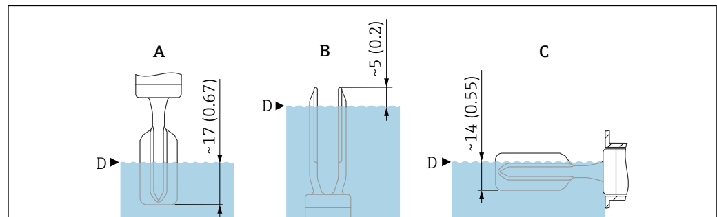
図 18 標準的なスイッチポイント、エナメルコーティング仕様の音叉部、寸法（コーティング厚さを含まず）。測定単位 mm (in)
