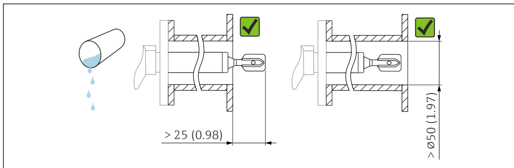
図 22 低粘度液体の設置例。測定単位 mm (in)
