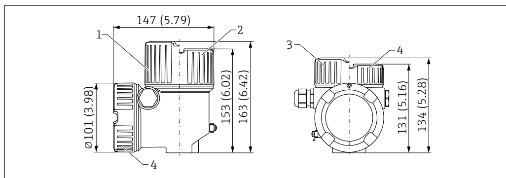
図 39 デュアルコンパートメントハウジング、L字型、アルミニウム、コーティングの寸法 (Ex d/XP、粉塵防爆仕様)。測定単位 mm (in)
