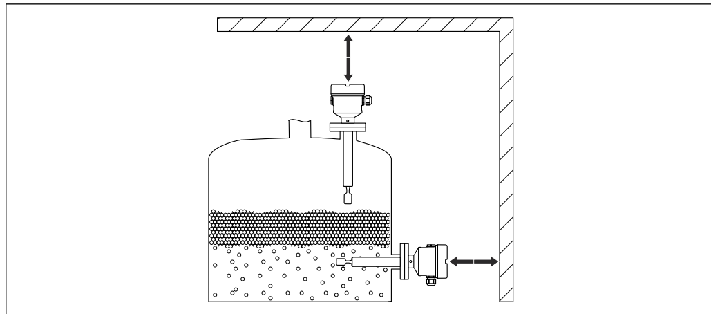
図 25 間隔を考慮すること
