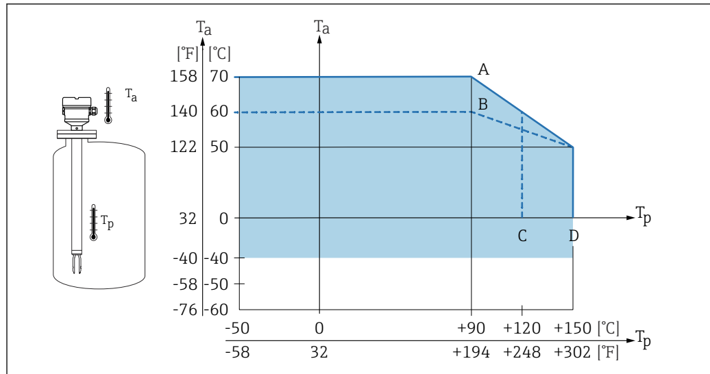
図 32 容器内のプロセス温度 T_p に応じたハウジングの許容周囲温度 T_a
