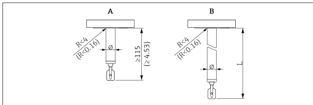
図 41 プローブ型式: ショートパイプ、伸長パイプ。測定単位 mm (in)
