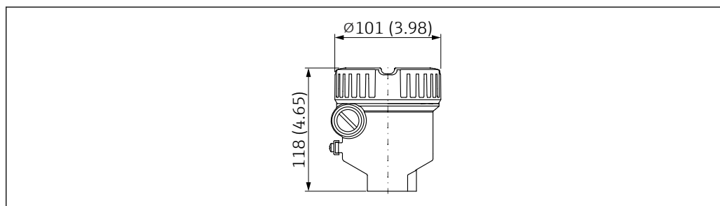
37 シングルコンパートメントハウジング、SUS 316L 相当の寸法（Ex d/XP および 粉塵防爆仕様、ハウジングカバーの窓なし）。測定単位 mm (in)
