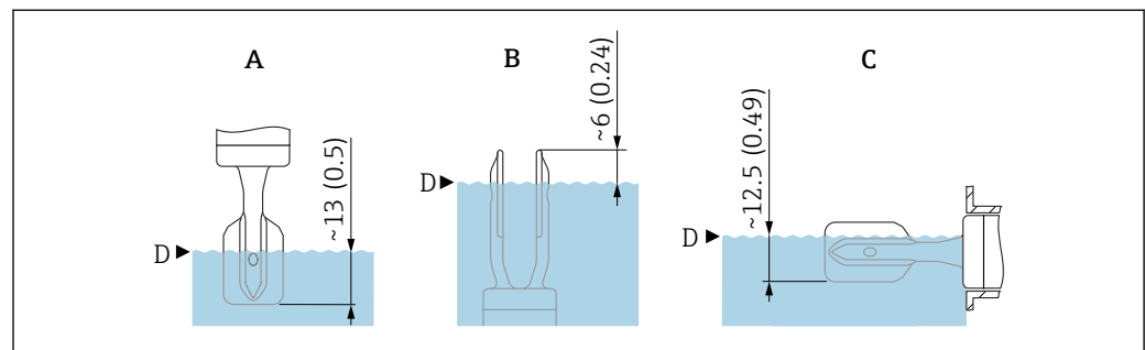
図 17 標準的なスイッチポイント、プラスチックコーティング仕様の音叉部（ECTFE、PFA）、寸法（コーティング厚さを含まず）。測定単位 mm (in)
