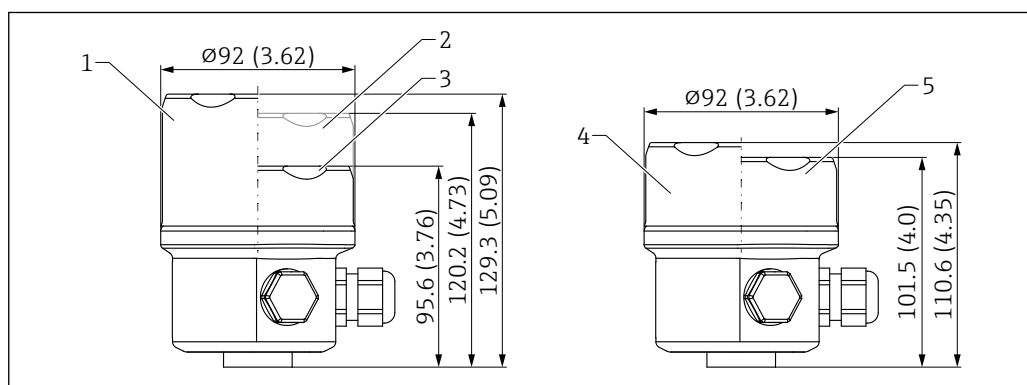
38 シングルコンパートメントハウジング、SUS 316L 相当、サニタリ仕様の寸法。測定単位 mm (in)
