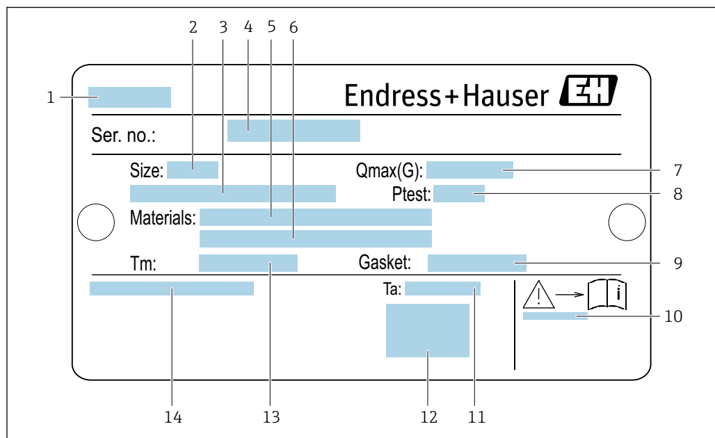
1 Exemple d'une plaque signalétique de capteur
