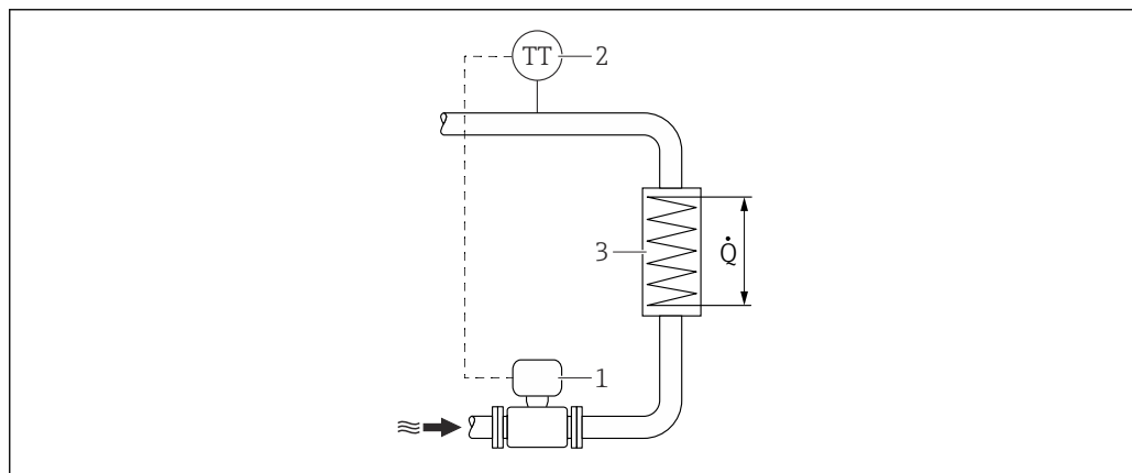
5 Disposition pour la mesure de différence de chaleur dans de la vapeur saturée et de l'eau
