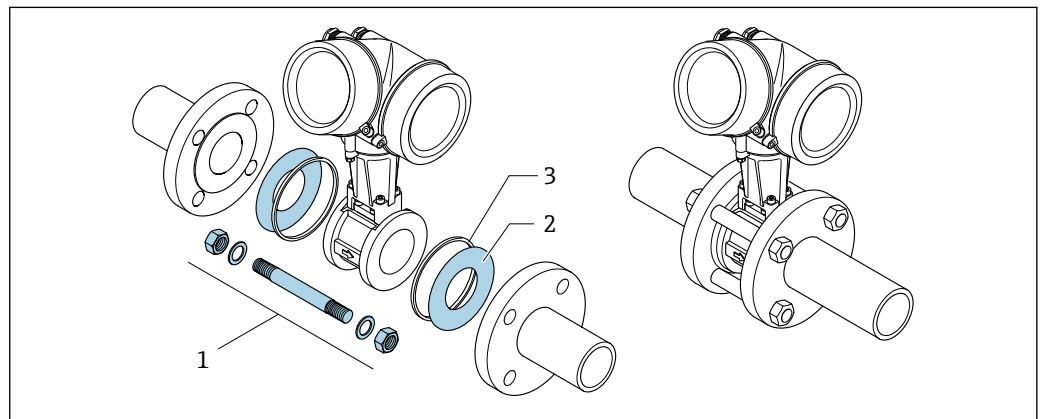
6 Kit de montage pour version entre brides
