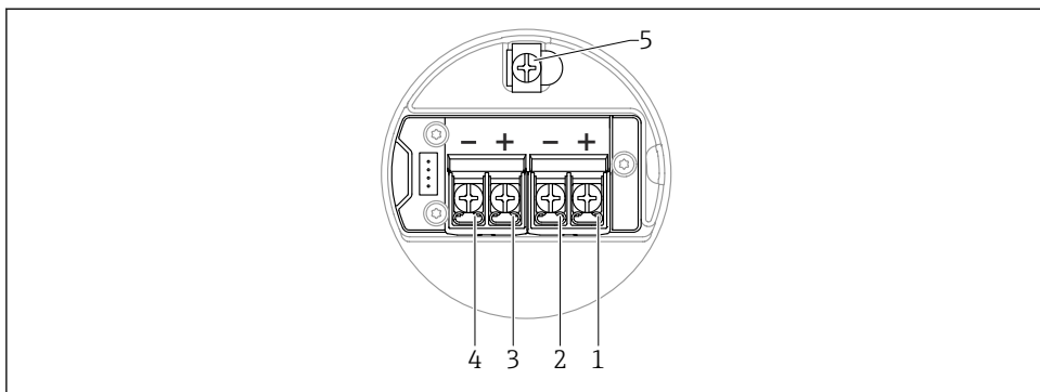
17 Klemmenbelegung im Anschlussraum; 4 ... 20 mA HART, Schaltausgang; Zweikammergehäuse L-Form
