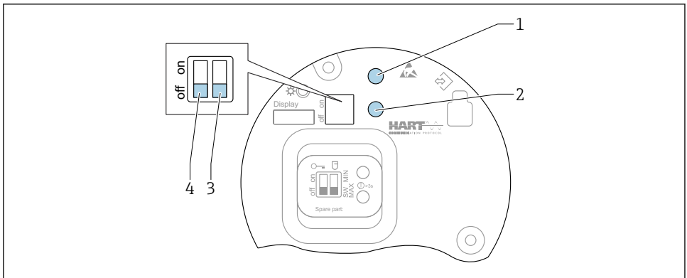
18 Bedientasten und DIP-Schalter auf dem HART Elektronikeinsatz
