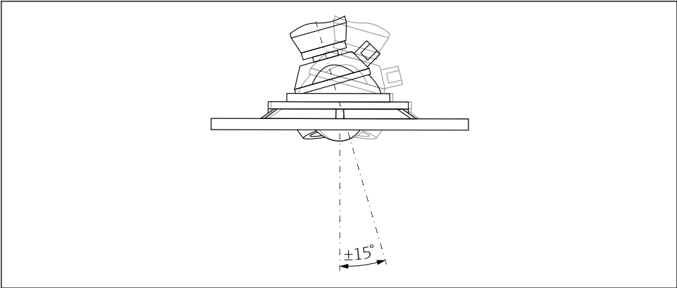
2 Antenne frontbündig mit Ausrichtvorrichtung
