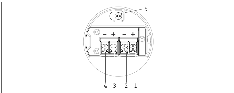
13 Klemmenbelegung im Anschlussraum; 4 ... 20 mA HART + 4 ... 20 mA analog; Zweikammergehäuse
