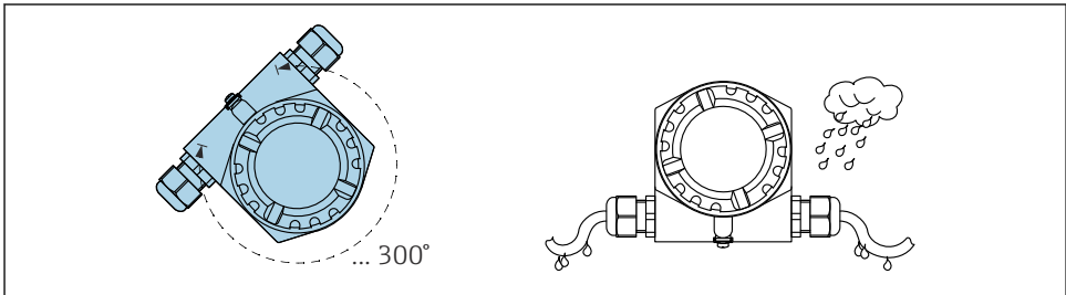
▣ 14 Kućište bez postavljenog vijka; formira petlju za kapanje na kabelu
