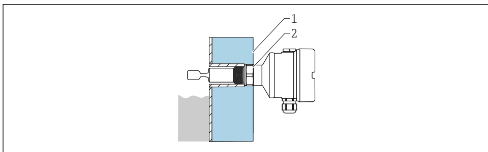
▣ 3 Primjer posude s toplinskom izolacijom
