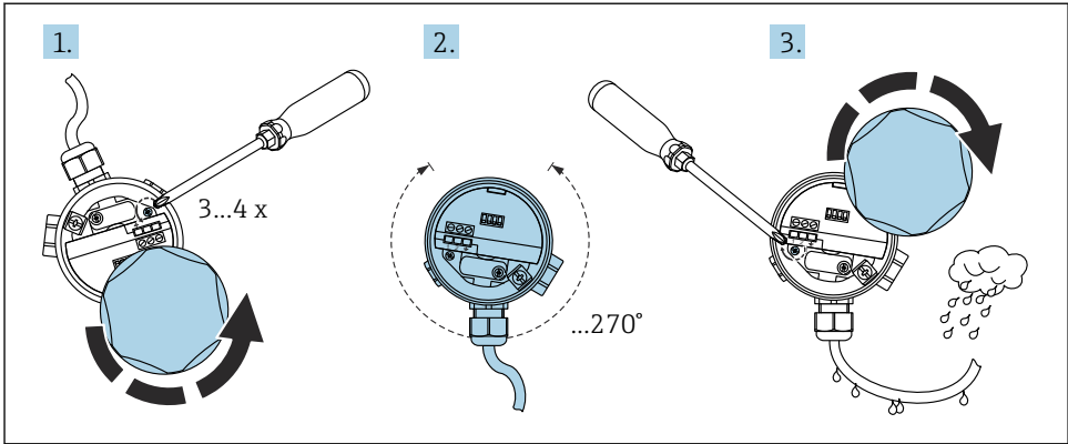
▣ 13 Kućište s vijkom za zaključavanje; formira petlju za kapanje na kabelu
