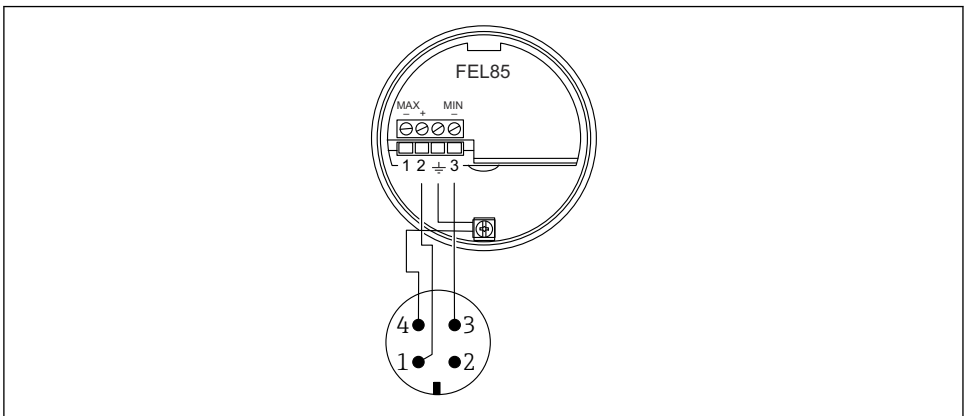
17 Raspored priključaka s konektorom M12, način rada s minimalnom detekcijom
