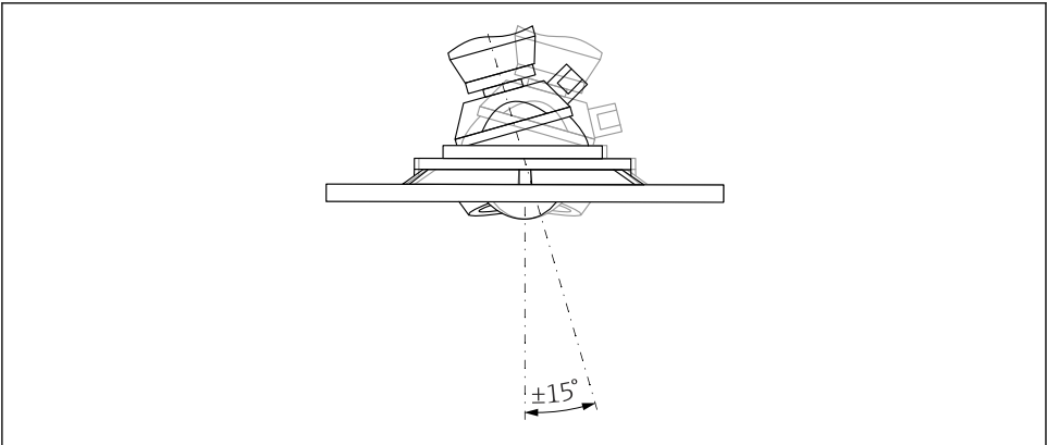
2 Soporte para montaje enrasado de la antena con unidad de alineación
