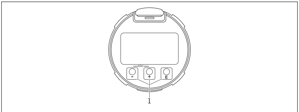
12 Indicador gráfico con teclas de configuración ópticas (1)
