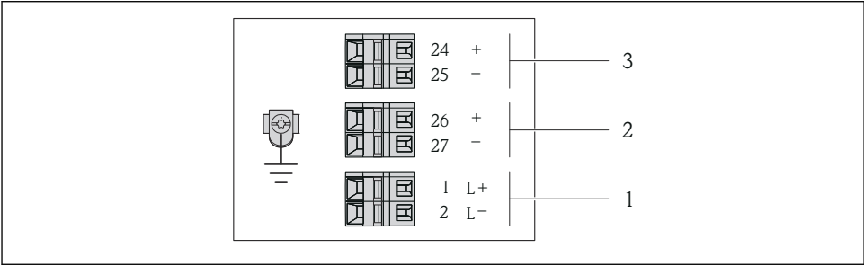
6 Occupation des bornes 4-20 mA HART avec sortie impulsion/fréquence/tor
