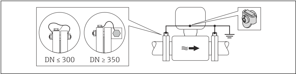
13 Compensation de potentiel via la borne de terre et la bride de conduite
