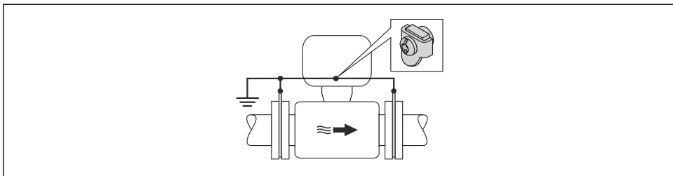
14 Compensation de potentiel via la borne de terre et les disques de masse
