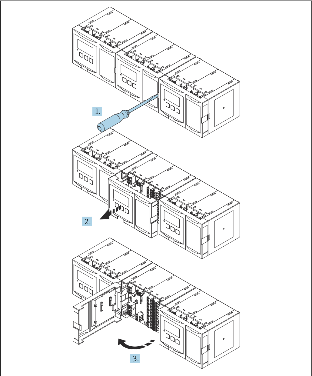
20 操作接线腔：多台 DIN 导轨盘装型外壳设备并排安装
