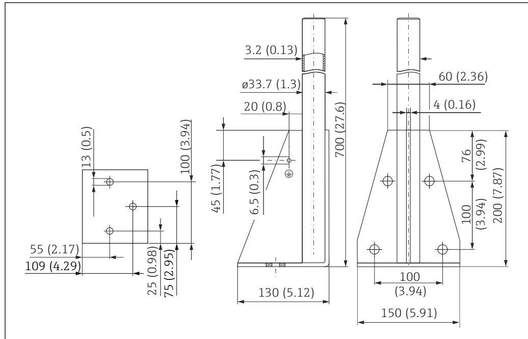
图 53 外形尺寸。测量单位 mm (in)
