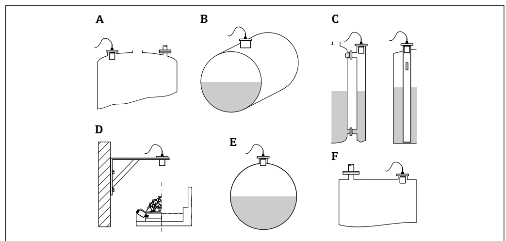
图 40 罐体形状
