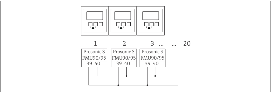
图 30 多个 FMU90/FMU95 变送器的同步
