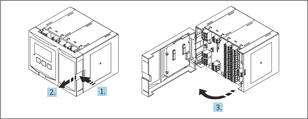
19 操作接线腔：单台 DIN 导轨盘装型外壳设备
