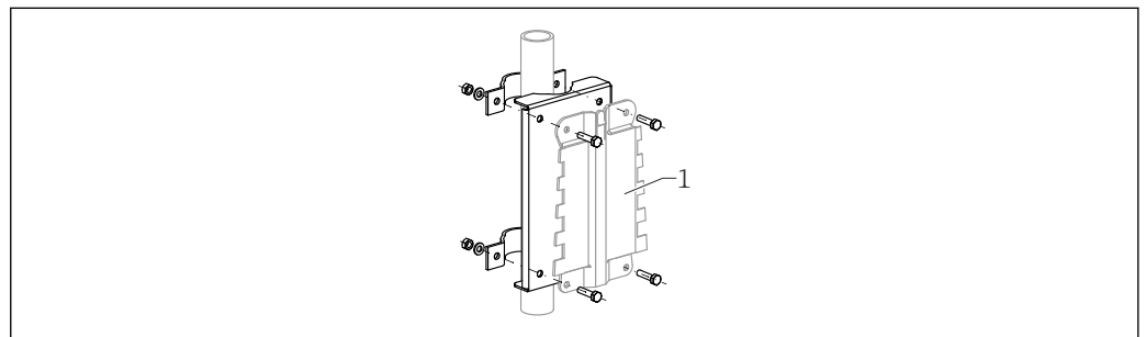
图 52 安装板，适用聚碳酸酯现场型外壳
