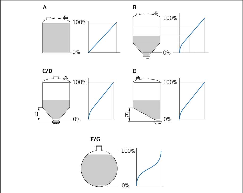
图 42 线性化类型
