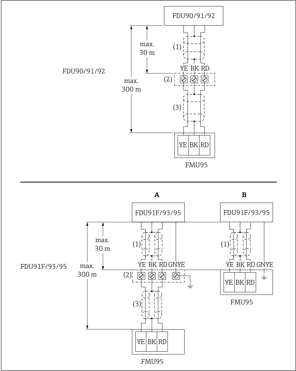
图 25 传感器 FDU9x 的接线图; YE: 黄色; BK: 黑色; RD: 红色; BU: 蓝色; BN: 棕色; GNYE: 绿色/黄色
