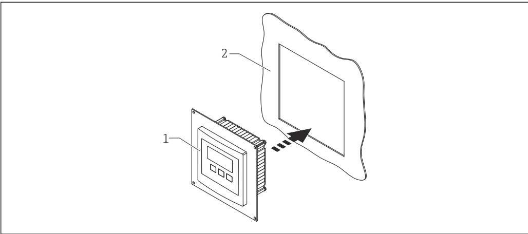
图 55 使用安装适配板
