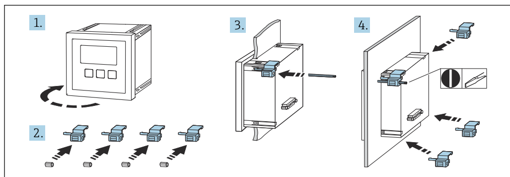
图 15 安装分离型显示与操作单元
