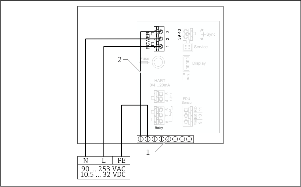
22 聚碳酸酯现场型外壳内的电源连接
