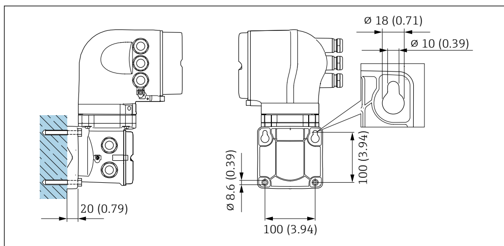
14 Единицы измерения: мм (дюймы)
