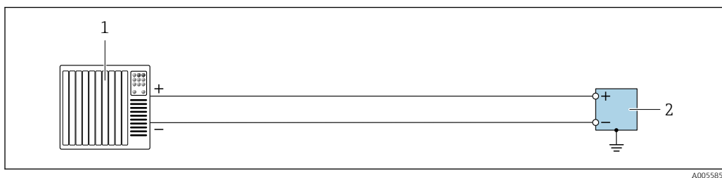
21 Пример подключения для импульсного/частотного/релейного выхода (активного)
