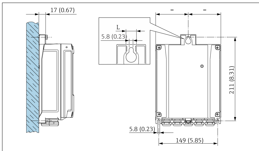
13 Ед. изм.: мм (дюймы)
