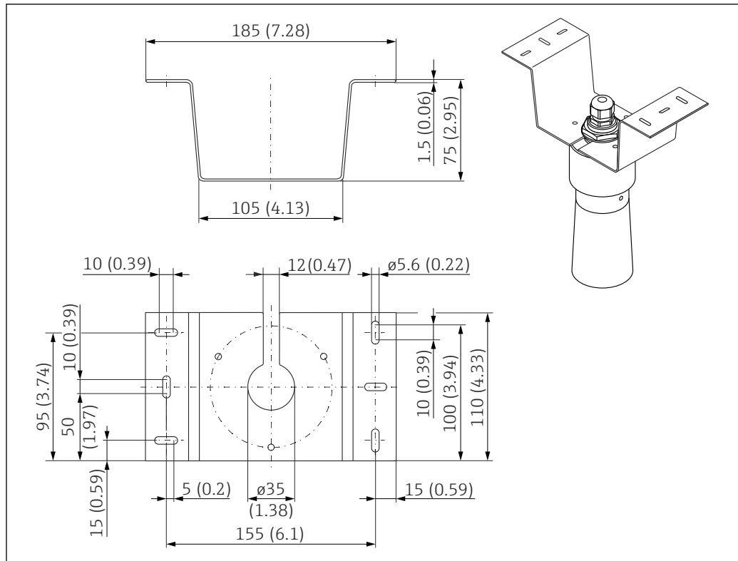
19 Montažni nosač za montažu na strop. Mjerna jedinica mm (in)
