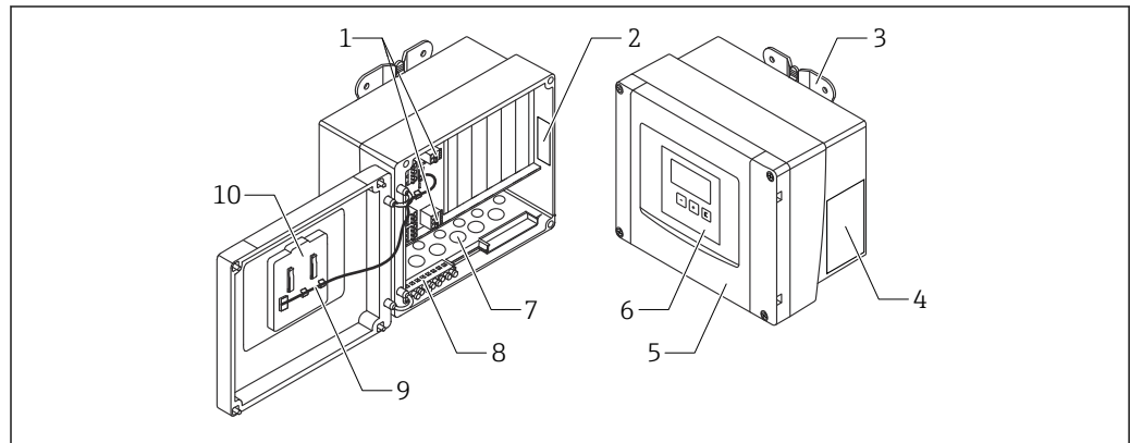
i 1 Parti di Prosonic S nella custodia da campo in polycarbonato
