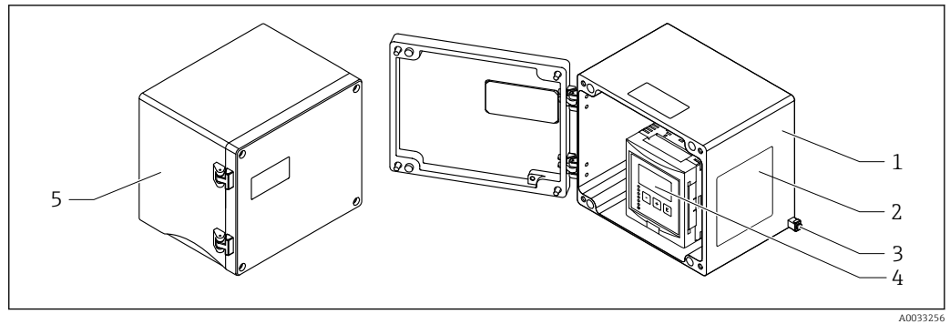
2 Parti del Prosonic S nella custodia da campo in alluminio
