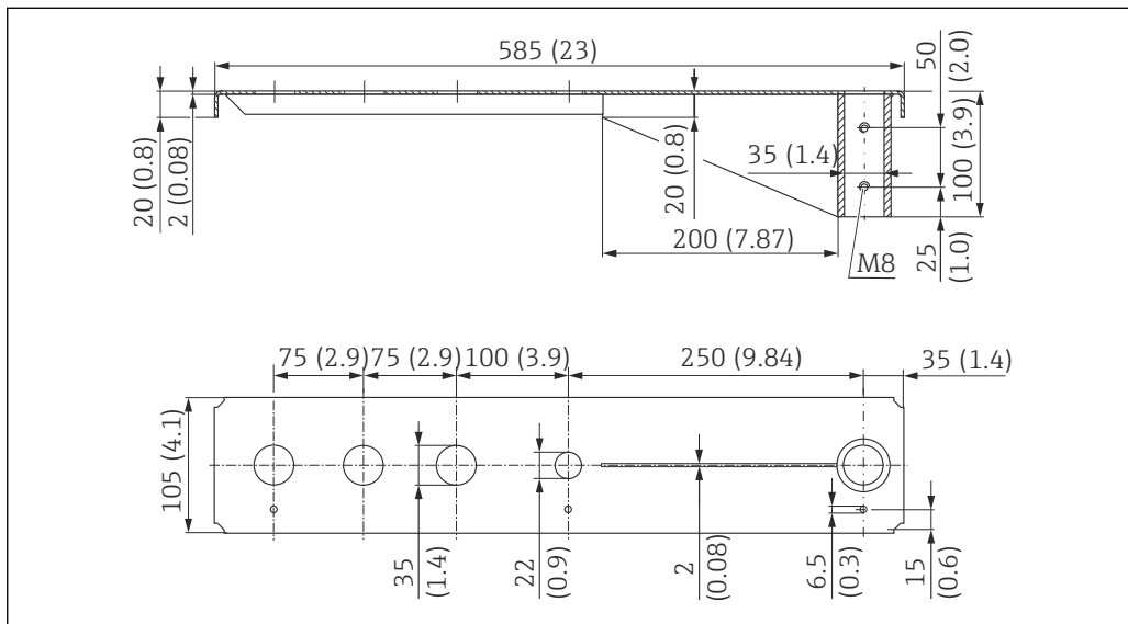
17 Rozměry. Jednotka měření mm (in)
