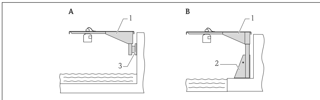
16 Montáž senzoru s konzolovým ramenem
