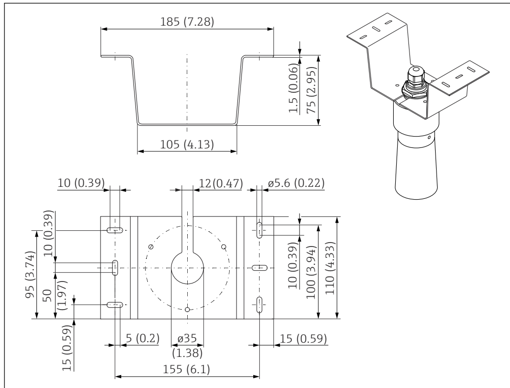
22 Montážní držák pro stropní montáž. Jednotka měření mm (in)
