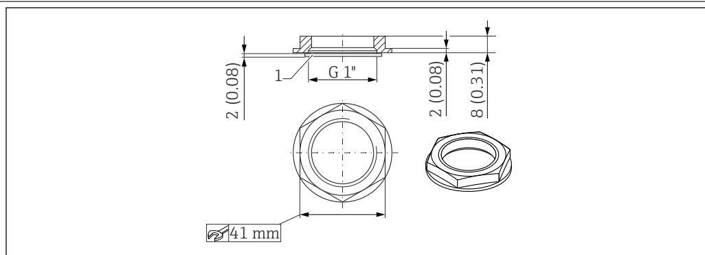
11 Kontramatice; rozměry. Jednotka měření mm (in)
