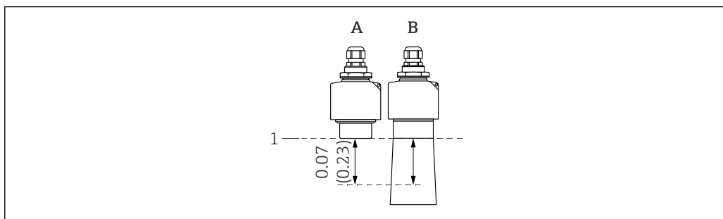
1 Blokovací vzdálenost ultrazvukového senzoru. Technická jednotka m (ft)
