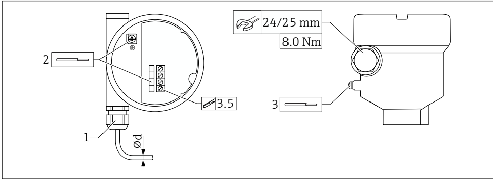
図 16 カップリングの例（電線口、エレクトロニックインサートと端子）
