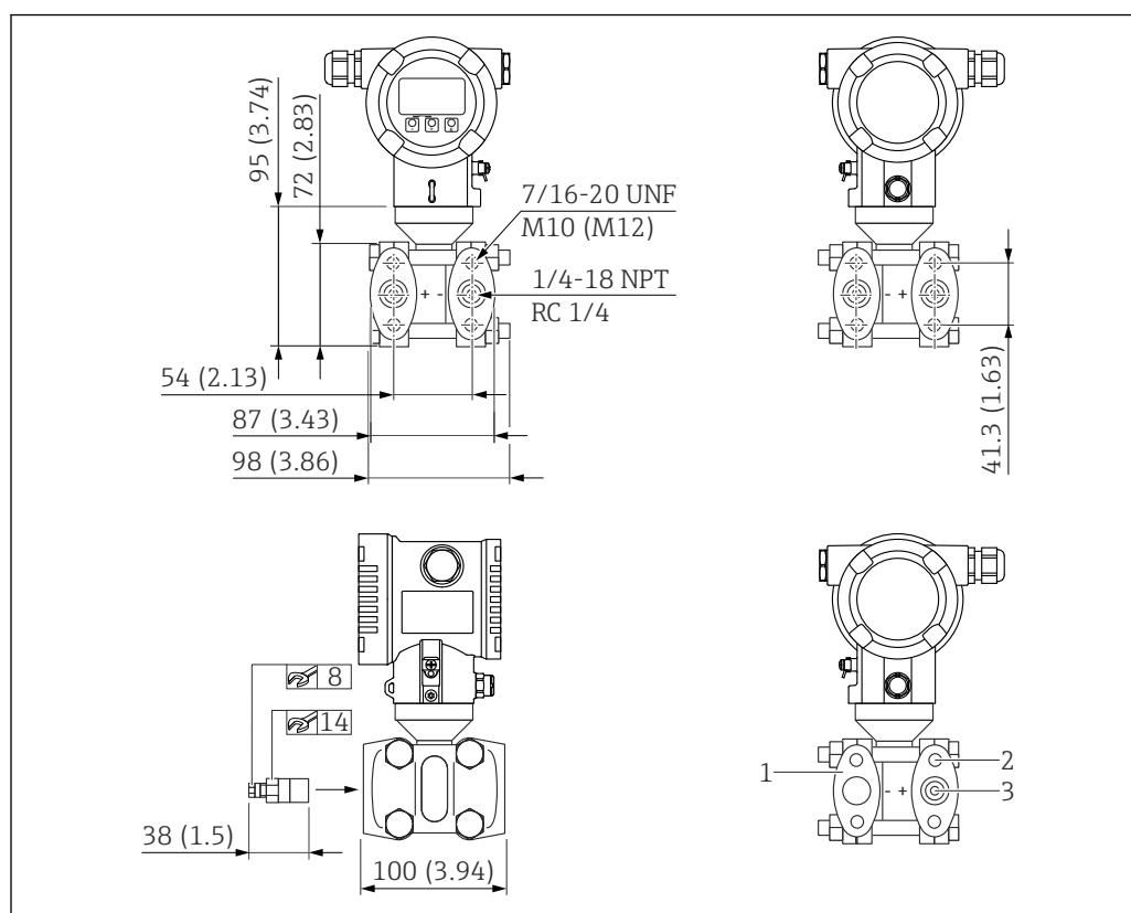
図 8 正面図、左側面図、右側面図。測定単位 mm (in)
