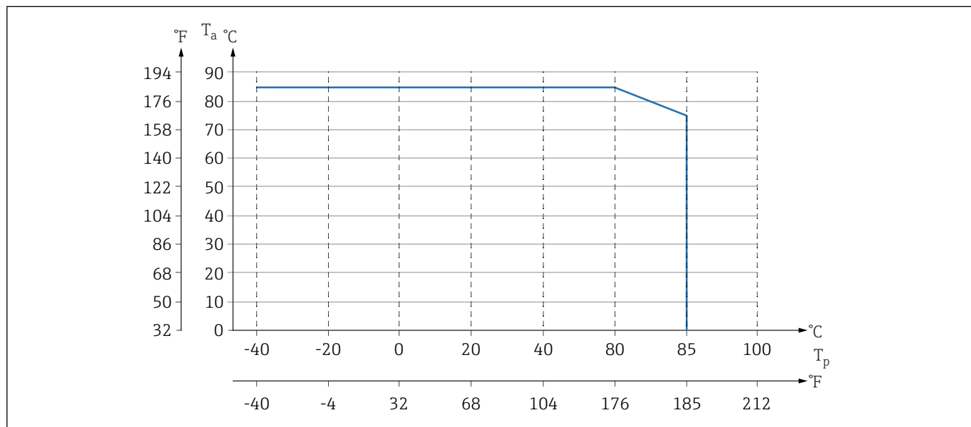
図 7 断熱材を使用しない垂直取付時の値
