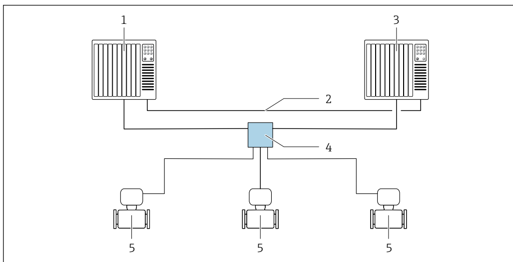
36 Пример компоновки резервируемой системы (S2): топология «звезда»
