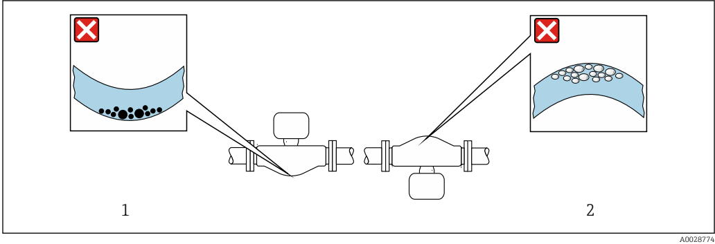
☒ 7 Монтажное положение датчика с изогнутой измерительной трубкой
