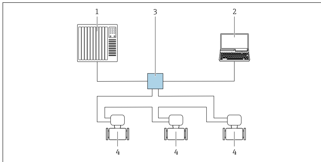
32 Варианты дистанционного управления через сеть PROFINET: топология «кольцо»
