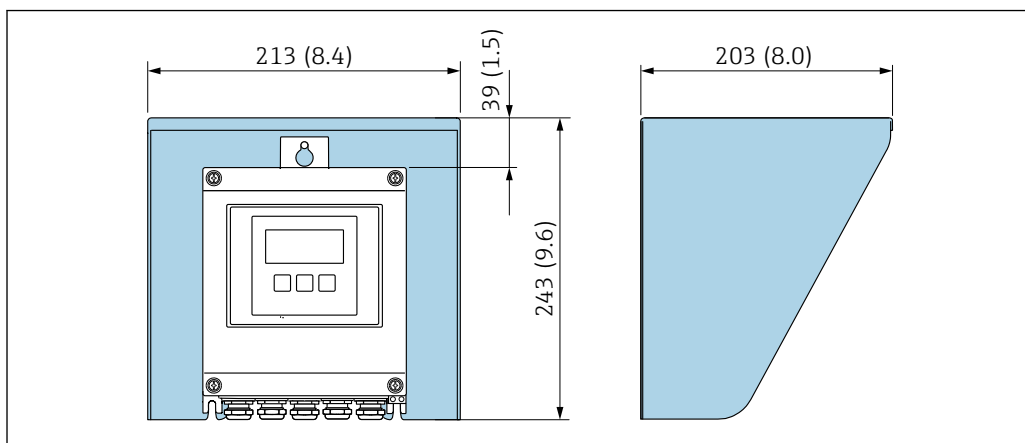
11 Защитный козырек от погодных явлений для Proline 500 – цифровое исполнение; мм (дюймах)
