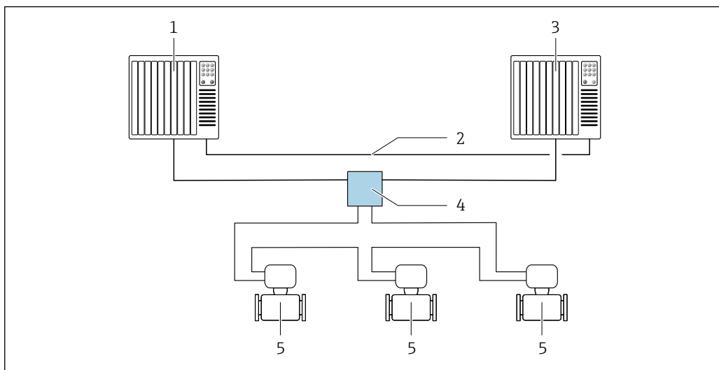
35 Пример компоновки резервируемой системы (S2): кольцевая топология
