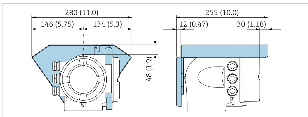
12 Защитный козырек от погодных явлений для Proline 500 – единица измерения- мм (дюймах)
