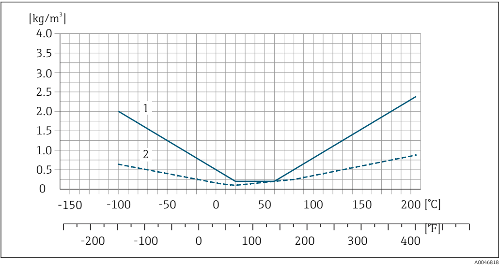
1 Стандартная плотность 2 Высоточное измерение плотности
