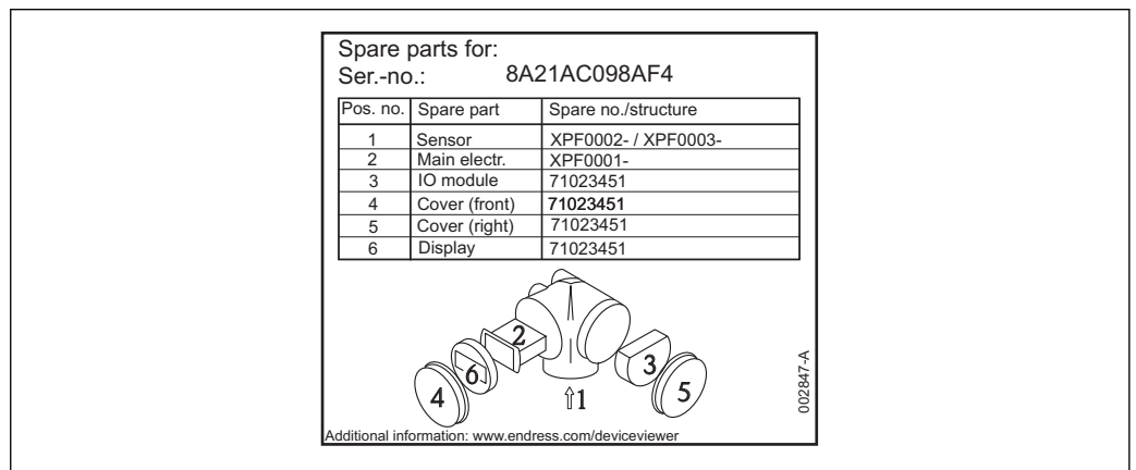
Fig. 22 Esempio di etichetta della parte di ricambio nel coperchio del vano connessioni
