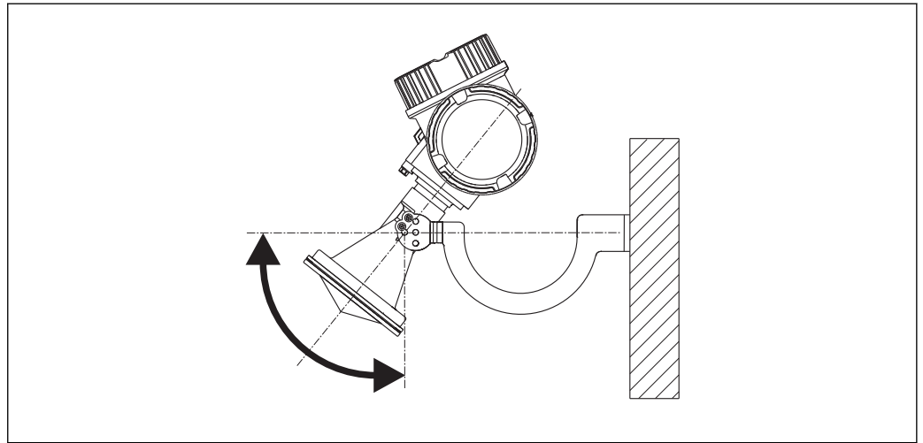
7 Installazione dell'antenna a cono con staffa di montaggio (FMR50/FMR56)
