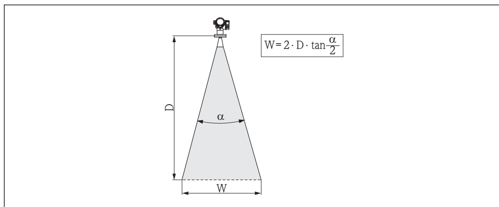
4 Rapporto tra angolo di emissione \alpha , distanza D e diametro del lobo di emissione W
