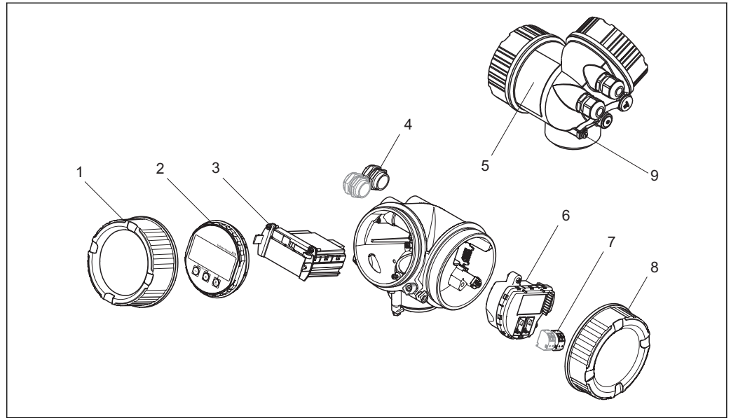
2 Struttura della custodia dell'elettronica
