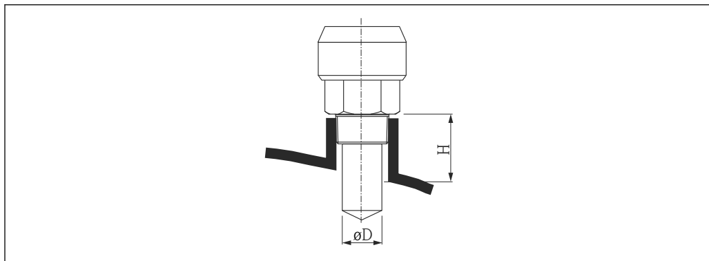
5 Altezza e diametro del tronchetto per antenna a cono, incapsulata (FMR50)
