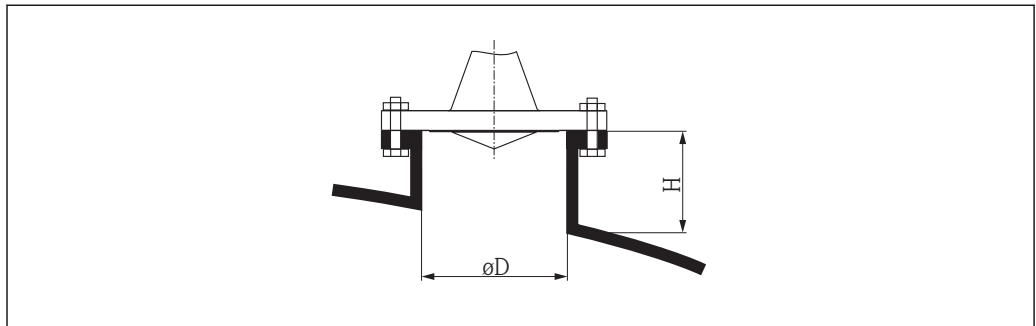
6 Altezza e diametro del tronchetto per antenna a cono con flangia slip-on (FMR50/FMR56)
