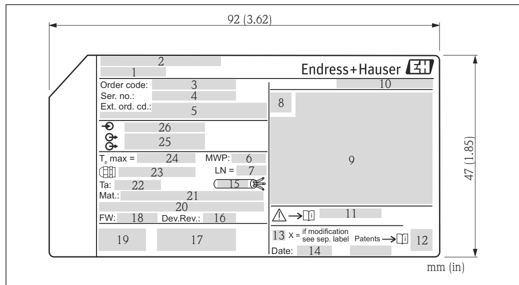
3 Targhetta del misuratore Micropilot
