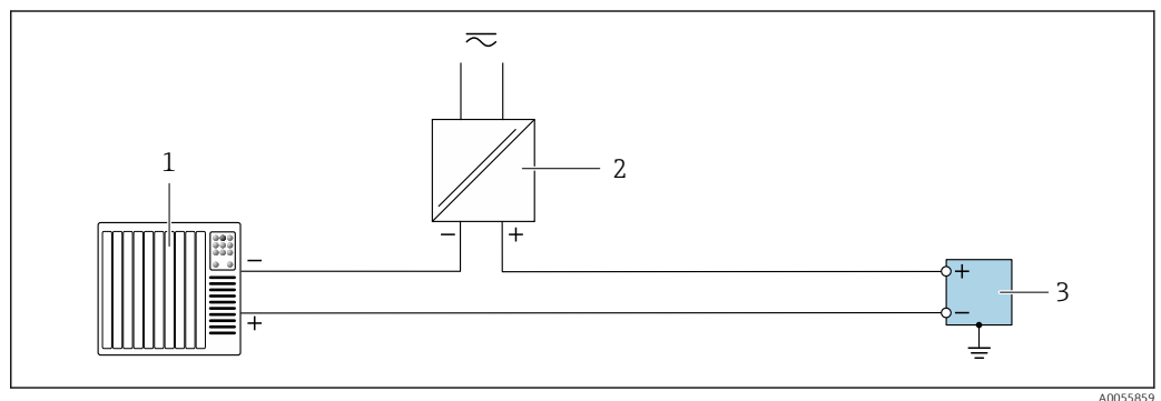
26 Esempio di collegamento per uscita a relè
