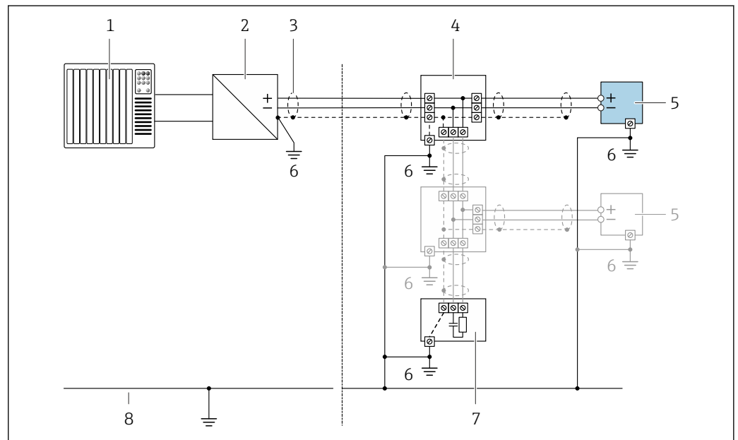
18 Esempio di collegamento per PROFIBUS PA
