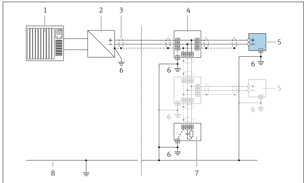
28 Exemple de raccordement pour FOUNDATION Fieldbus
