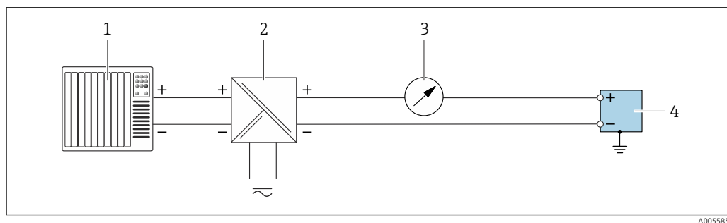
22 Exemple de raccordement pour sortie courant 4 ... 20 mA (passive)
