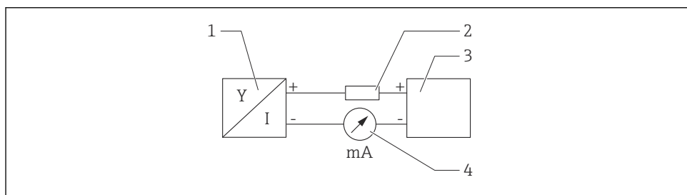
15 Блок-схема подключения HART
