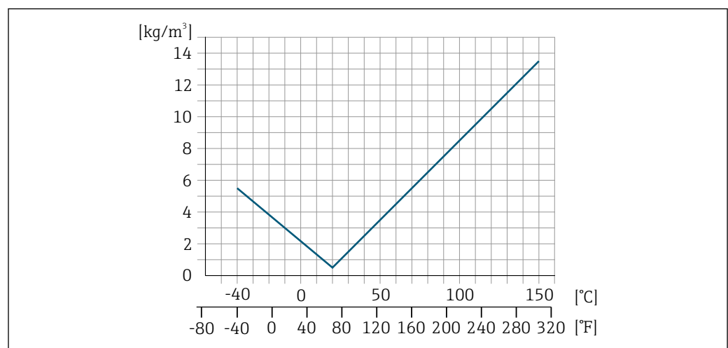
37 Ajuste en campo de la densidad, p. ej., a +20 \text{ }^\circ\text{C} ( +68 \text{ }^\circ\text{F} )
