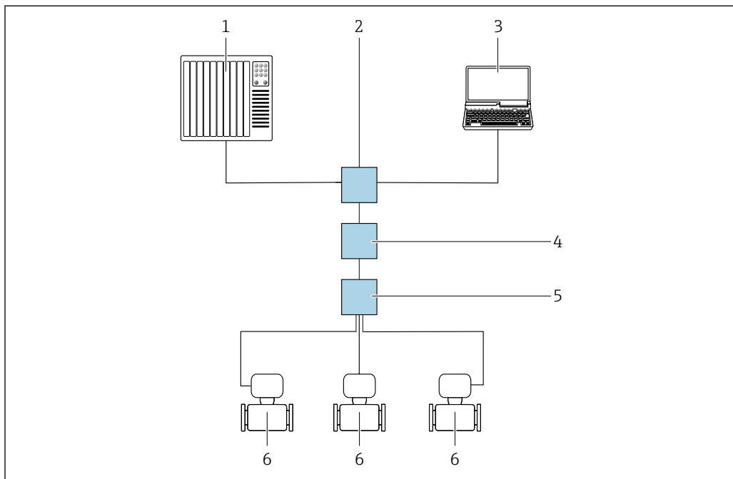
图 20 通过 Modbus TCP + Ethernet-APL 通信进行远程操作（有源信号）
