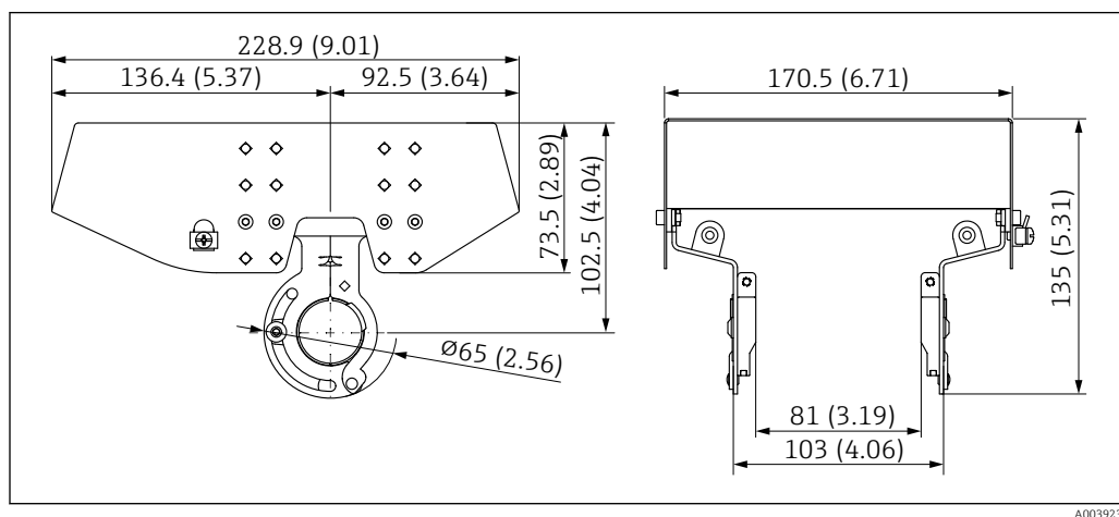
22 Dimensões da tampa de proteção contra tempo, 316L, XW112. Unidade de medida mm (in)
