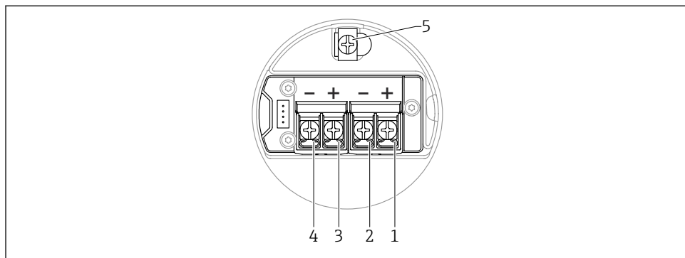
14 Plintadressering i anslutningsfack; 4 ... 20 mA HART; kontaktutgång, L-format hus med dubbla kammare
