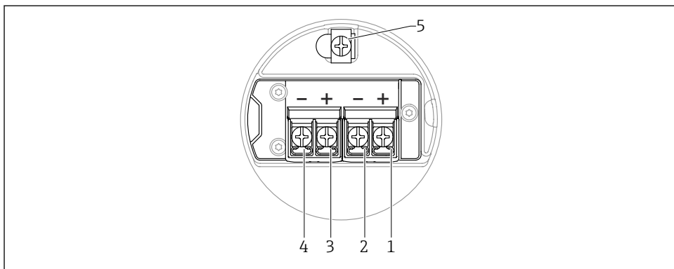
10 Plintadressering i anslutningsfack; 4 ... 20 mA HART + 4 ... 20 mA analog; hus med dubbla kammare
