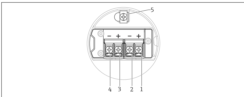
11 Plintadressering i anslutningsfack; 4 ... 20 mA HART, kontaktutgång, hus med dubbla kammare
