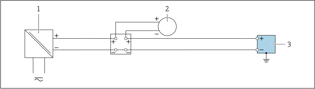
17 接线实例：4 ... 20 mA 电流输入
