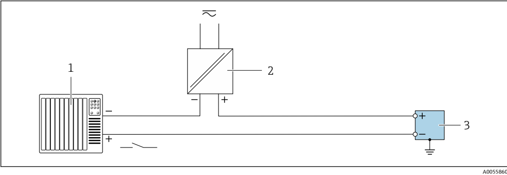
21 状态输入 1 自动化系统，带无源开关量输出（例如 PLC） 2 电源 3 变送器，带状态输入
