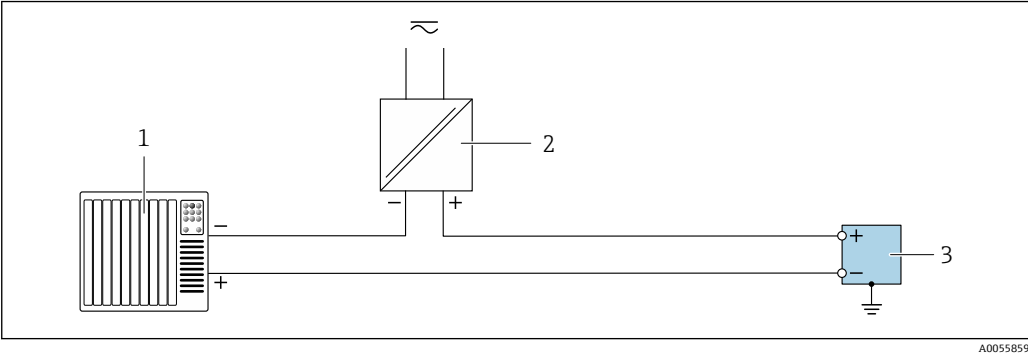
20 接线实例：继电器输出 1 自动化系统，带开关量输入（例如 PLC） 2 电源 3 变送器，带继电器输出
