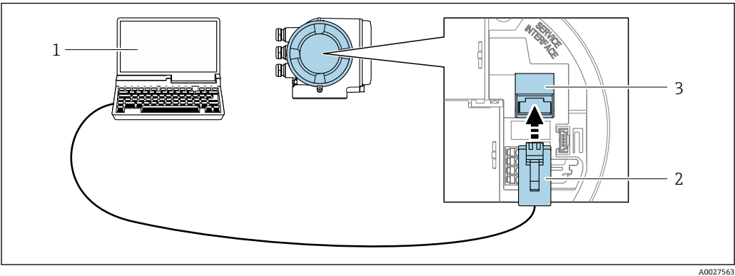
图 30 通过服务接口 (CDI-RJ45) 连接
