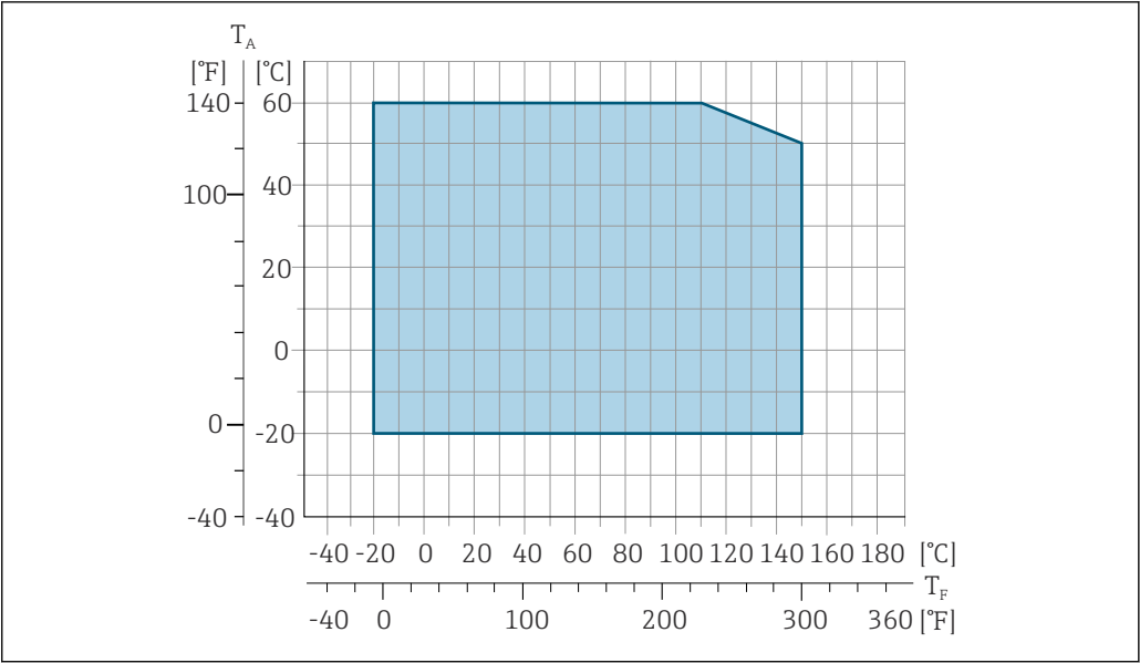
39 Promag 500 (数字)
