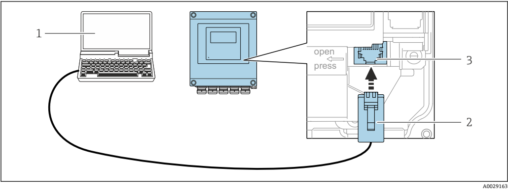
图 29 通过服务接口 (CDI-RJ45) 连接
