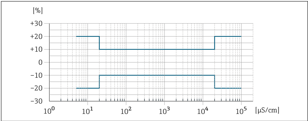
图 37 测量误差 (标准)
