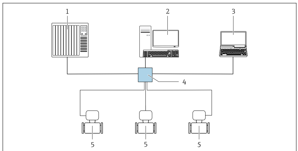
图 28 通过 Modbus TCP + Ethernet 进行远程操作 - 100 Mbit/s: 星形拓扑结构
