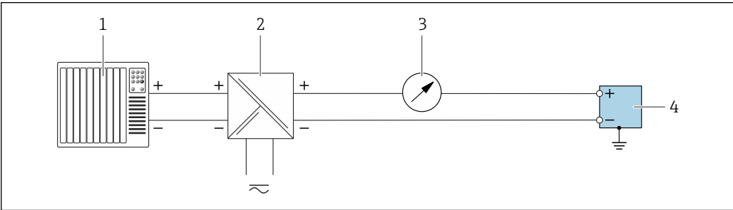
图 16 接线实例：4 ... 20 mA 电流输出（无源）
