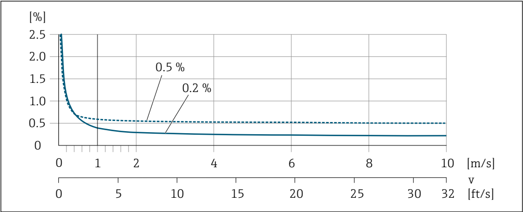
图 36 最大测量误差 (% o.r.)
