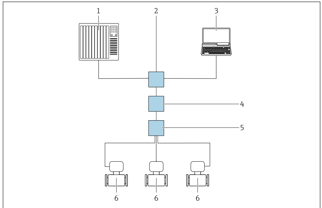
图 27 通过 Modbus TCP + Ethernet-APL 通信进行远程操作（有源信号）
