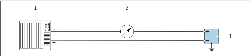
图 15 接线实例：4 ... 20 mA 电流输出（有源）
