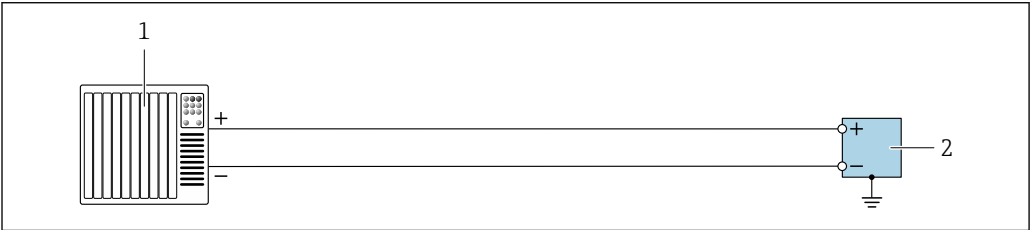
18 接线实例：脉冲输出/频率输出/开关量输出（有源）
