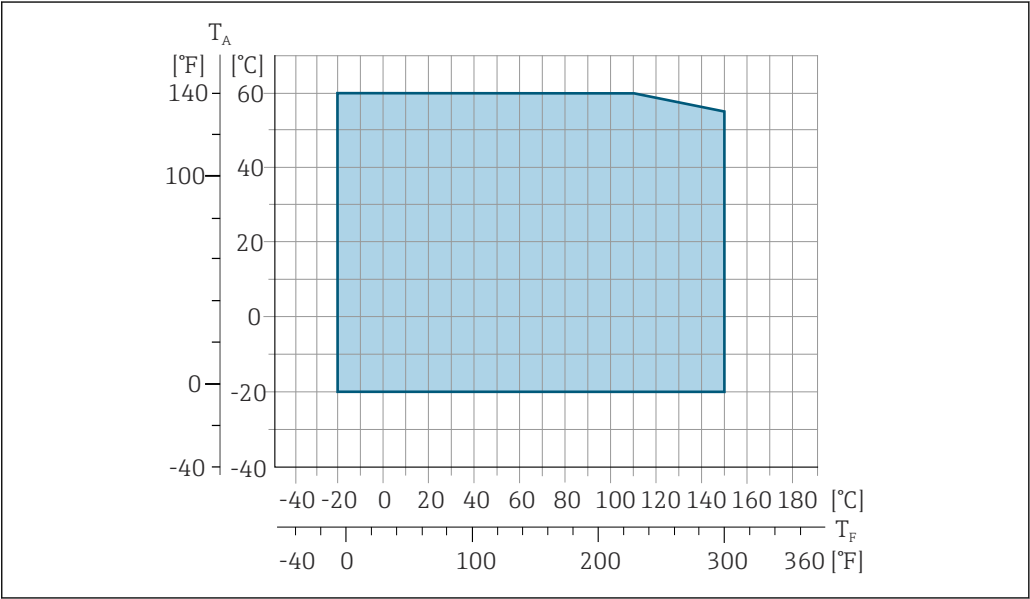
40 Promag 500 (模拟)
