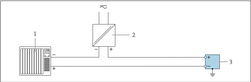
19 接线实例：脉冲输出/频率输出/开关量输出（无源）
