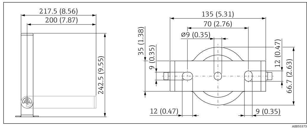
図 30 取付ブラケットの寸法。測定単位 mm (in)
