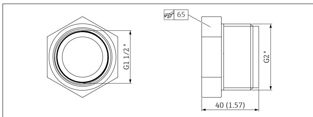
図 27 UNI アダプタの寸法
