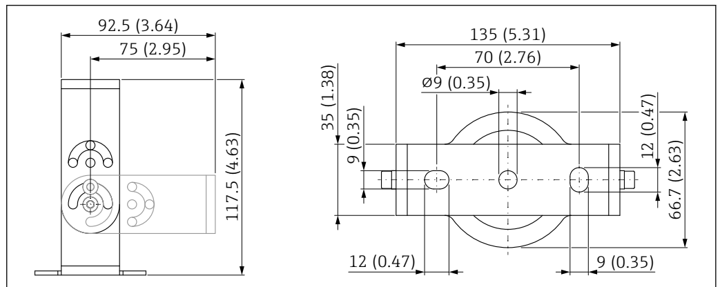
29 取付ブラケットの寸法。測定単位 mm (in)
