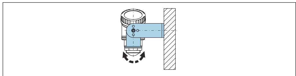
図 15 調整可能な取付ブラケットによる設置
