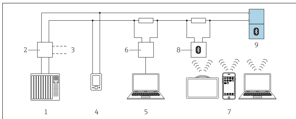
図 23 HART プロトコルを使用したリモート操作オプション
