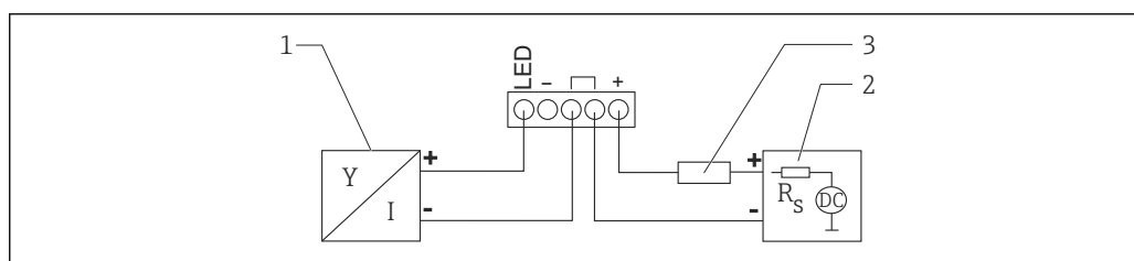
図 6 機能図：HART 機器と RIA15 プロセス表示器の接続（ライトあり）
