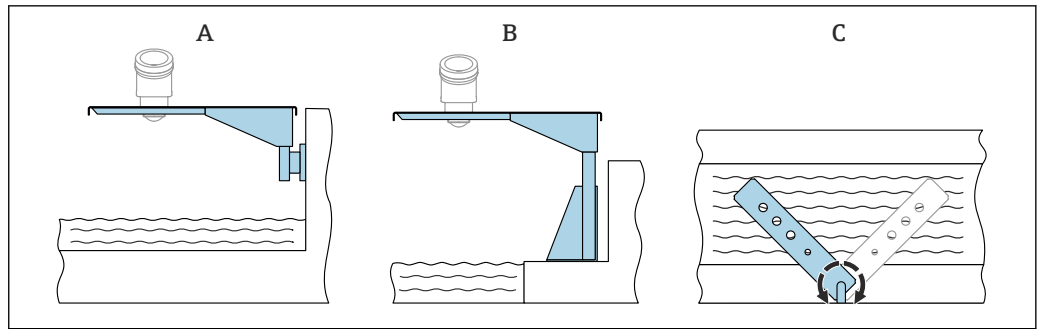
■ 16 回転可能なカンチレバーによる設置
