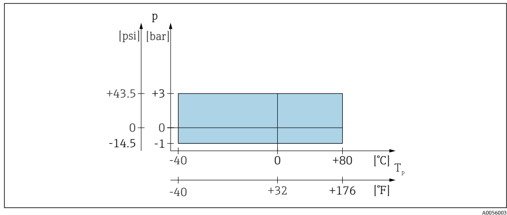
図 17 プロセス温度およびプロセス圧力の許容範囲
