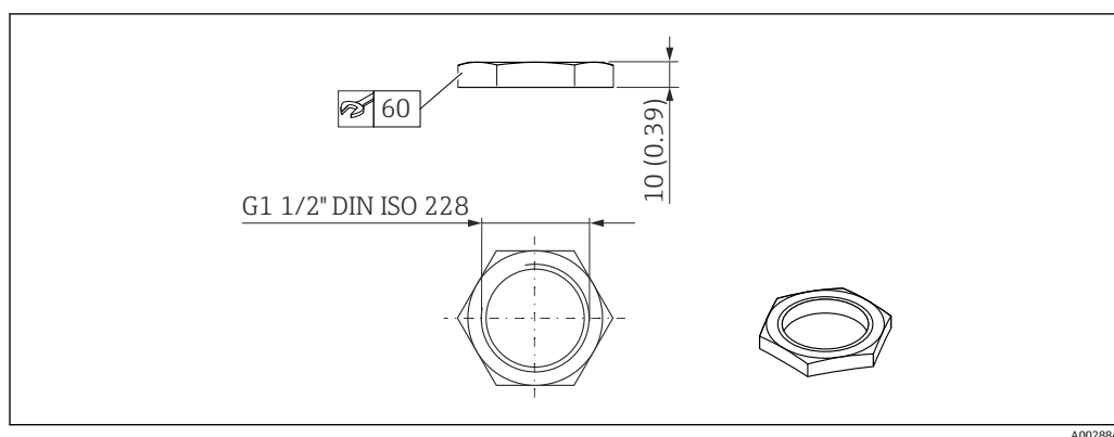
図 25 固定ナットの寸法。測定単位 mm (in)
