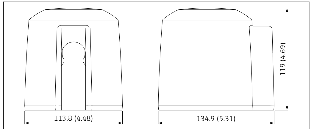
図 24 日除けカバーの寸法。測定単位 mm (in)
