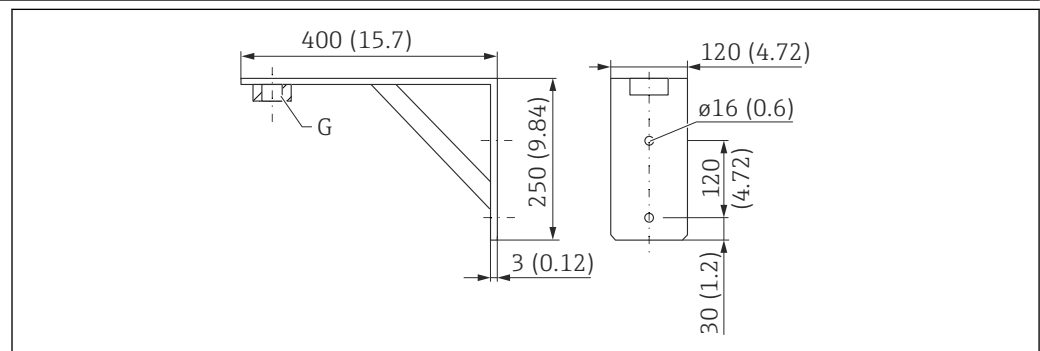
図 31 取付ブラケットの寸法。測定単位 mm (in)
