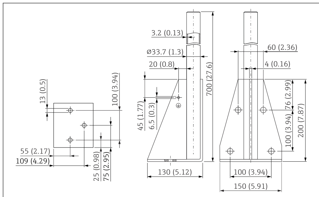
図 35 寸法。測定単位 mm (in)
