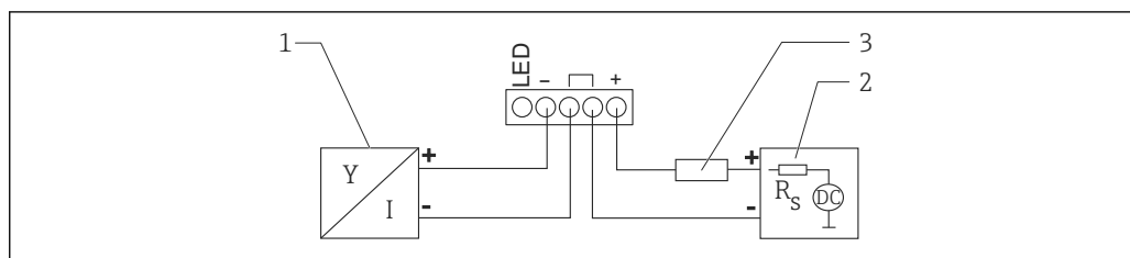
図 5 機能図：HART 機器と RIA15 プロセス表示器の接続（ライトなし）
