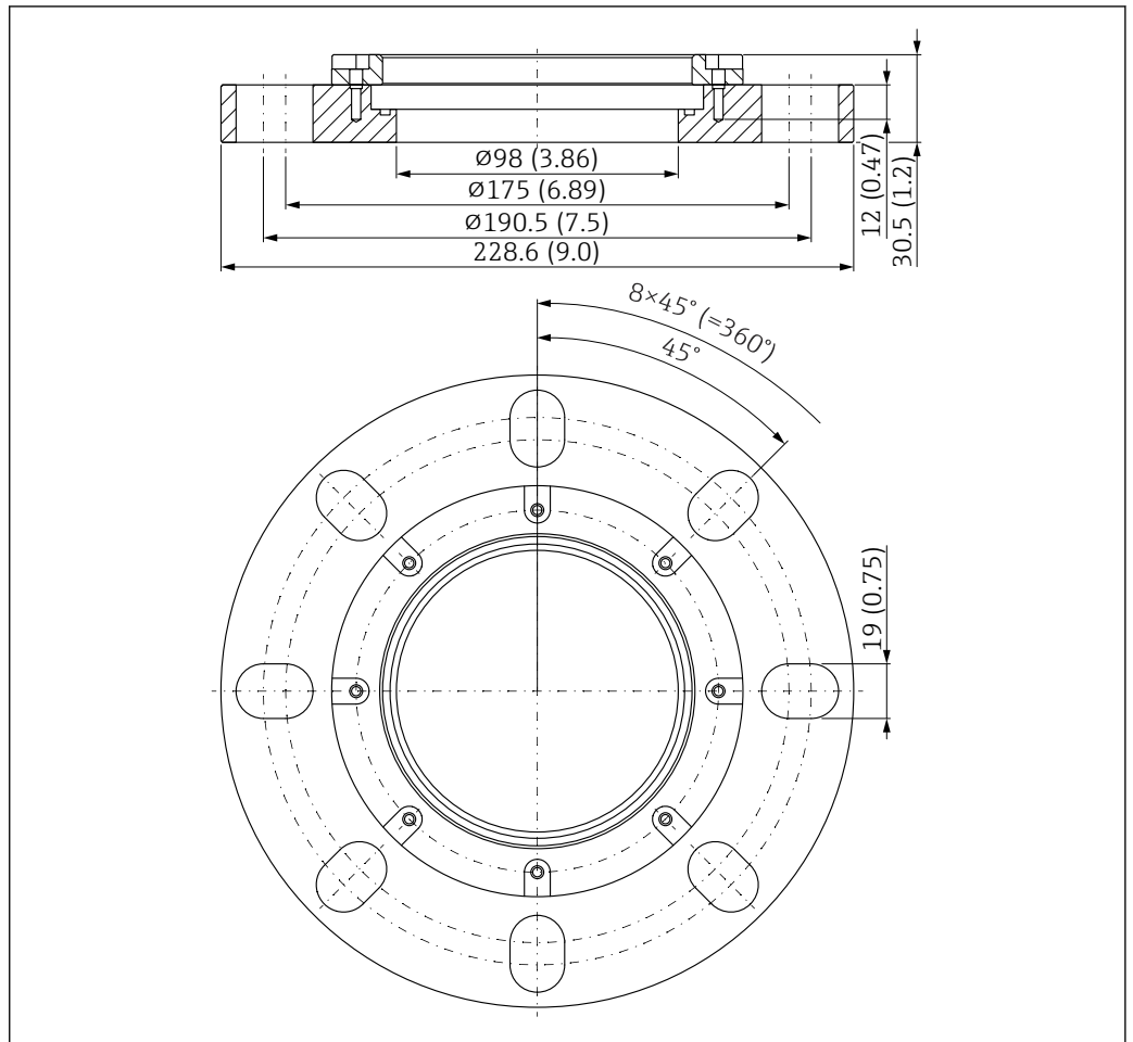
39 UNI スリップオンフランジ 4"/DN100/100 の寸法。測定単位 mm (in)
