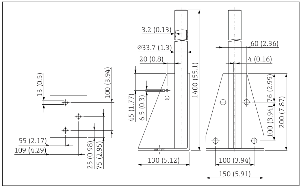
図 36 寸法。測定単位 mm (in)
