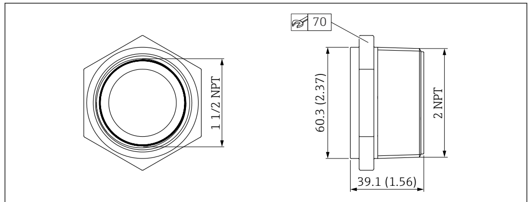
28 UNI アダプタの寸法
