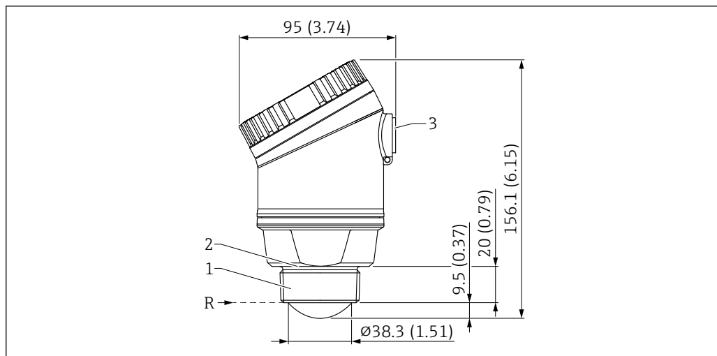
■ 19 寸法：40 mm (1.5 in) アンテナ。測定単位 mm (in)
