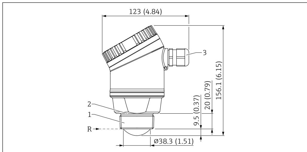
■ 18 寸法：40 mm (1.5 in) アンテナ。測定単位 mm (in)
