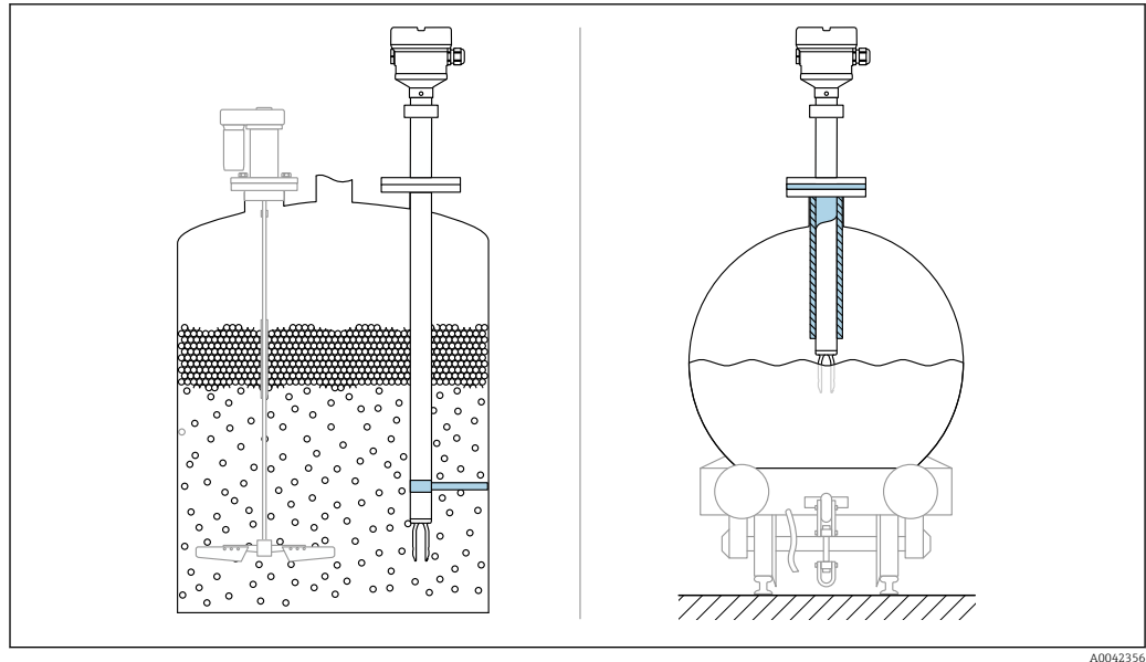
10 Примеры использования опоры при динамической нагрузке
