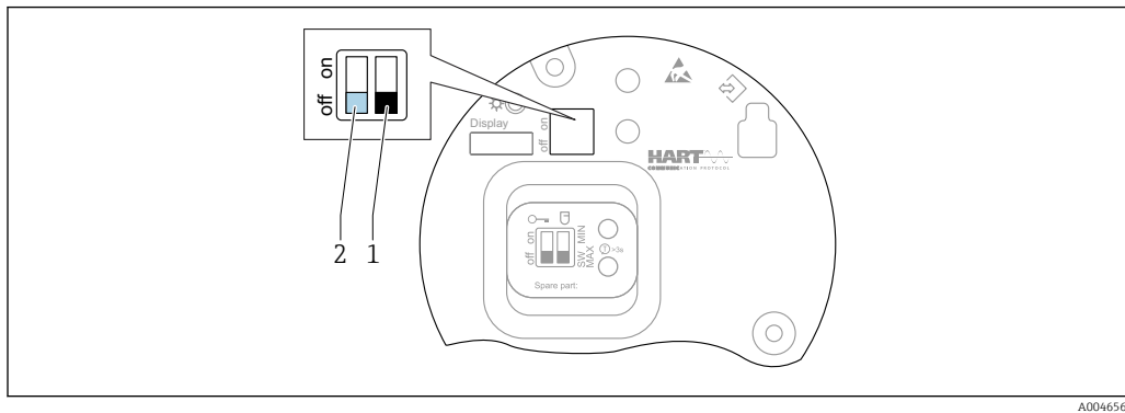
27 Функции DIP-переключателей на электронной вставке FEL60H
