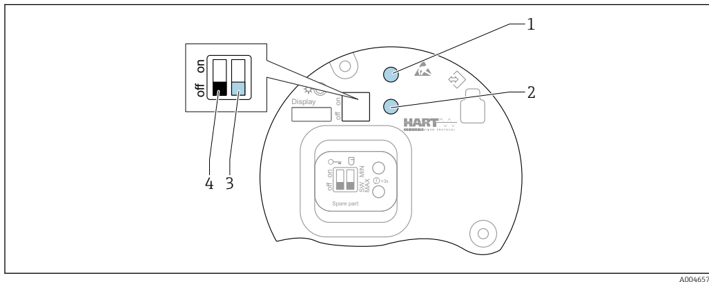
26 Кнопки управления и DIP-переключатель на электронной вставке FEL60H
