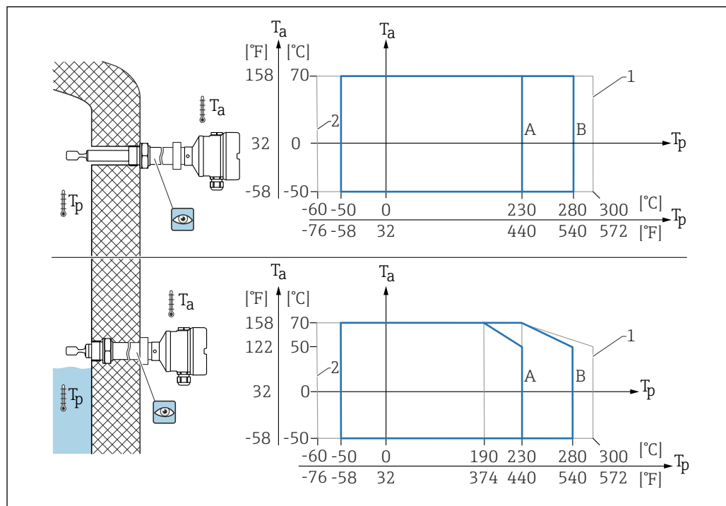
33 Зависимость допустимой температуры окружающей среды T_a в зоне корпуса от рабочей температуры T_p в резервуаре
