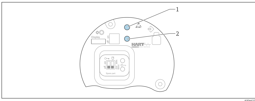
28 Кнопки управления на электронной вставке FEL60H
