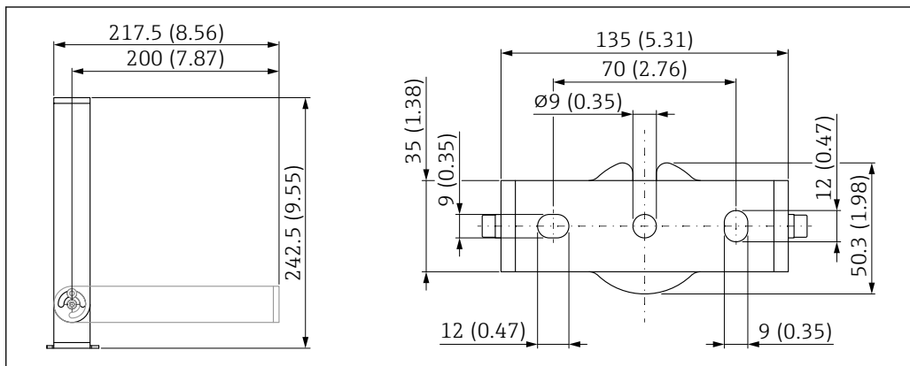
図 36 取付ブラケットの寸法。測定単位 mm (in)
