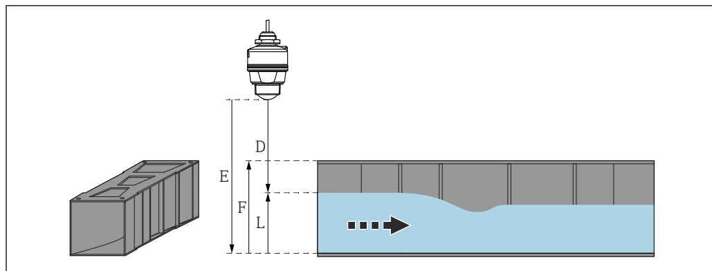
図 23 例：カーファギーベンチュリフリューム
