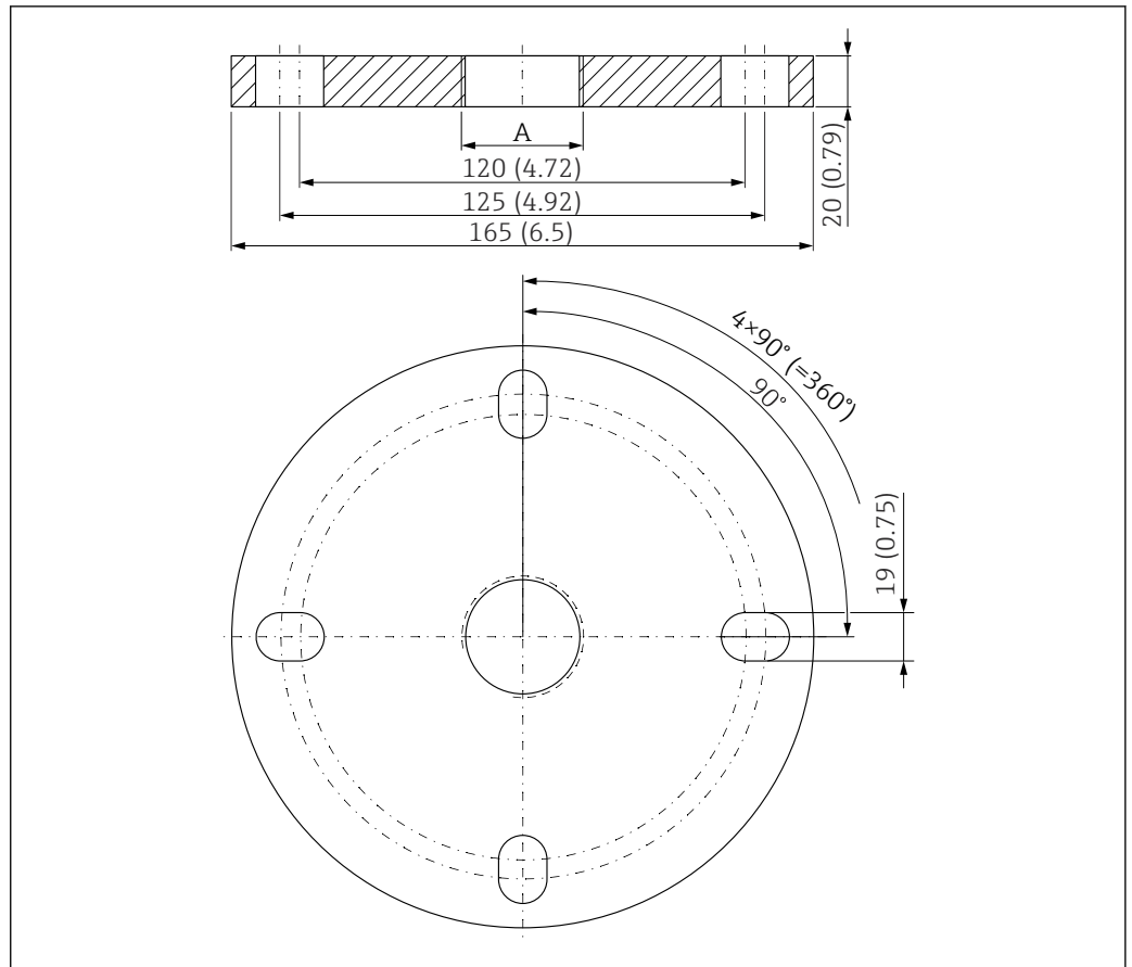
図 53 UNI フランジ 2"/DN50/50 の寸法。測定単位 mm (in)
