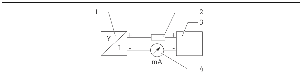
図 11 機能図：HART 接続
