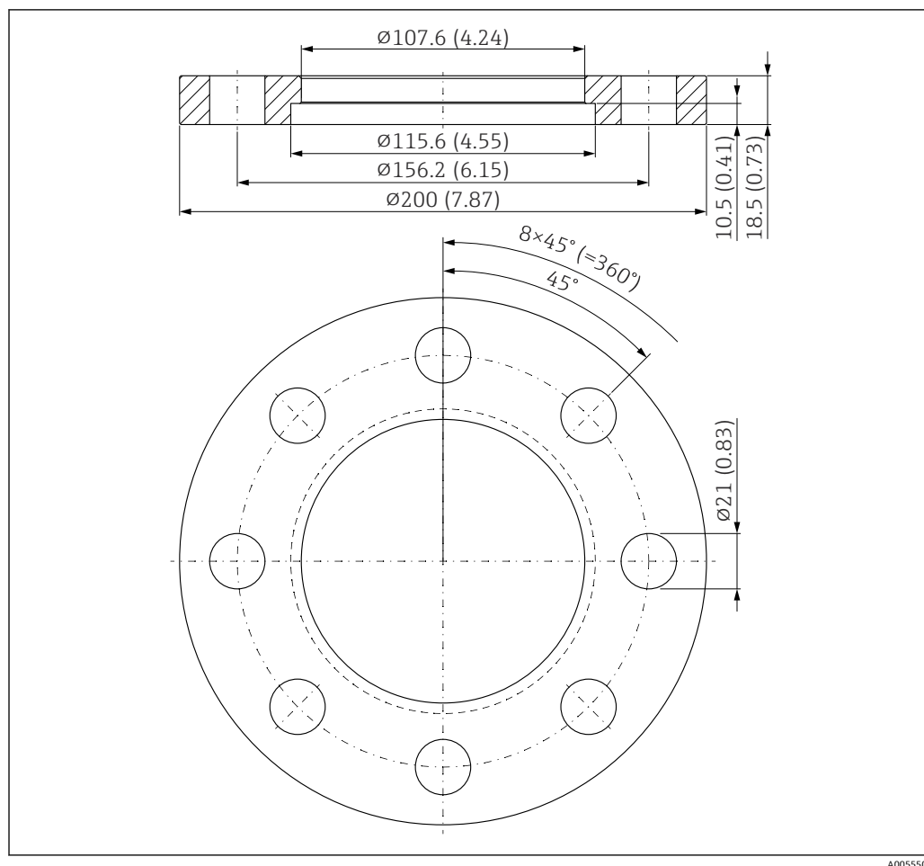
図 50 UNI スリップオンフランジ 3"/DN80/80 の寸法。測定単位 mm (in)
