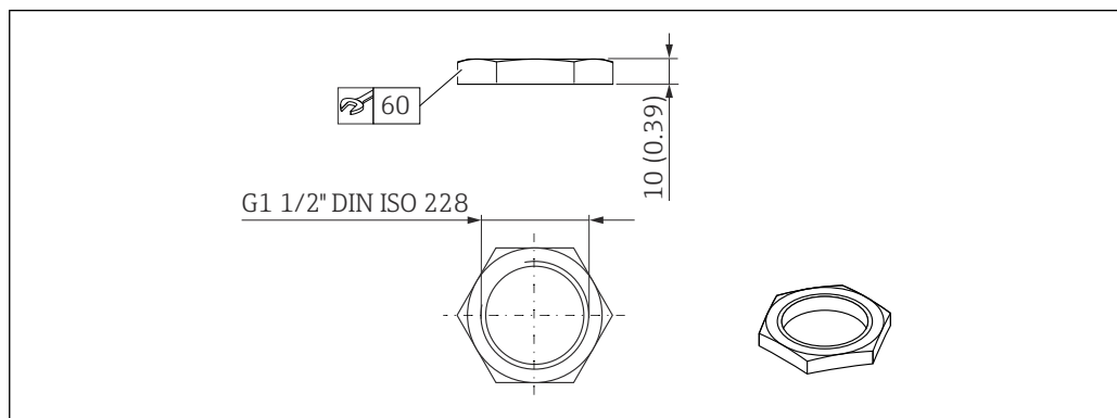
図 28 固定ナットの寸法。測定単位 mm (in)
