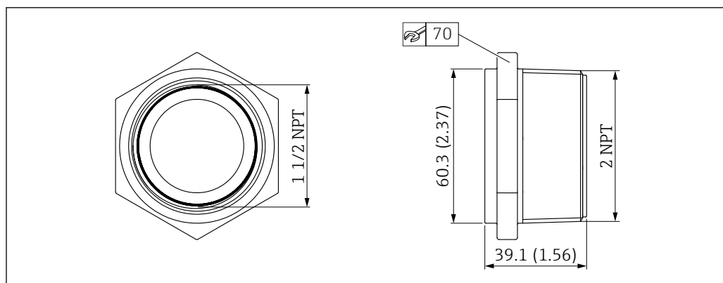
図 31 UNI アダプタの寸法
