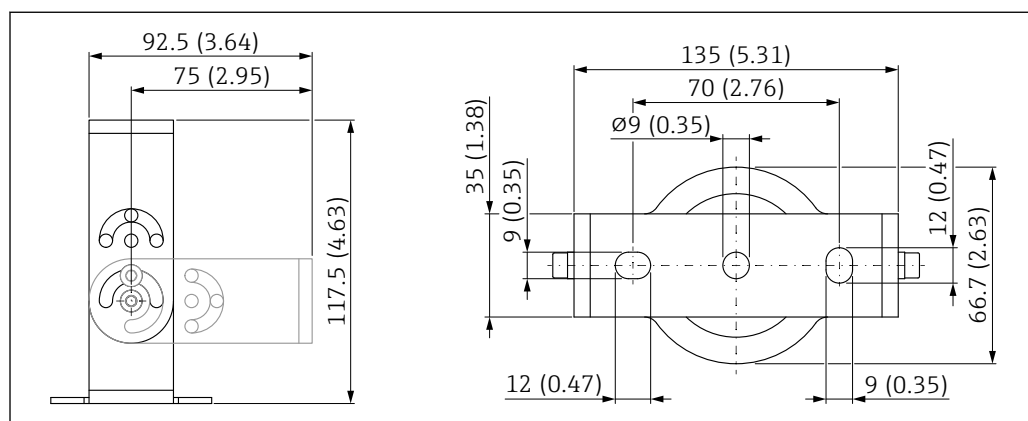
図 35 取付ブラケットの寸法。測定単位 mm (in)
