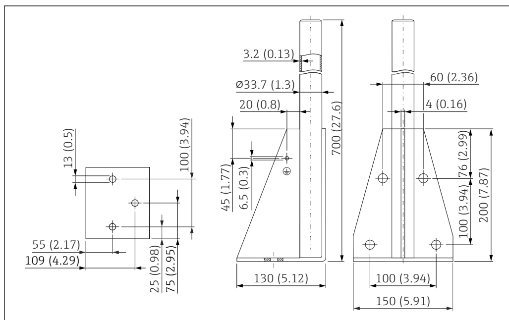
図 45 寸法。測定単位 mm (in)
