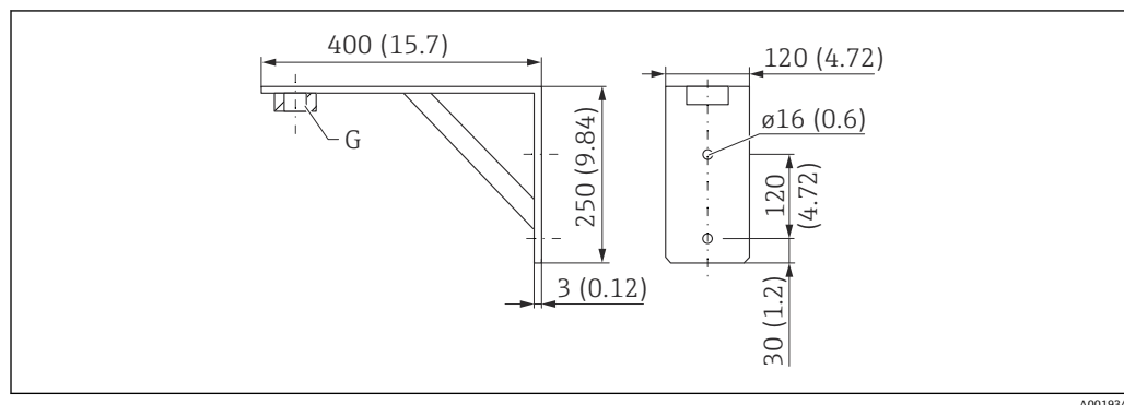
図 38 取付ブラケットの寸法。測定単位 mm (in)
