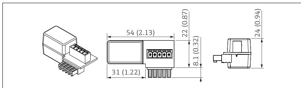
図 58 HART 通信用抵抗器の寸法。測定単位 mm (in)
