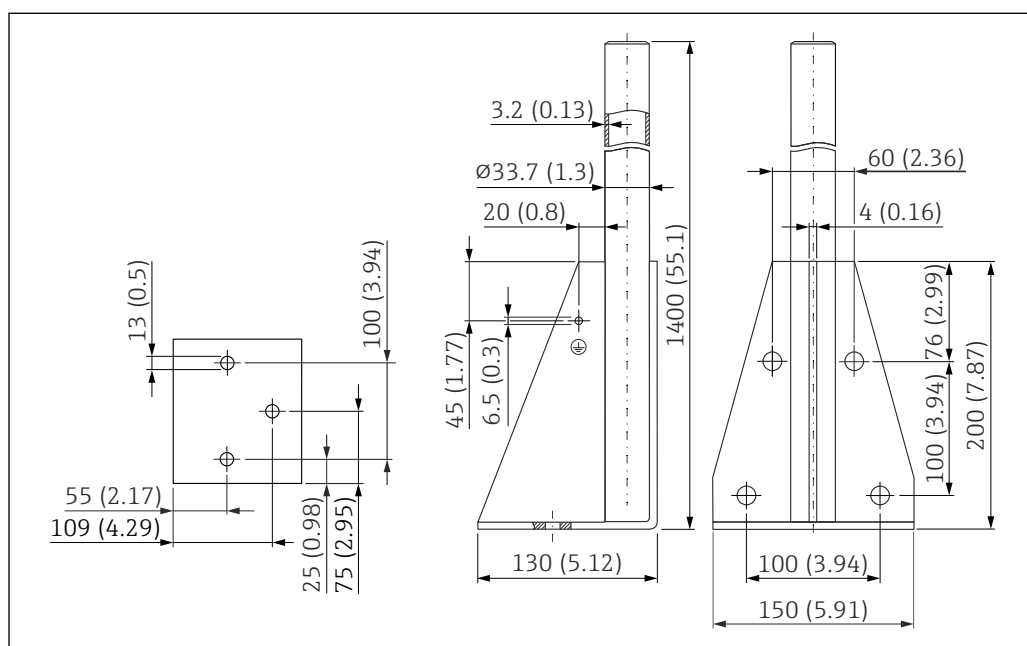
図 46 寸法。測定単位 mm (in)
