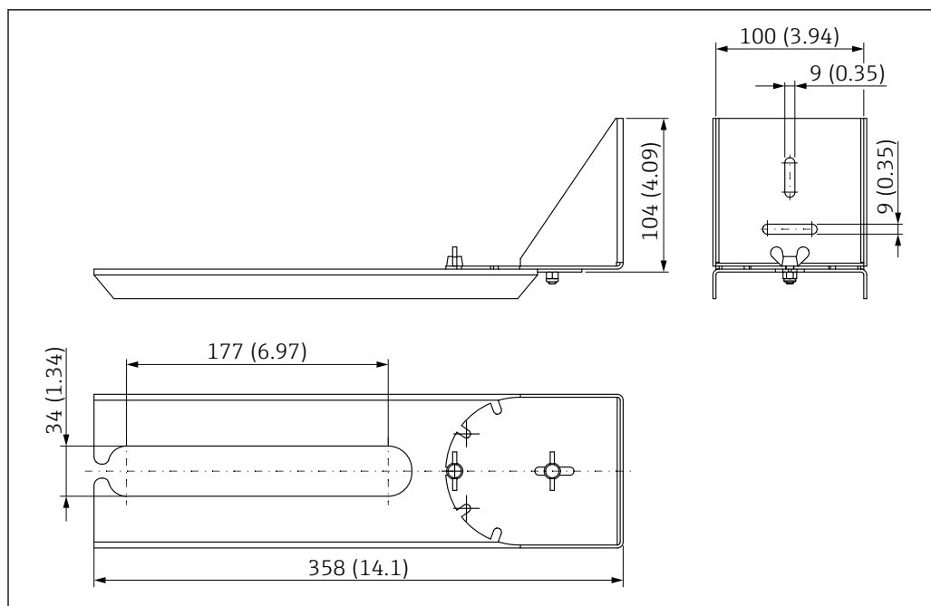
図 48 回転可能な取付ブラケットの寸法。測定単位 mm (in)
