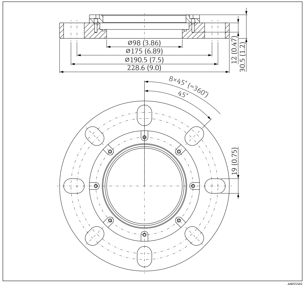
51 UNI スリップオンフランジ 4"/DN100/100 の寸法。測定単位 mm (in)
