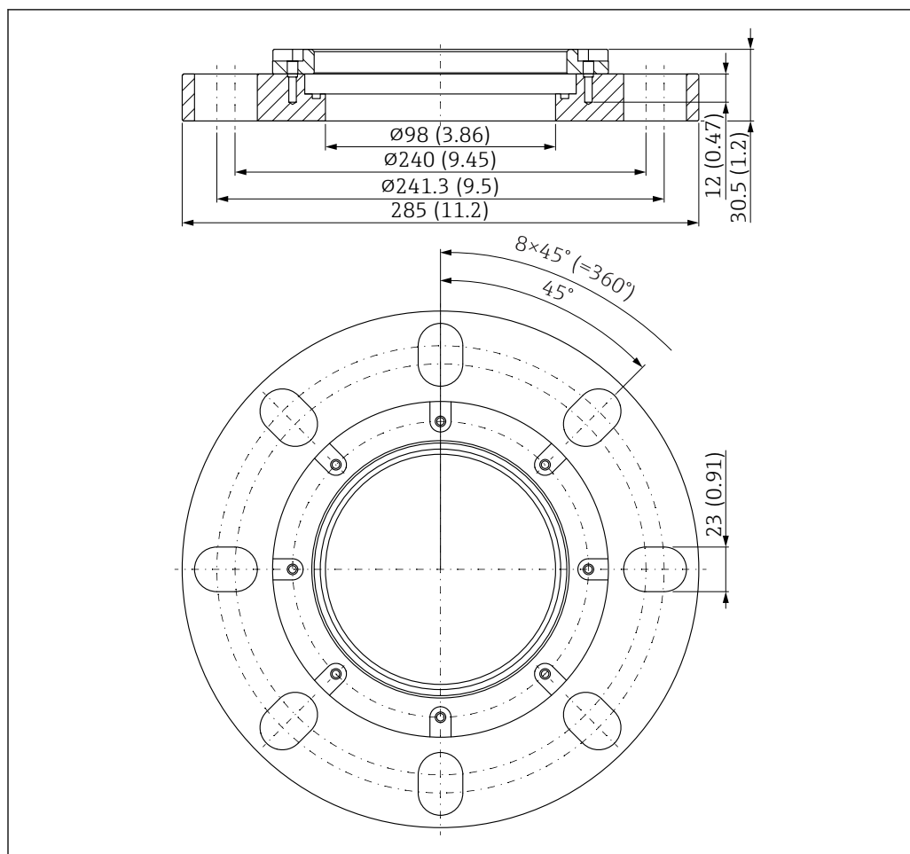
図 52 UNI スリップオンフランジ 6"/DN150/150 の寸法。測定単位 mm (in)
