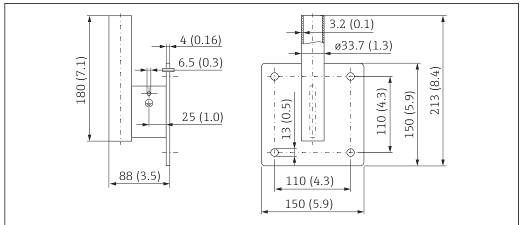
図 47 壁面ブラケットの寸法。測定単位 mm (in)
