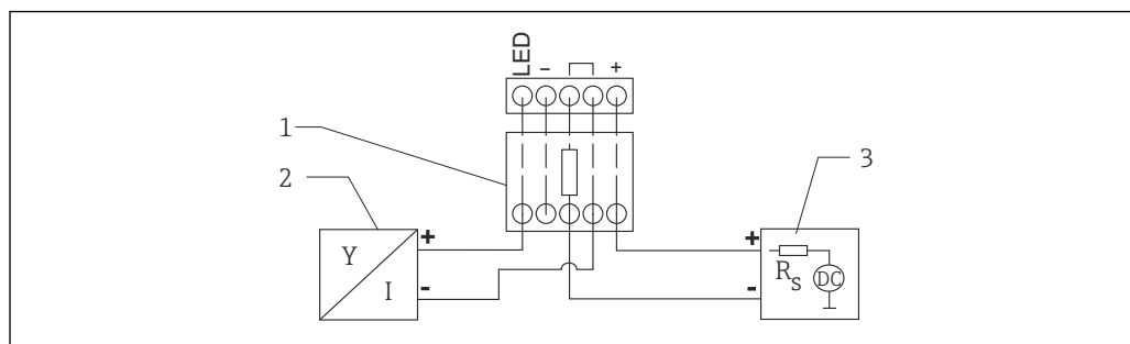
図 15 機能図：HART 機器、RIA15（ライトあり）、HART 通信抵抗モジュールの接続
