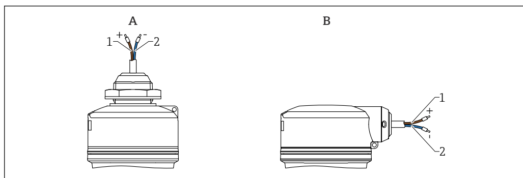
図 10 ケーブルの割当て
