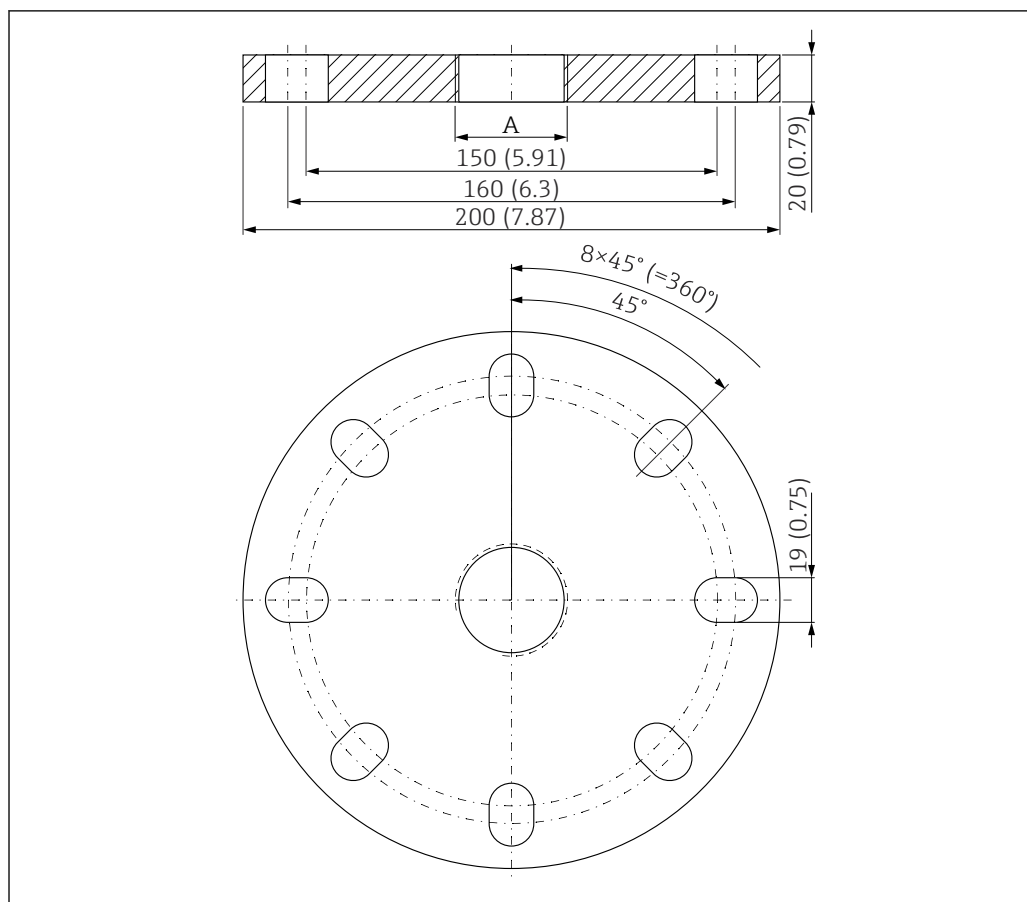
図 54 UNI フランジ 3"/DN80/80 の寸法。測定単位 mm (in)
