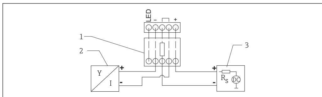
図 14 機能図：HART 機器、RIA15（ライトなし）、HART 通信抵抗モジュールの接続
