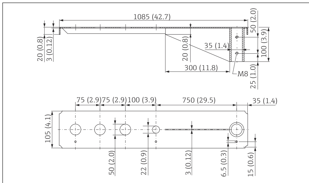
44 回転可能な 1000 mm カンチレバーの寸法：アンテナ終端のプロセス接続 G 1½" の場合。測定単位 mm (in)
