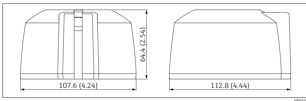
図 26 保護カバー G1/NPT1 の寸法、上部に電線口。測定単位 mm (in)
