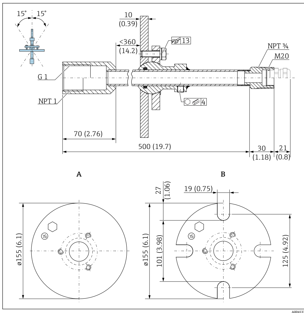
49 寸法。測定単位 mm (in)
