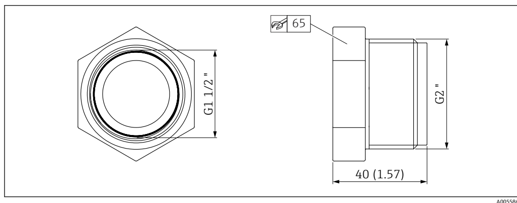
図 30 UNI アダプタの寸法
