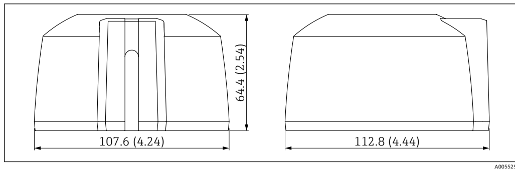
図 27 保護カバーの寸法、側面に電線口。測定単位 mm (in)
