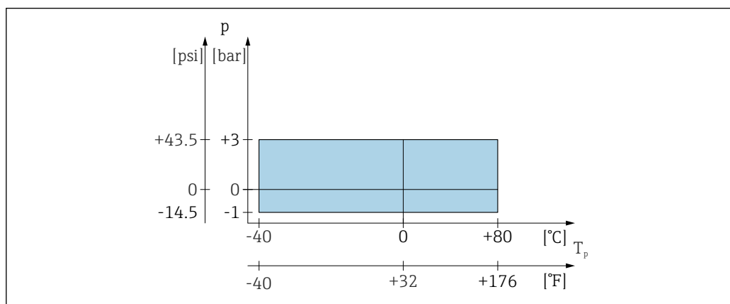
図 59 プロセス温度およびプロセス圧力の許容範囲
