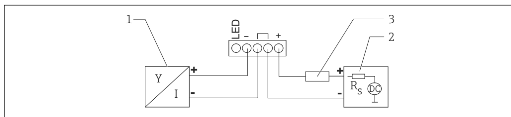
図 12 機能図：HART 機器と RIA15 プロセス表示器の接続（ライトなし）
