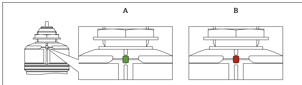
図 16 機器の LED インジケータ
