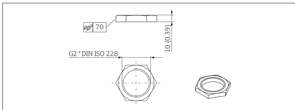
図 29 固定ナットの寸法。測定単位 mm (in)
