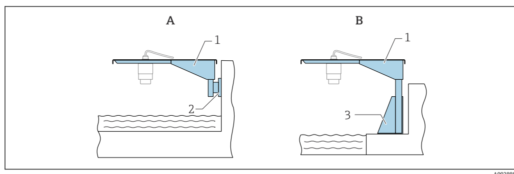
図 39 センサ設置タイプ：電線口がプロセス接続
