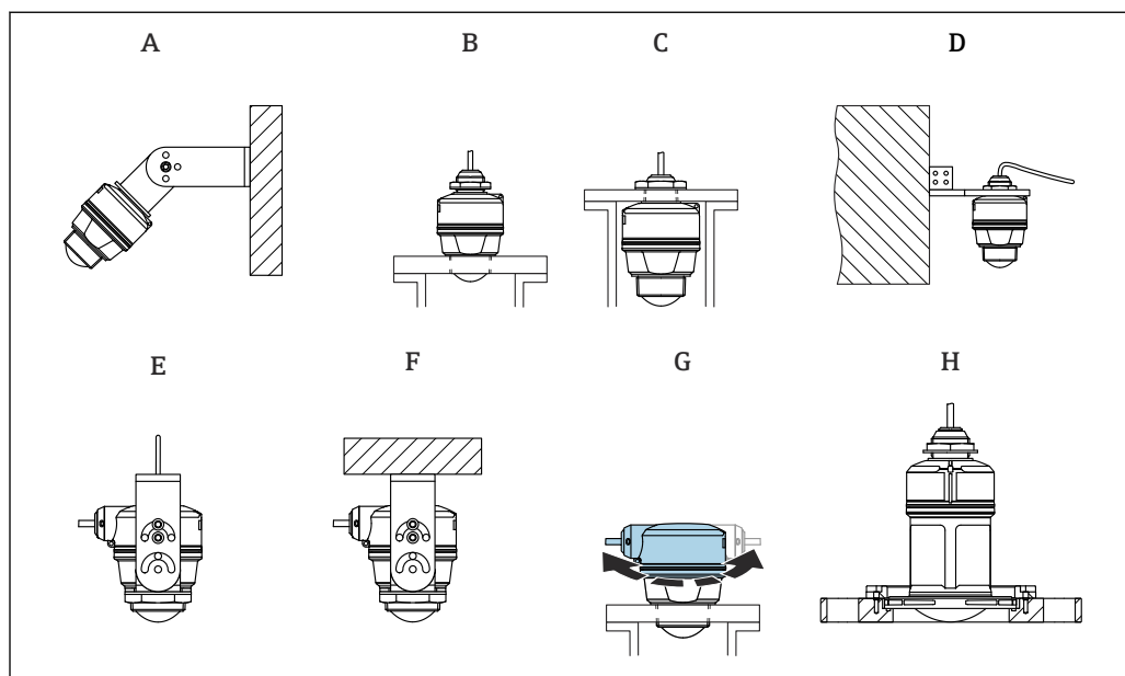
図 2 壁面または天井取付け
