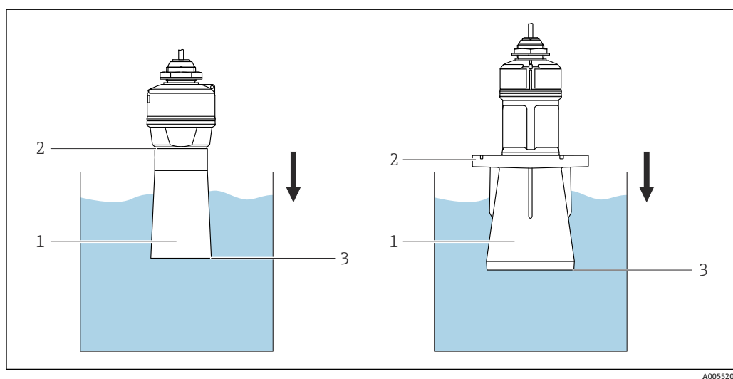
図 5 溢れ防止チューブの機能
