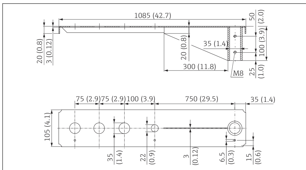
41 回転可能な 1000 mm カンチレバーの寸法：電線口がプロセス接続の場合。測定単位 mm (in)
