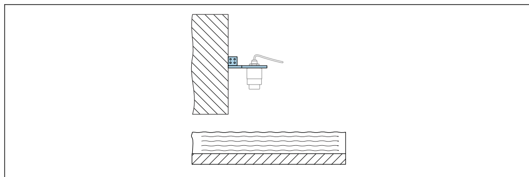
図 9 回転および調整可能なカンチレバーと壁面取付ブラケット（例：フレュームの中央に機器を位置合わせするため）
