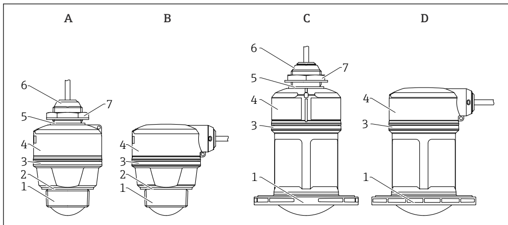
図 1 機器構成
