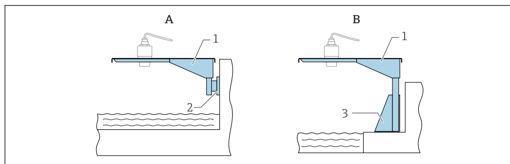
図 42 センサ設置タイプ：アンテナ終端のプロセス接続
