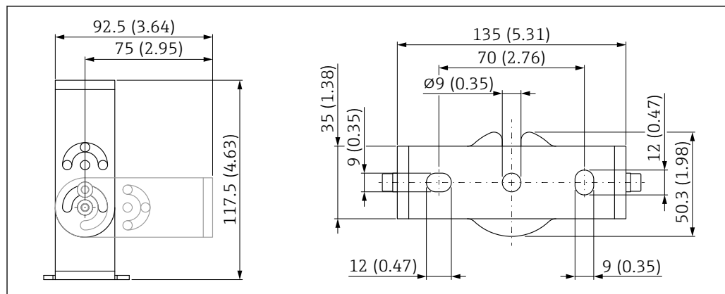
図 34 取付ブラケットの寸法。測定単位 mm (in)
