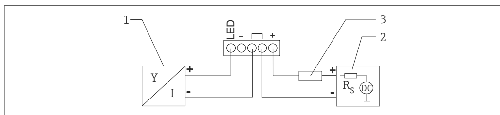
図 13 機能図：HART 機器と RIA15 プロセス表示器の接続（ライトあり）
