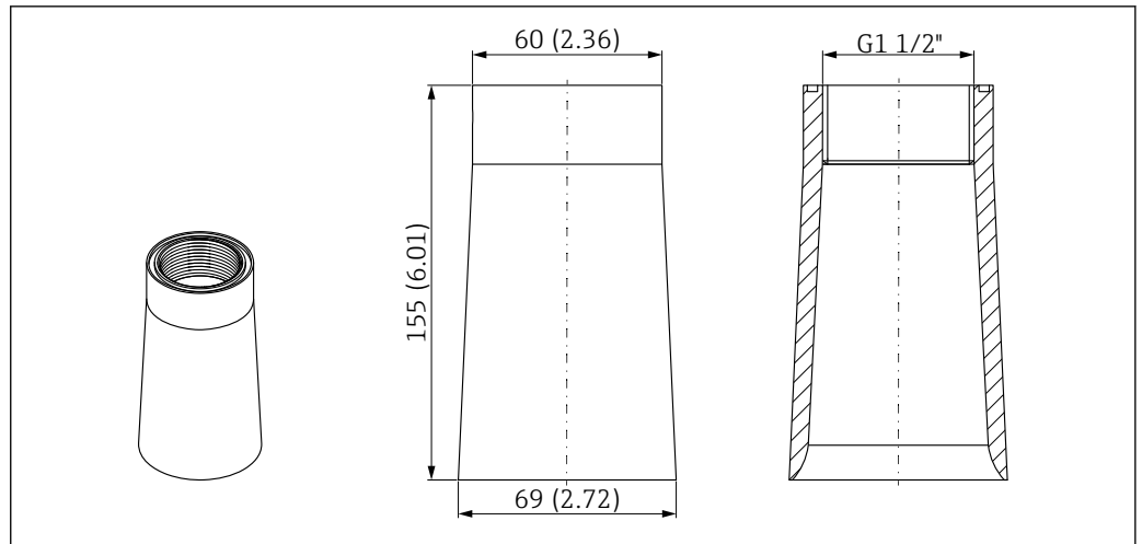
図 32 溢れ防止チューブ 40 mm (1.5 in) の寸法。測定単位 mm (in)
