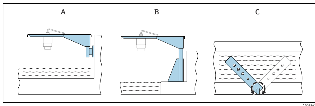
図 8 回転可能なカンチレバーによる設置
