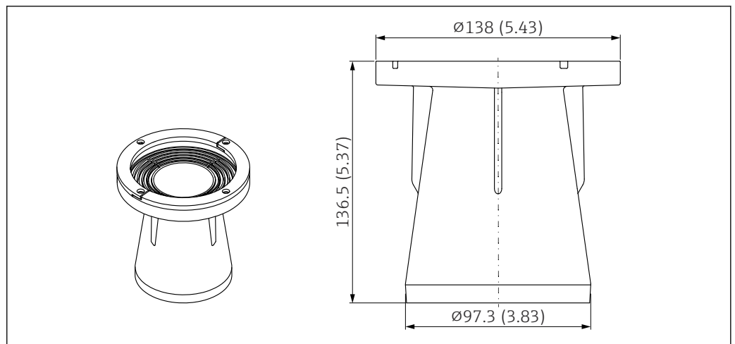
図 33 溢れ防止チューブ 80 mm (3 in) の寸法。測定単位 mm (in)
