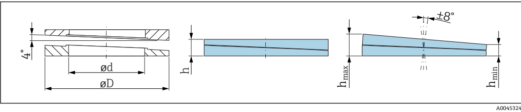
56 寸法
