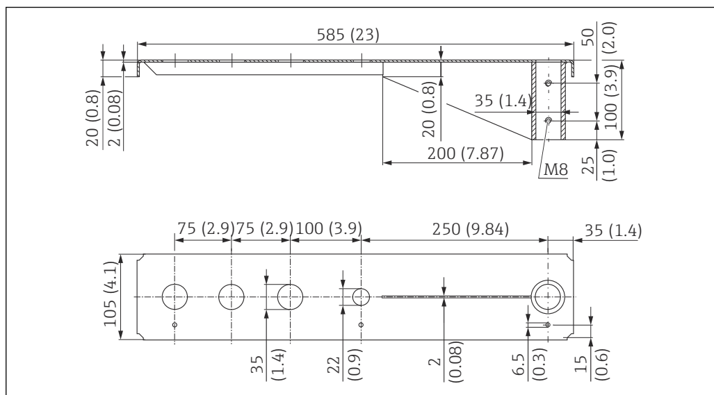
40 回転可能な 500 mm カンチレバーの寸法：電線口がプロセス接続の場合。測定単位 mm (in)
