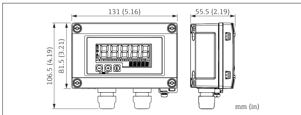
図 57 フィールドハウジング付き RIA15 の寸法。測定単位 mm (in)
