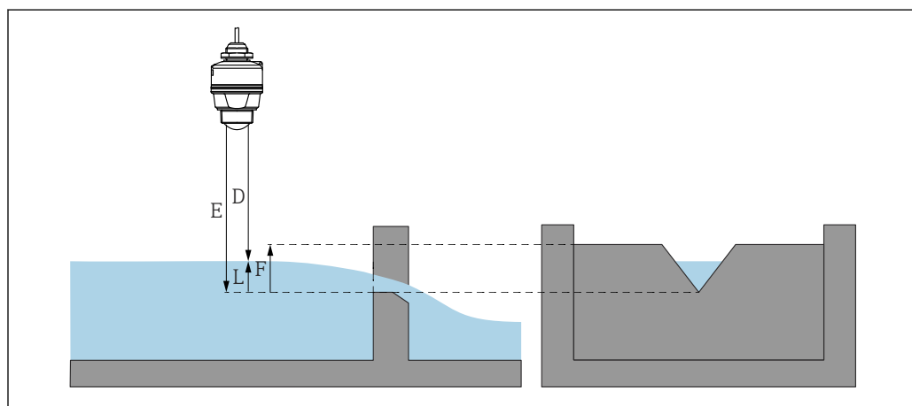
図 24 例：三角堰
