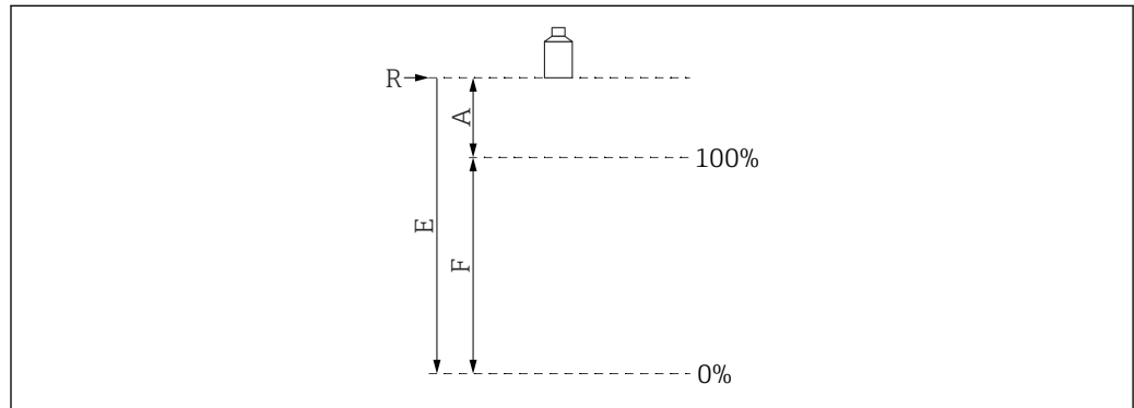
10 Variabili per definire il campo
