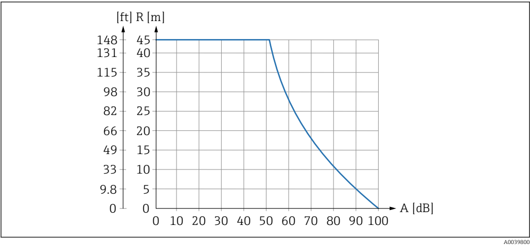
2 Grafico del campo per sensori a ultrasuoni
