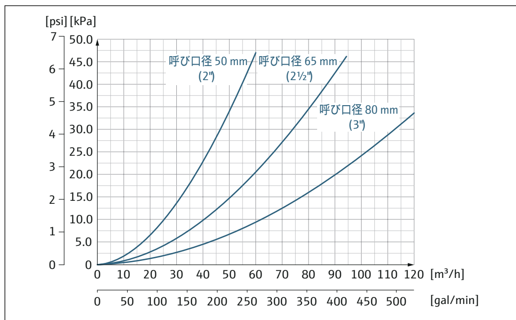
図 29 呼び口径 50~80 mm (2~3") の圧力損失: 「設計」のオーダーコード、オプション C 「固定フランジ、狭径計測チューブ、0 x 呼び口径 上流側/下流側直管長」の場合
