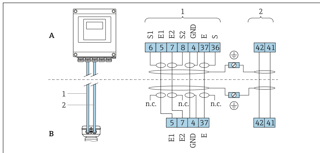
図 2 分離型の端子の割当て
