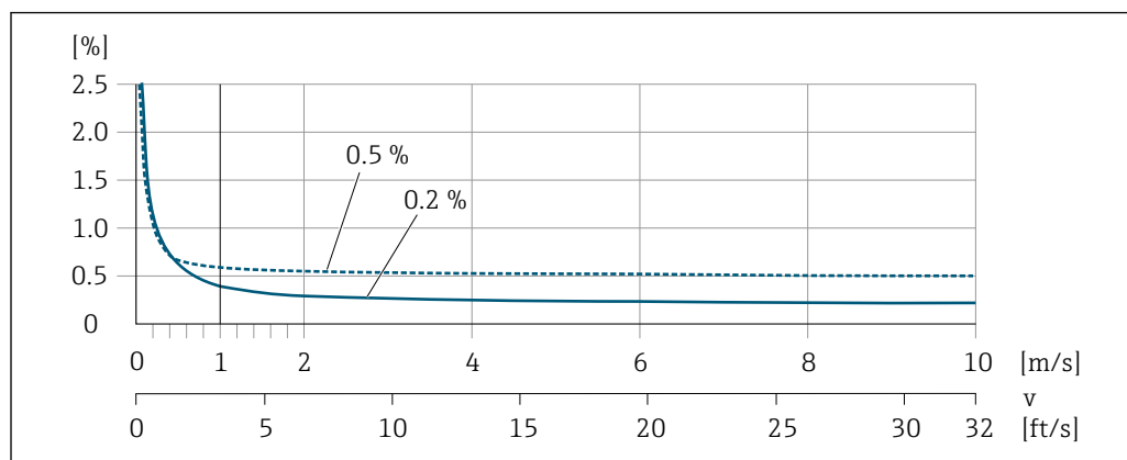
図 14 最大測定誤差 (%) o.r.
