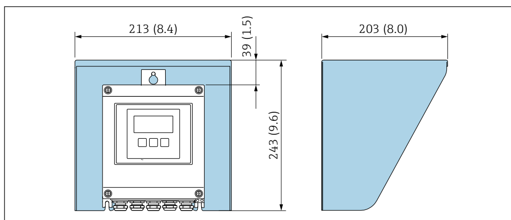
図 31 日除けカバー、寸法 : mm (in)
