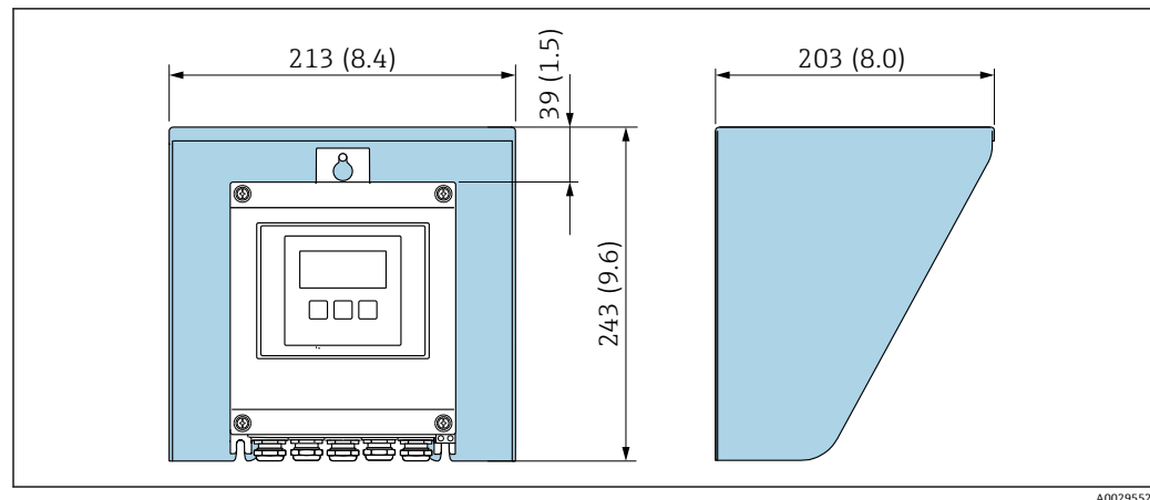
図 18 日除けカバー、寸法：mm (in)
