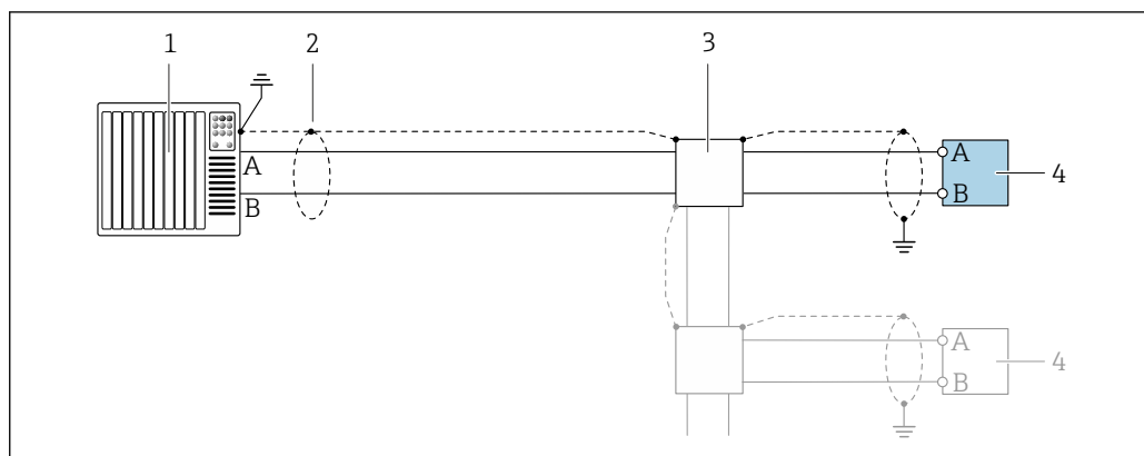
図 10 Modbus RS485（非危険場所およびゾーン 2/Div. 2 用）の接続例
