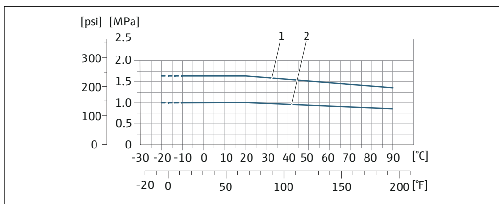
図 28 プロセス接続材質: ステンレス (-20 °C (-4 °F)); 炭素鋼 (-10 °C (14 °F))
