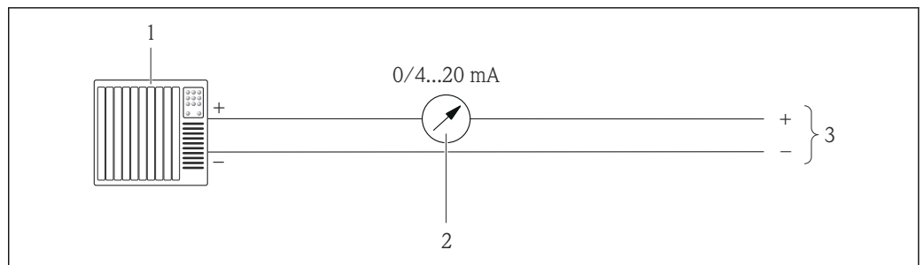
図 6 電流出力 0~20 mA（アクティブ）および 4~20 mA（アクティブ）の接続例
