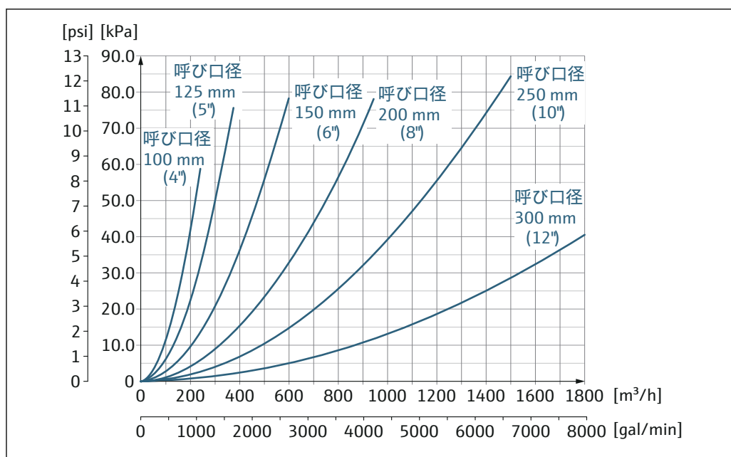
図 30 呼び口径 100～300 mm (4～12") の圧力損失：「設計」のオーダーコード、オプション C「固定フランジ、狭窄計測チューブ、0 x 呼び口径 上流側/下流側直管長」の場合
