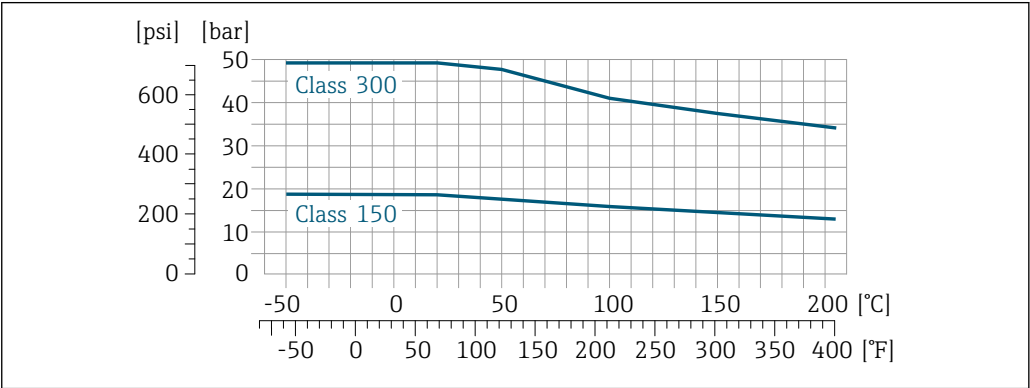
18 Com material do flange: 1.4539 (904L); flanges soltos (não úmidos) 1.4404 (316/316L)
