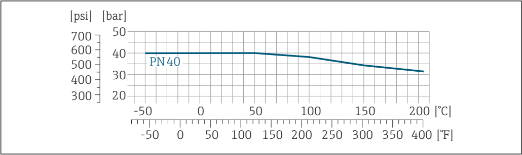
17 Com material do flange: 1.4539 (904L), Liga C22; flanges soltos (não úmidos) 1.4404 (316/316L)
