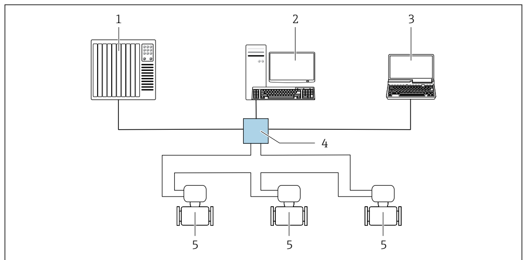
42 Opções para operação remota através da rede EtherNet/IP: topologia de anel
