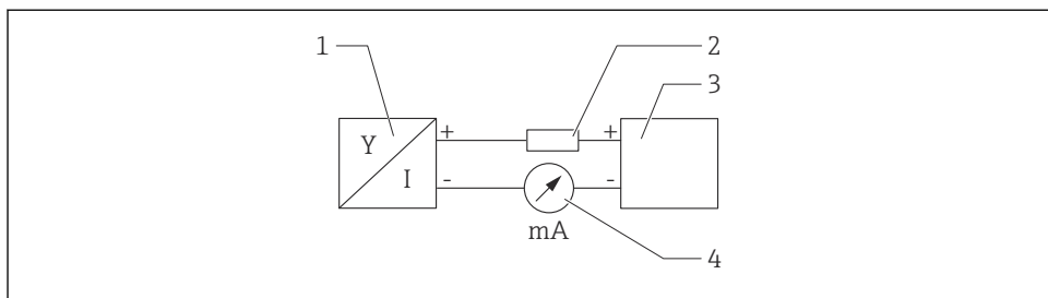
4 Blokovna shema vezave HART
