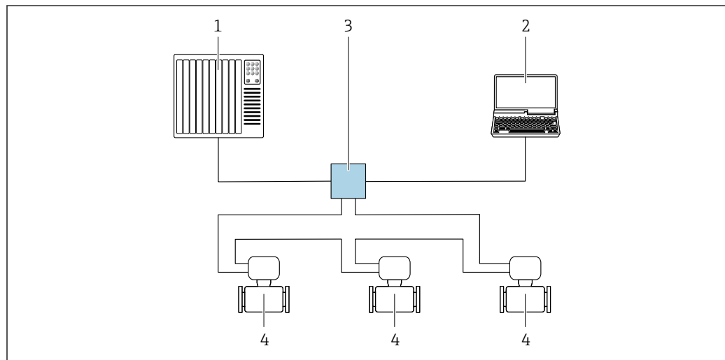
44 Möglichkeiten der Fernbedienung via PROFINET-Netzwerk: Ringtopologie
