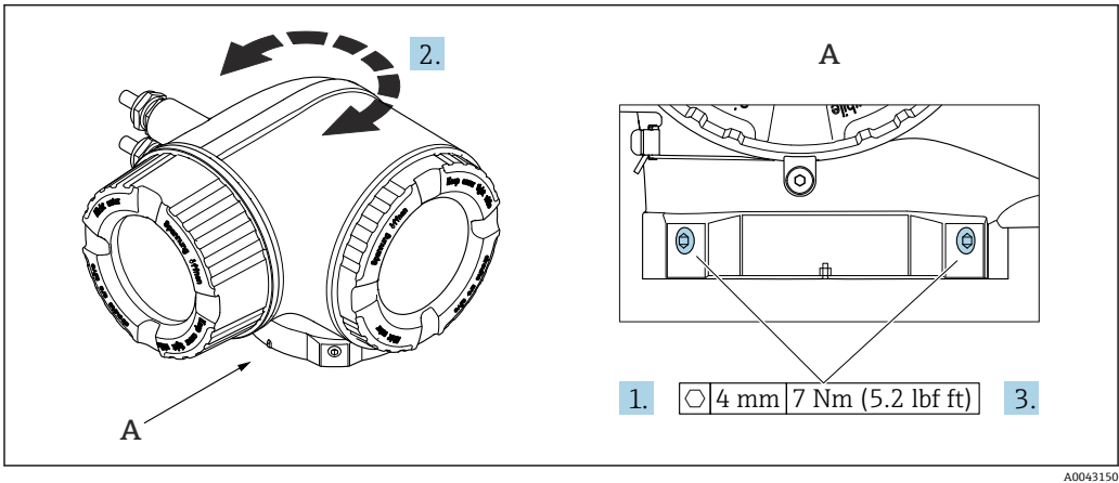
图 6 防爆型外壳
