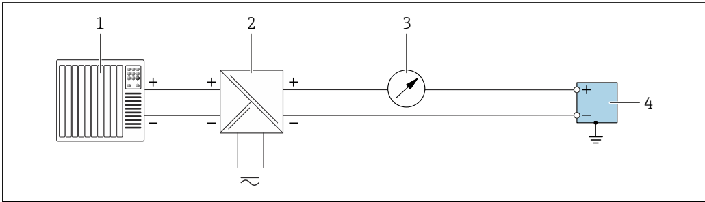
9 接线实例：4 ... 20 mA 电流输出（无源）
