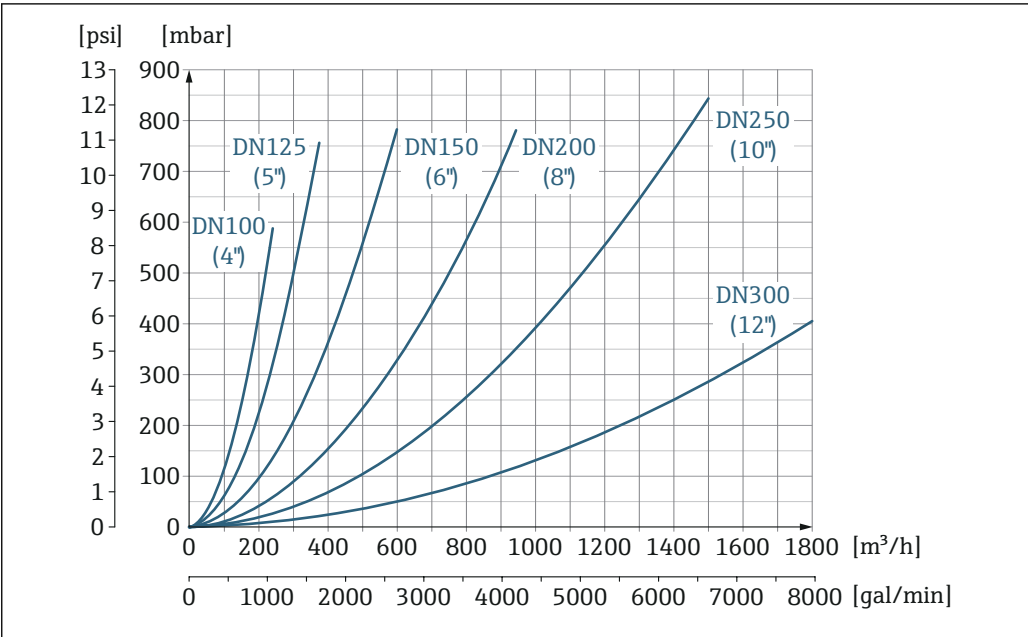
33 压损: 适用口径 DN 100...300 (4...12"); 订购选项“设计”, 选型代号 C “固定法兰, 缩径测量管, 无前后直管段长度要求”
