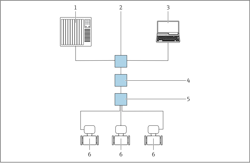
图 20 通过 Modbus TCP + Ethernet-APL 通信进行远程操作（有源信号）
