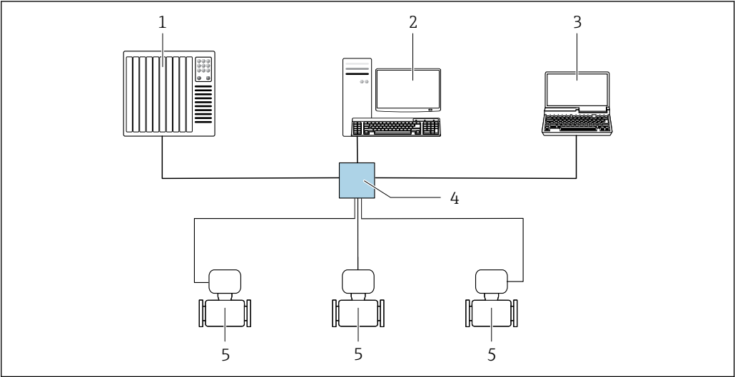
图 21 通过 Modbus TCP + Ethernet 进行远程操作 - 100 Mbit/s: 星形拓扑结构
