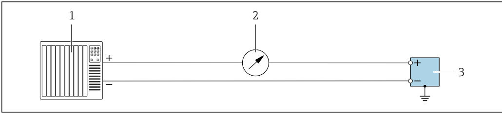
8 接线实例：4 ... 20 mA 电流输出（有源）
