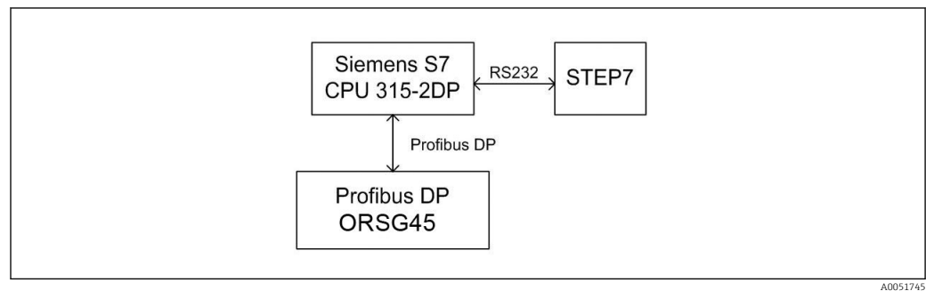
19 Netzwerkübersicht (auch für Nachfolger Siemens S7 CPU 315-2 PN/DP)
