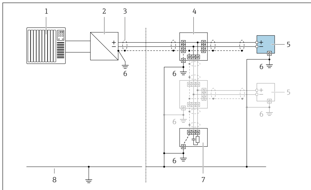
16 Esempio di collegamento per PROFIBUS PA
