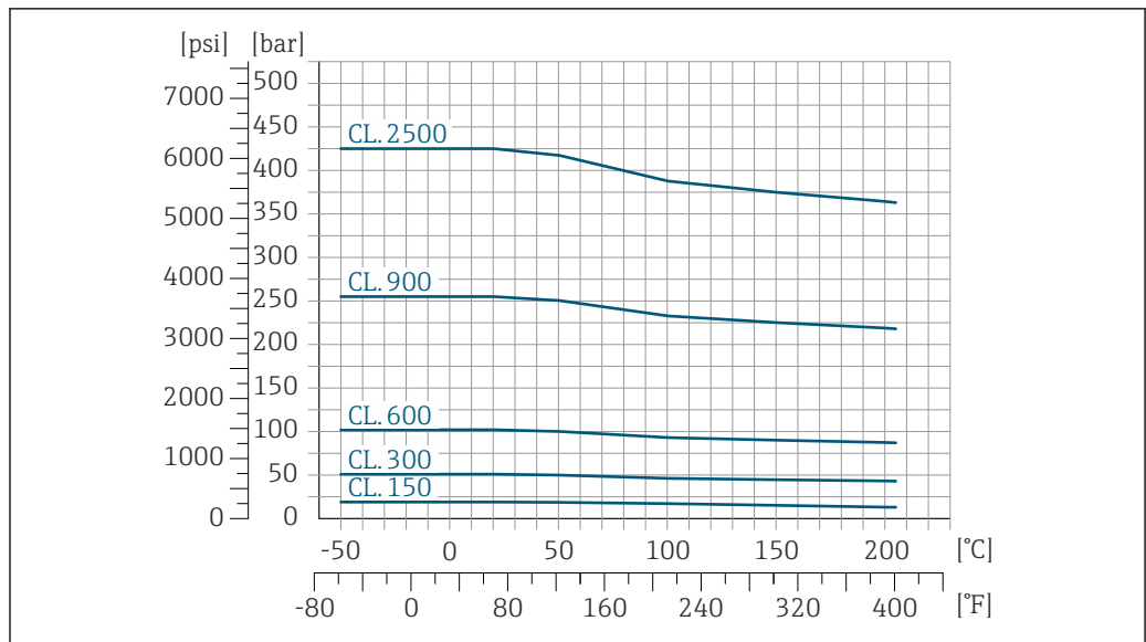
24 Avec matériau de bride 1.4404 (316/316L)
