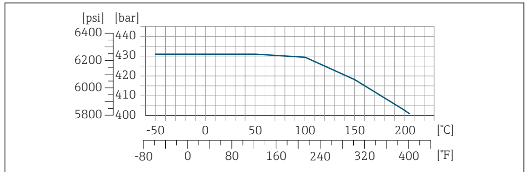
31 Avec matériau de bride : Alloy C22, 2.4602 (UNS N06022) ; caractéristique de commande "Mat. tube mesure, surface en contact", option HB
