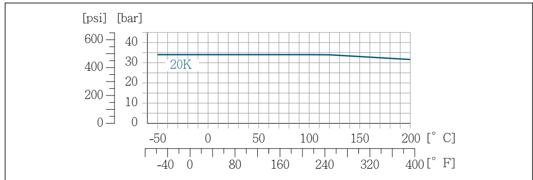
28 Bride tournante avec matériau de bride : 1.4301 (F304), parties en contact avec le produit Alloy C22: 2.4602 (UNS N06022)
