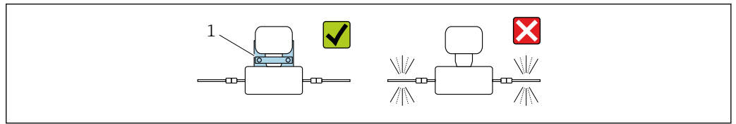
1 Support de capteur (Caractéristique de commande "Accessoires fournis", option PR)
