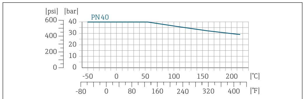
23 Bride tournante avec matériau de bride : 1.4301 (F304), parties en contact avec le produit Alloy C22 : 2.4602 (UNS N06022)
