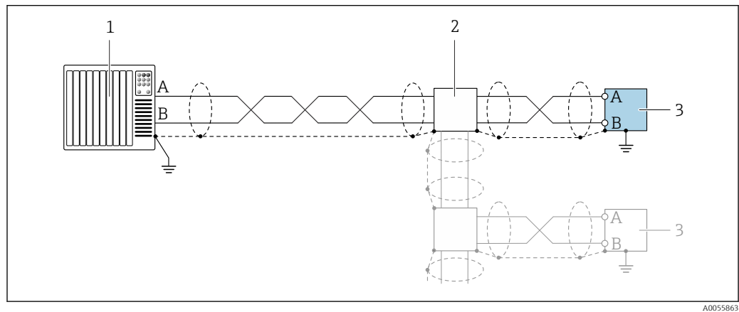
20 Ejemplo de conexión para Modbus RS485
