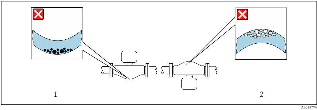
5 Orientación del sensor con tubo de medición curvado 1 Evite esta orientación para productos con sólidos en suspensión: Riesgo de acumulación de sólidos 2 Evite esta orientación para productos que contengan gas: Riesgo de acumulación de gas
