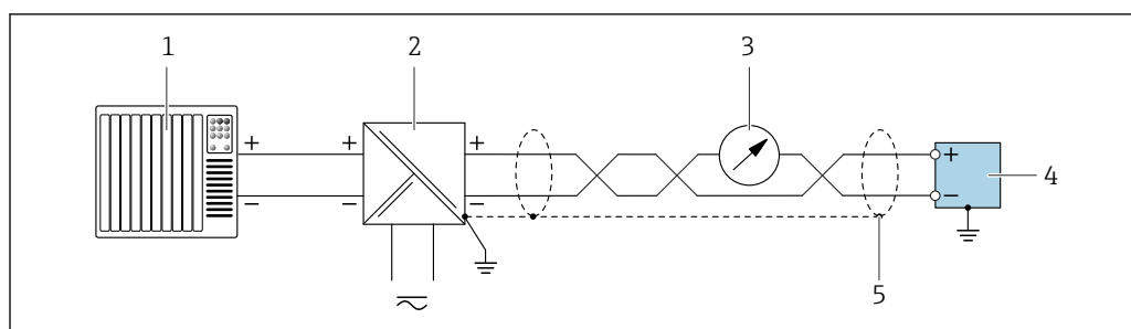
图 9 接线实例: 4 ... 20 mA HART 电流输出 (无源)
