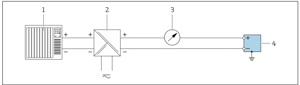
图 6 接线实例: 4 ... 20 mA 电流输出 (无源)
