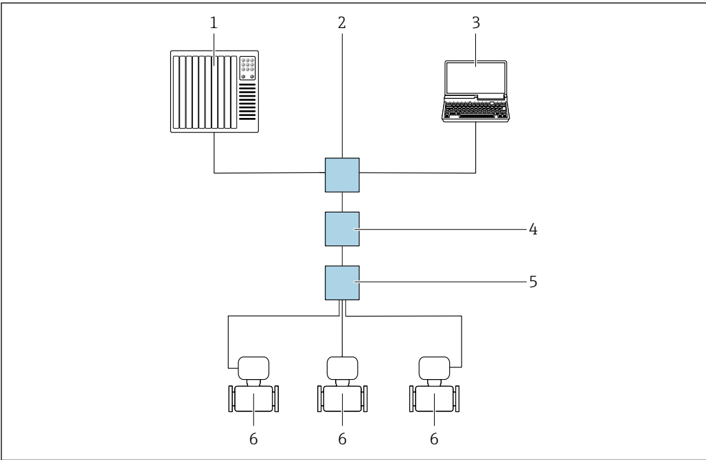
图 29 通过 Modbus TCP + Ethernet-APL 通信进行远程操作 (有源信号)
