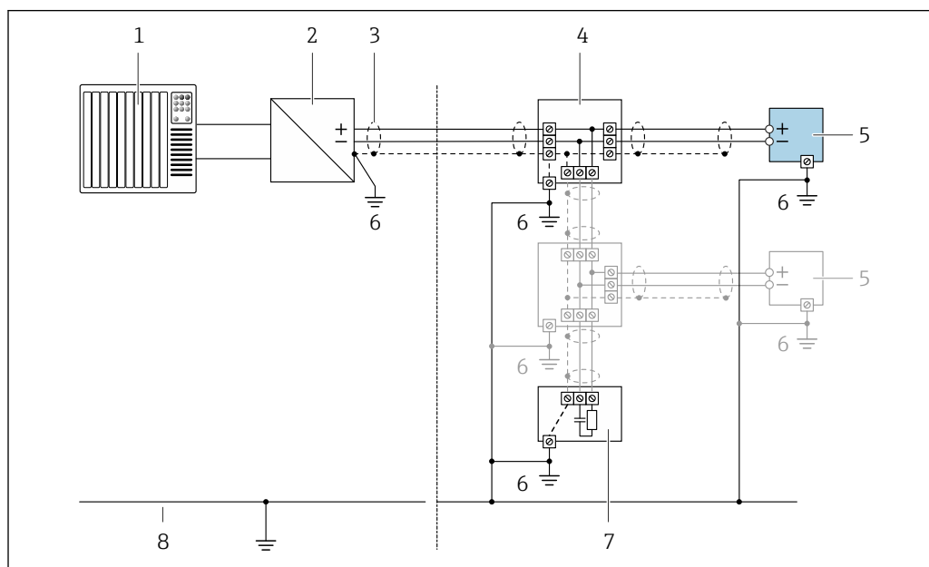
10 接线实例: FOUNDATION Fieldbus
