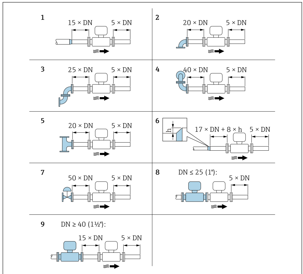
图 12 使用不同节流装置时的最小前后直管段长度
