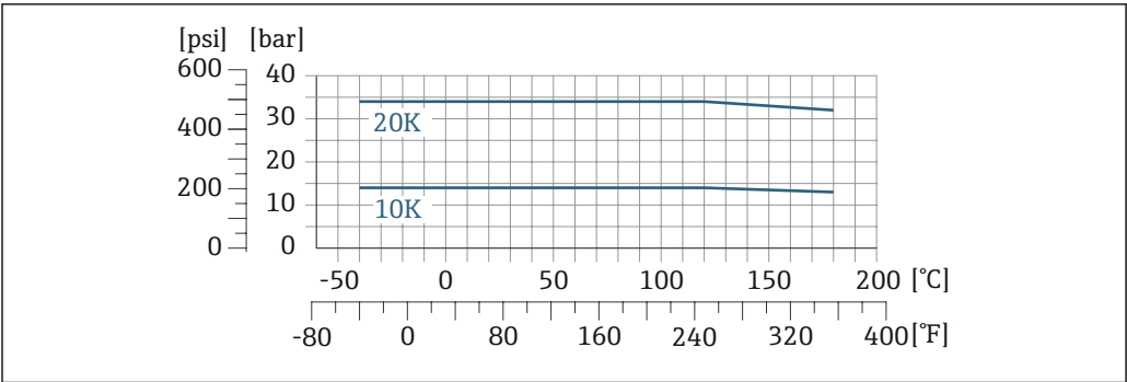
图 18 连接法兰的材质: 不锈钢 1.4404/F316/F316L, 多种材料认证
