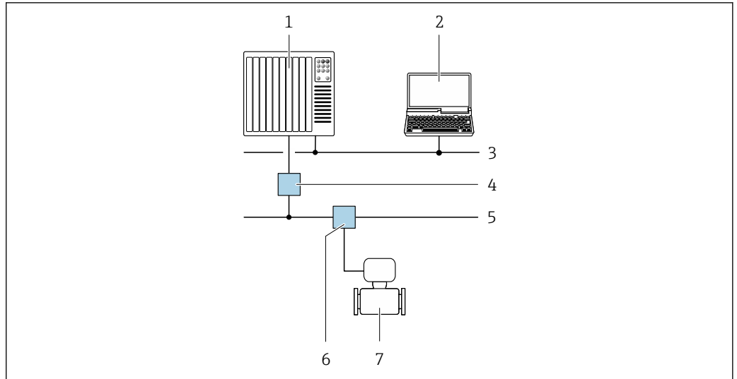
27 通过 PROFIBUS PA 网络进行远程操作
