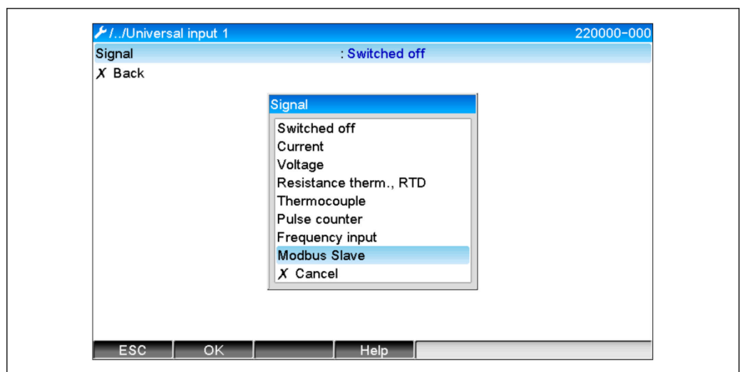
4 Ställa in universalingången till Modbus
