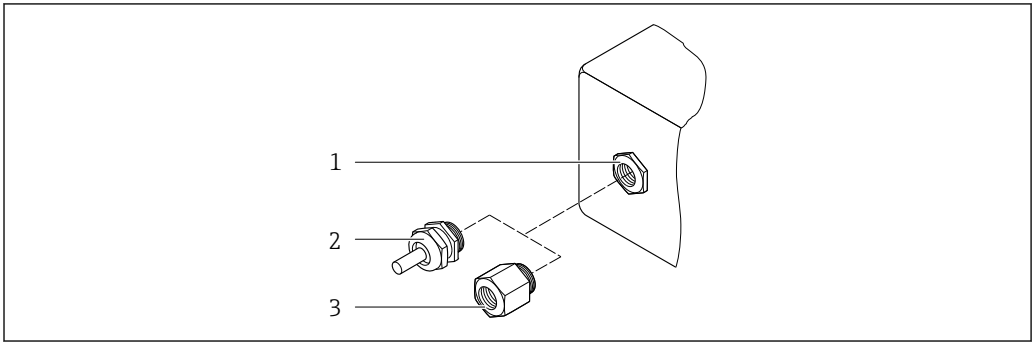
28 允许的电缆入口/缆塞
