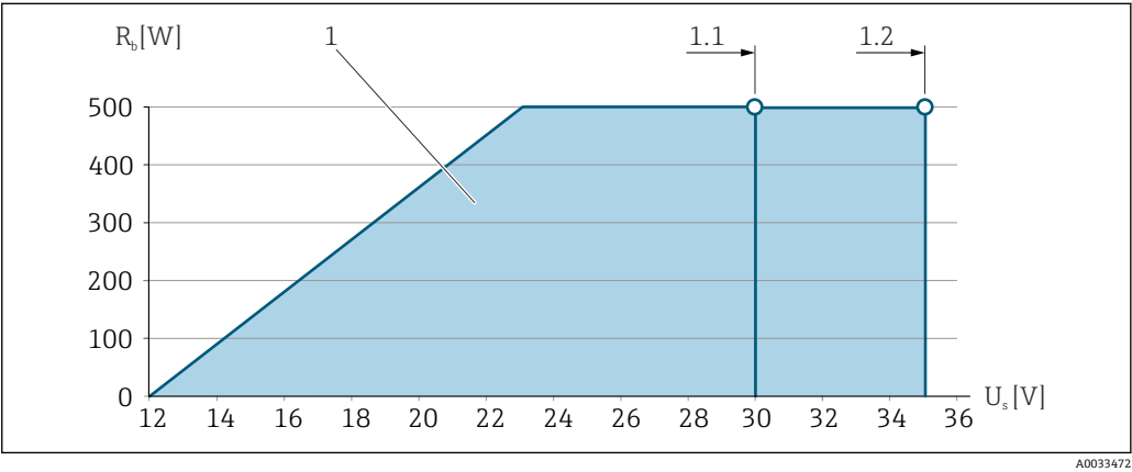
图 11 不带现场操作单元的一体式仪表的负载曲线
