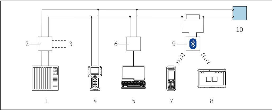
图 18 通过 HART 通信进行远程操作（无源信号）
