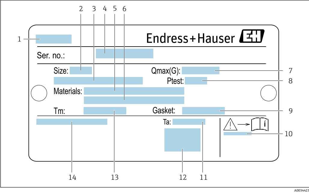
图 2 传感器的铭牌示意图 1 传感器名称 2 传感器公称口径 3 法兰公称口径/标称压力 4 序列号 5 测量管材质 6 测量管材质 7 最大允许体积流量（气体/蒸汽）： Q_{max} → 149 8 传感器测试压力：OPL 9 密封圈材质 10 《安全指南》补充文档资料代号 → 175 11 环境温度范围 12 CE 认证 13 介质温度范围 14 防护等级
