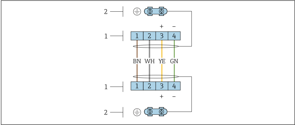
图 10 变送器墙装架中的接线腔和传感器接线盒内的接线端子
