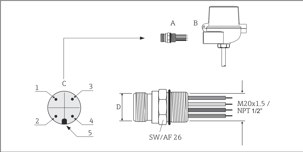
7 连接到 PROFIBUS® PA 现场总线的连接头
