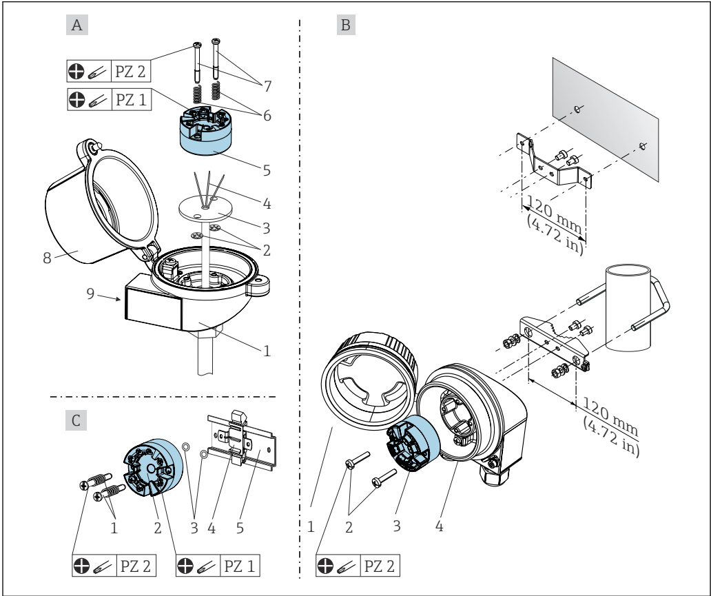
1 模块化温度变送器的安装示意图（三种安装方式）
