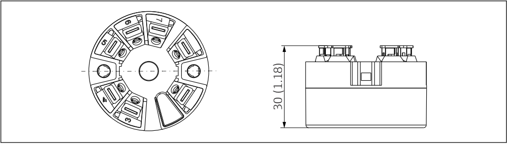
16 带直推式接线端子的设备型号。除外壳高度之外，其他尺寸参数均与带螺纹式接线端子的设备型号相同。
