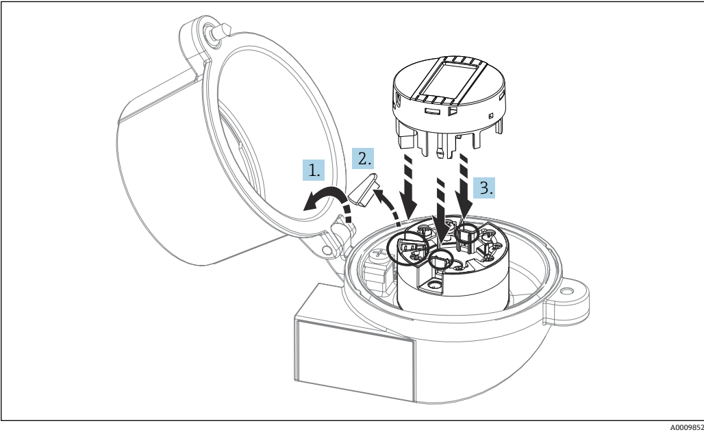
图 3 安装显示单元
