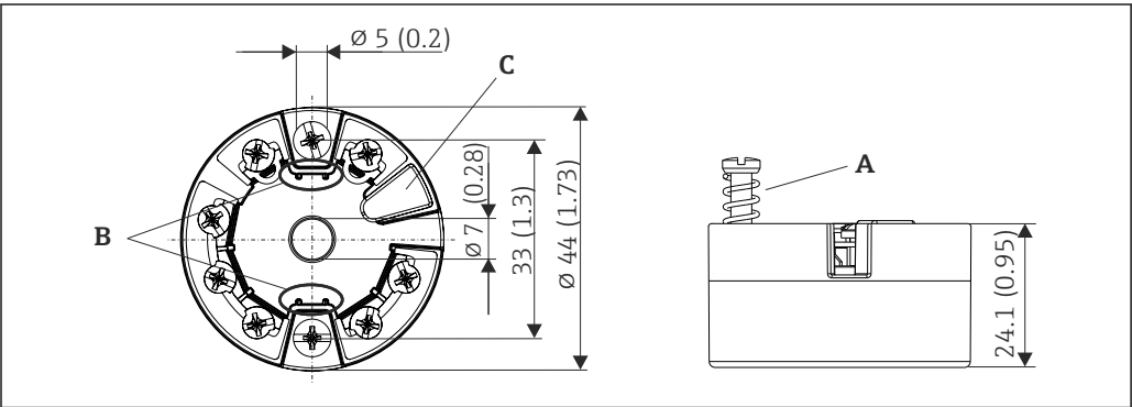
15 带螺纹式接线端子的设备型号 A 弹簧行程 L \geq 5\text{ mm} （非美标 M4 固定螺丝） B 安装部件，用于固定插拔式测量值显示单元 TID10 C 服务接口，连接测量值显示单元或调试工具
