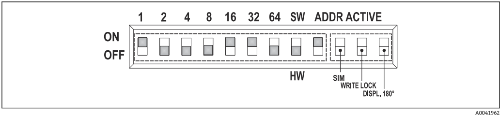
图 12 以总线地址 49 为例设置设备地址
