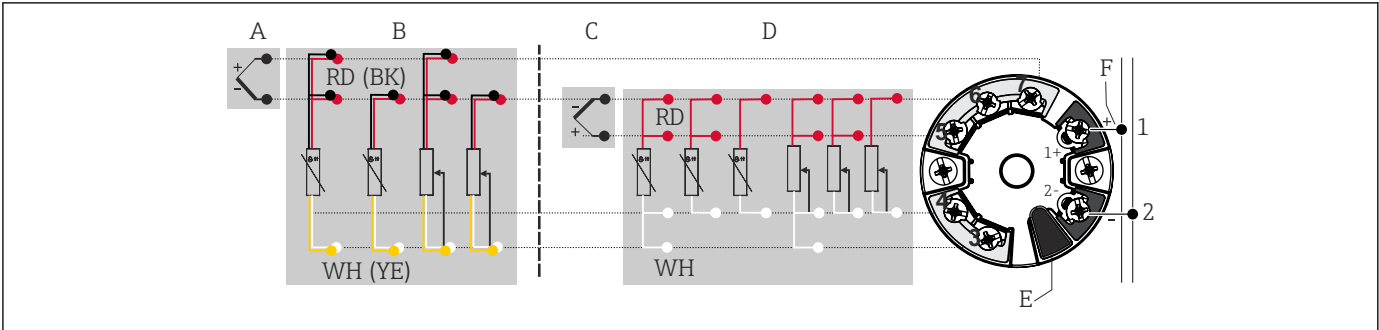
图 14 接线端子分配示意图
