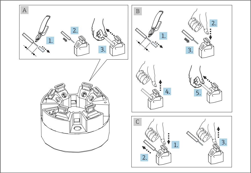
图 5 连接至直推式接线端子（以模块化温度变送器为例说明）
