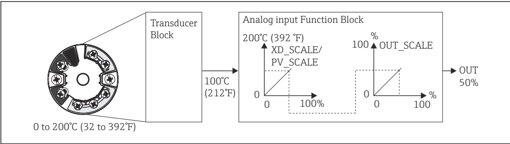
18 模拟量输入功能块比例调整步骤
