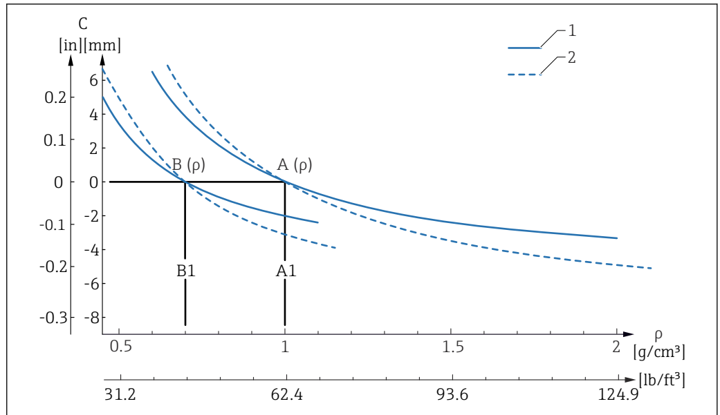
図 9 密度に対するスイッチポイント偏差
