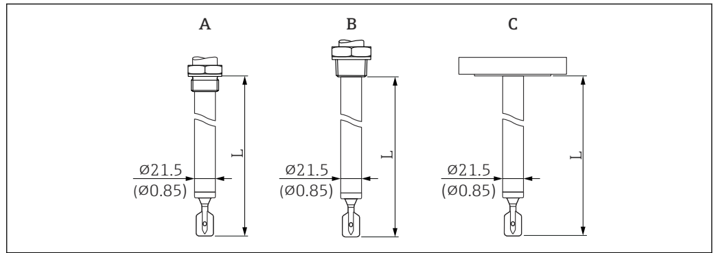
図 33 プローブ型式：伸長パイプ、ショートパイプ（センサ長 L）。測定単位 mm (in)
