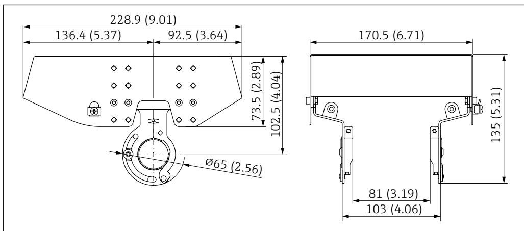
図 52 日除けカバー、SUS 316L 相当、XW112 の寸法。測定単位 mm (in)
