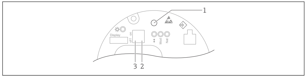
図 48 エレクトロニックインサートの操作キーおよび DIP スイッチ (FEL60P) - Ethernet-APL
