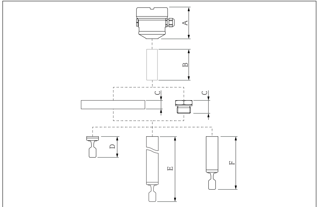
図 25 本体高さを特定するための構成品
