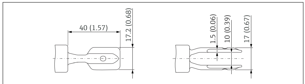
図 34 音叉部。測定単位 mm (in)
