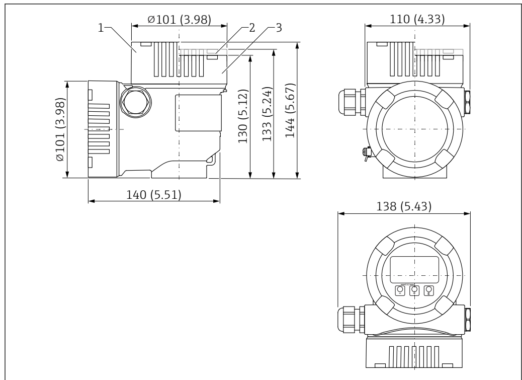
図 29 寸法 ; デュアルコンパートメントハウジング L 字型 (アルミニウム、コーティング) ; M20 カップリングおよびプラグ (プラスチック) 付き。測定単位 mm (in)
