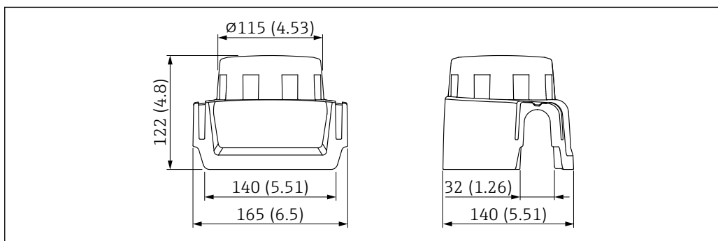
図 53 日除けカバー、プラスチック、XW111 の寸法。測定単位 mm (in)
