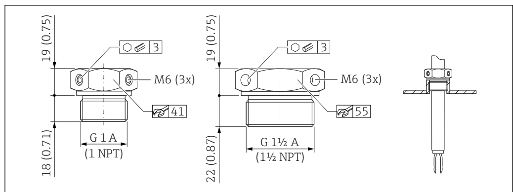
図 55 スライディングスリーブ (大気圧用： p_e = 0\text{ MPa} (0 psi))。測定単位 mm (in)
