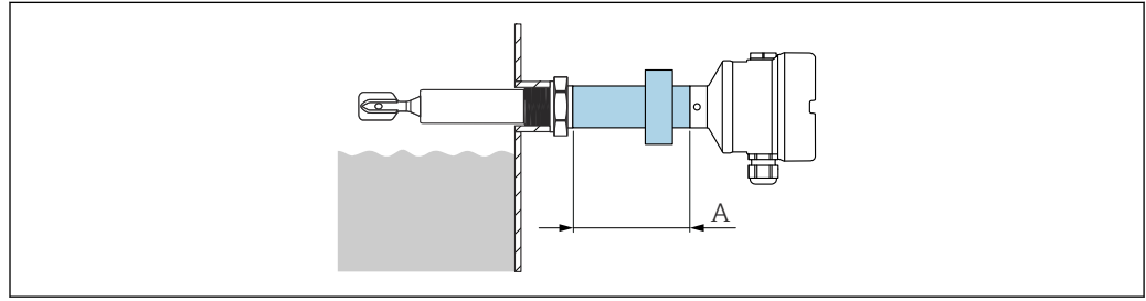
図 31 伸長パイプ用の耐圧防爆対応ガスタイトフィードスルー
