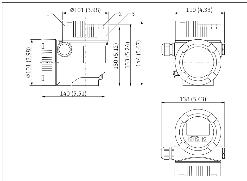
■ 30 寸法；デュアルコンパートメントハウジングL字型（SUS 316 L 相当）；M20 カップリングおよびプラグ（プラスチック）付き。測定単位 mm (in)
