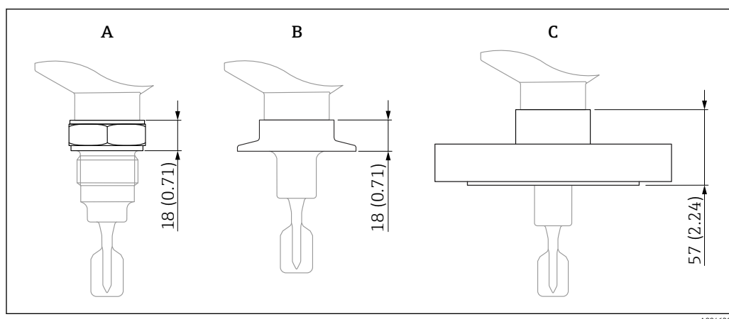
図 35 プロセス接続の最大高さ仕様。測定単位 mm (in)
