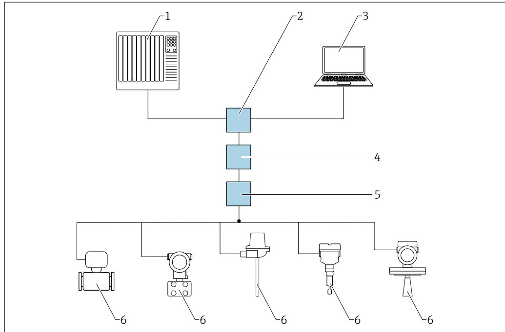
図 51 PROFINET over Ethernet-APL ネットワーク経由のリモート操作オプション：スター型トポロジー
