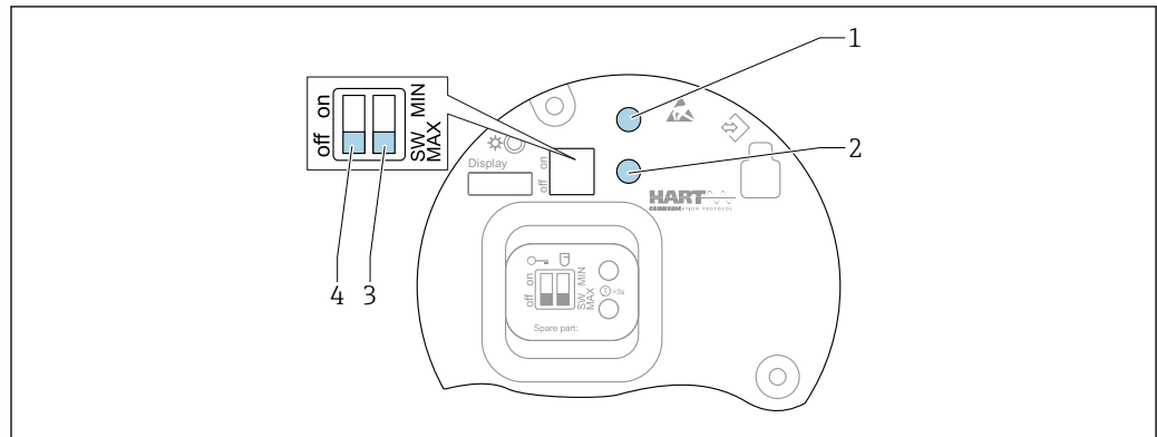
図 47 FEL60H エレクトロニックインサートの操作キーおよび DIP スイッチ
