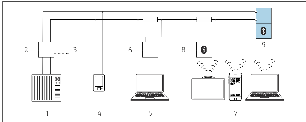
図 50 HART プロトコルを使用したリモート操作オプション
