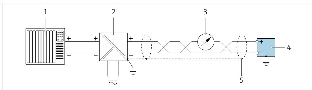
28 Пример подключения для токового выхода 4 до 20 мА (пассивного) с HART
