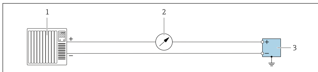
20 Пример подключения для токового выхода 4 до 20 мА (активного)
