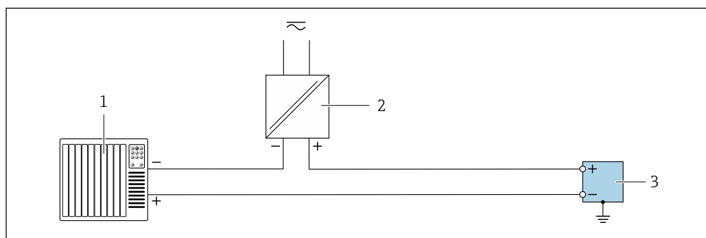
25 Пример подключения для релейного выхода
