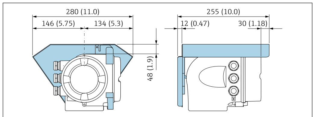
12 Защитный козырек от погодных явлений для Proline 500 – единица измерения- мм (дюймах)
