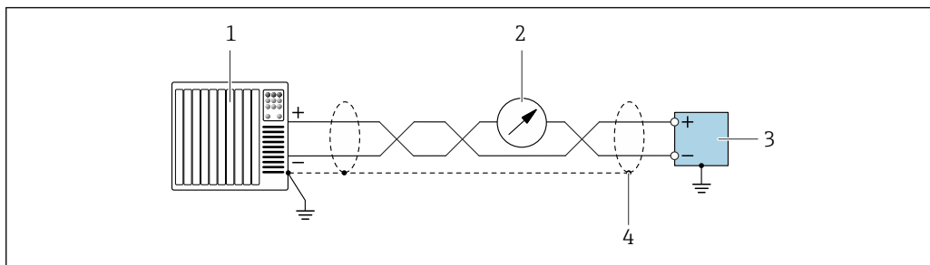
27 Пример подключения для токового выхода 4 до 20 мА (активного) с HART
