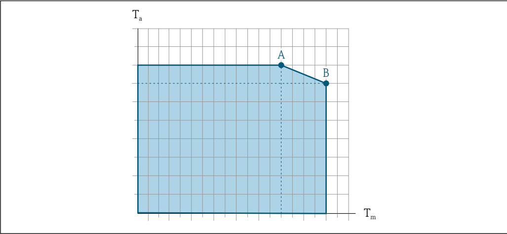
46 Пример зависимости, значения приведены в таблице. T a Температура окружающей среды T m Температура технологической среды A Максимально допустимая температура среды T m при T a max = 60 °C (140 °F); более высокие значения температуры технологической среды T m требуют снижения температуры окружающей среды T a B Максимально допустимая температура окружающей среды T a при максимальной установленной температуре среды T m для сенсора
