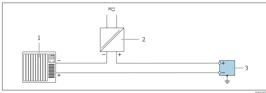
24 Пример подключения для импульсного/частотного/релейного выхода (пассивного)
