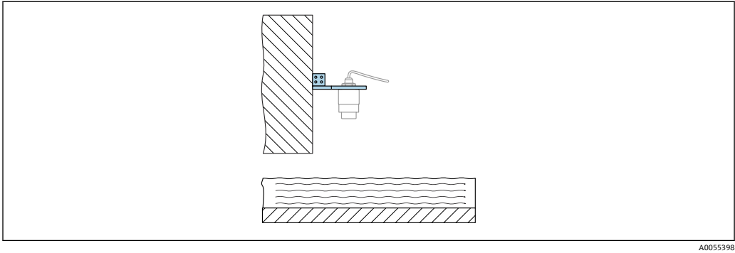
图 19 使用悬臂和墙装架安装，悬臂可以旋转和调节（例如在水渠正上方定位设备）
