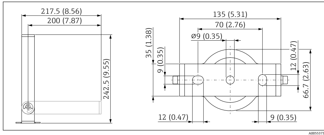
图 40 安装架的外形尺寸示意图。测量单位 mm (in)
