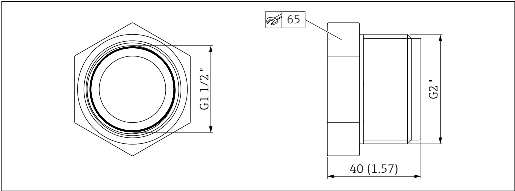
33 UNI 转接头的外形尺寸
