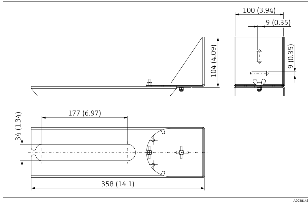
图 51 旋转安装架的外形尺寸。测量单位 mm (in)
