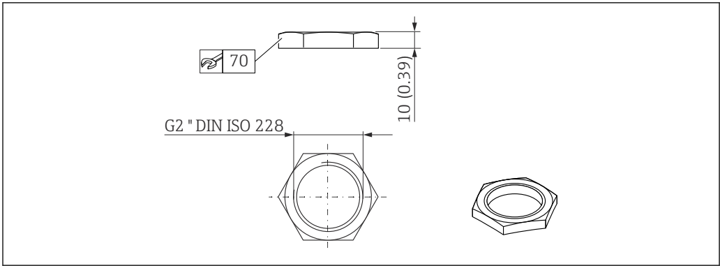
32 锁紧螺母的外形尺寸。测量单位 mm (in)
