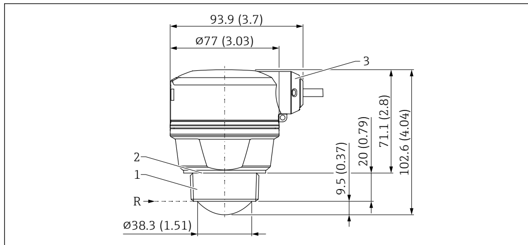
图 22 外形尺寸示意图；40 mm (1.5 in) 口径天线，侧面电缆入口。测量单位 mm (in)
