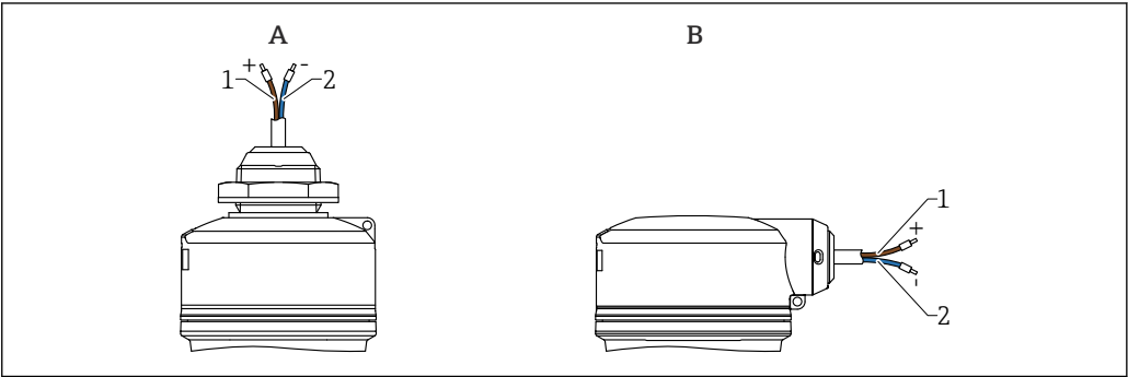
3 电缆分配 A 顶部电缆入口 B 侧面电缆入口 1 正极，棕线 2 负极，蓝线
