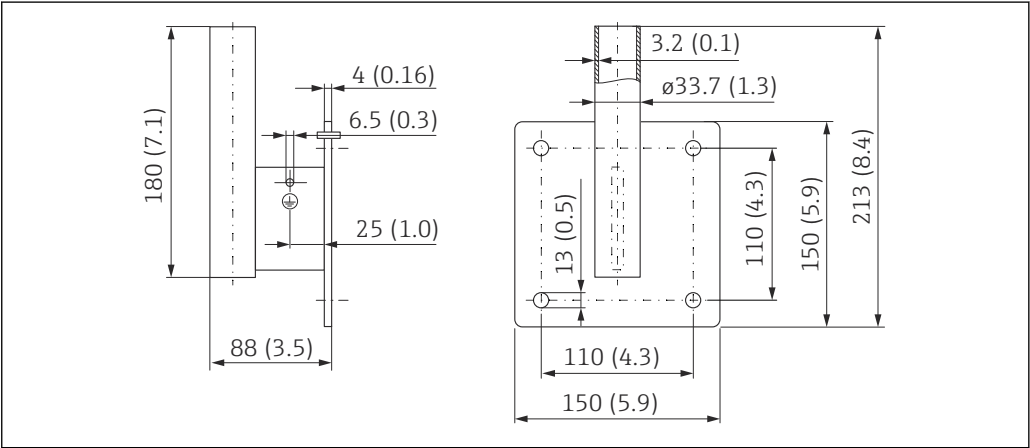
50 墙装架的外形尺寸。测量单位 mm (in)
