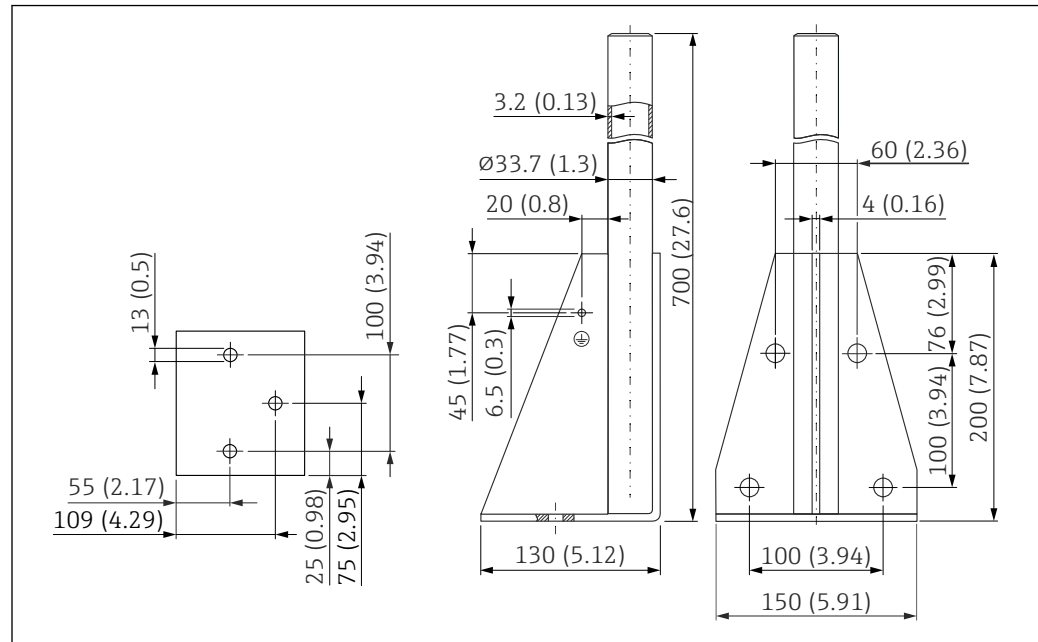
图 48 外形尺寸。测量单位 mm (in)
