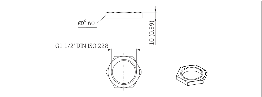
31 锁紧螺母的外形尺寸。测量单位 mm (in)
