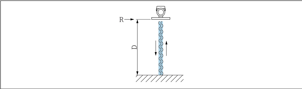
图 1 FMCW 原理：发送和反射连续波
