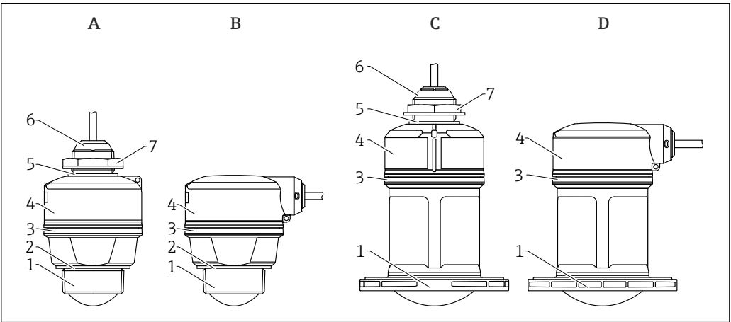
图 26 设备设计
