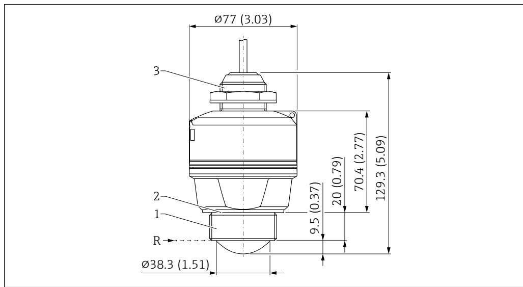
图 21 外形尺寸示意图；40 mm (1.5 in) 口径天线，顶部电缆入口。测量单位 mm (in)
