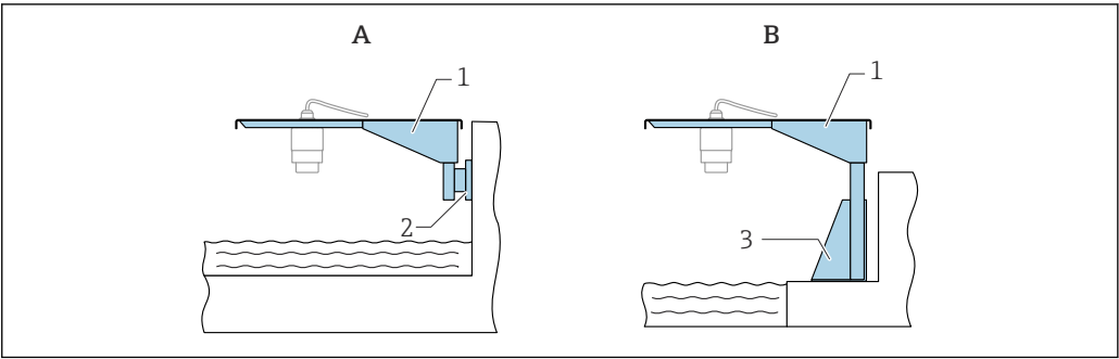
42 传感器电缆入口过程连接的安装方式
