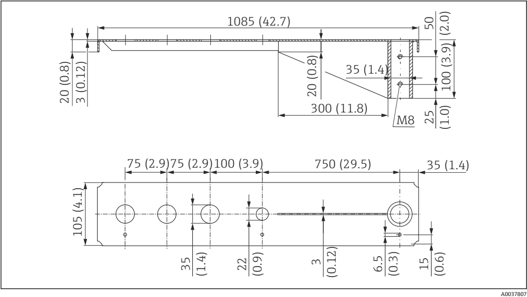
图 44 1000 mm 旋转悬臂的外形尺寸（安装在传感器电缆入口过程连接上）。测量单位 mm (in)
