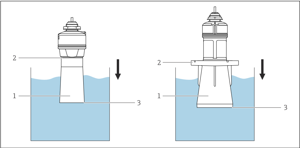
15 防溢管的功能
