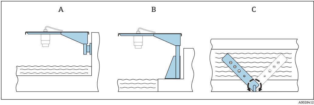
图 18 使用悬臂安装（可旋转） A 使用悬臂和墙装架安装（侧视图） B 使用悬臂和安装架安装（侧视图） C 悬臂可以旋转（例如在水渠正上方定位设备）（俯视图）
