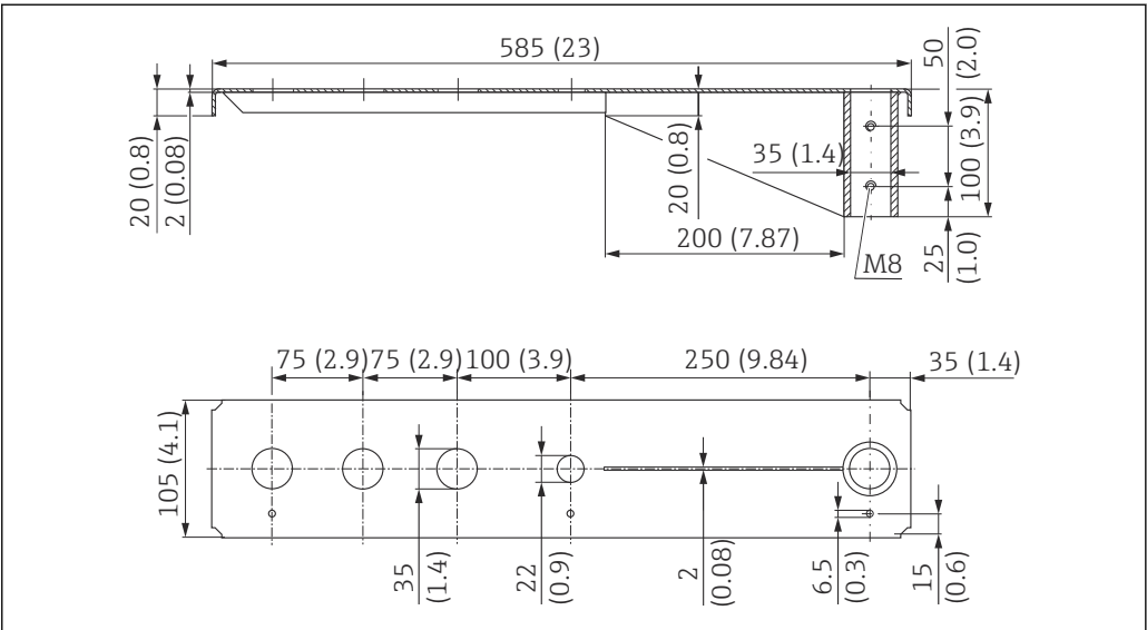
43 500 mm 旋转悬臂的外形尺寸（安装在传感器电缆入口过程连接上）。测量单位 mm (in)
