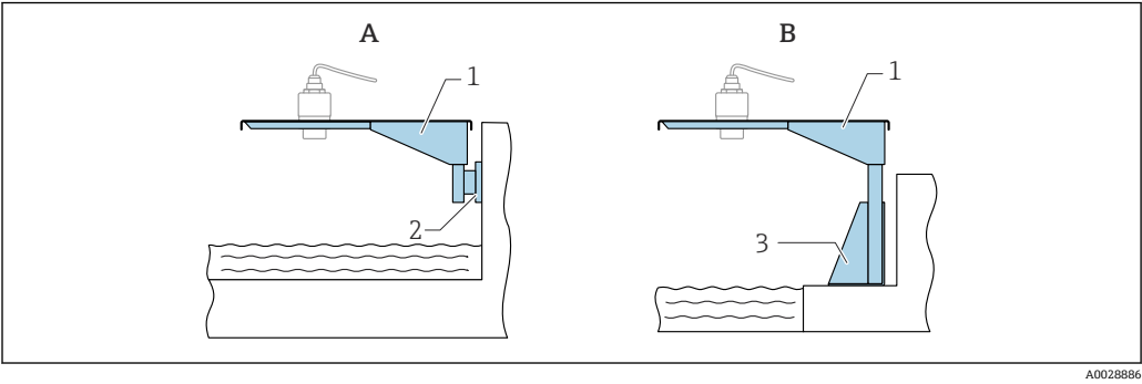
图 45 传感器天线端过程连接的安装方式
