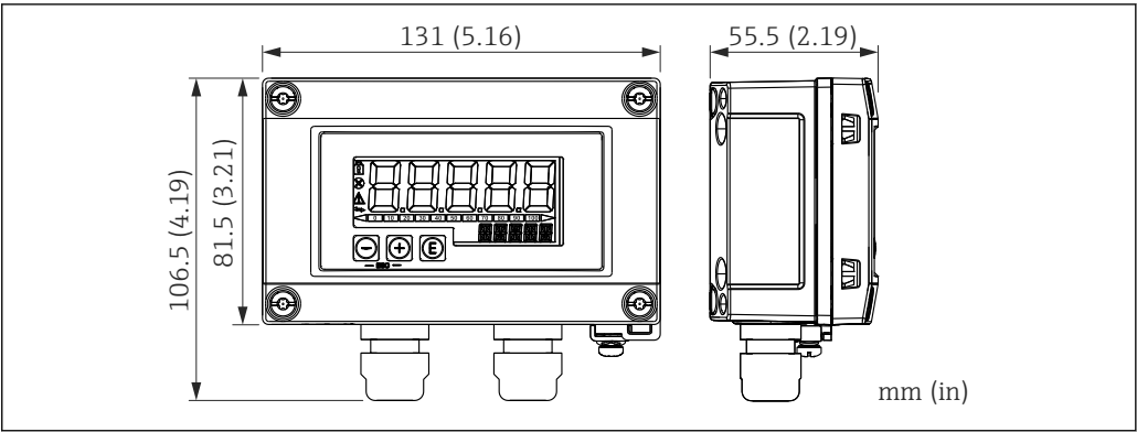
60 RIA15 (现场型外壳) 的外形尺寸。测量单位 mm (in)
