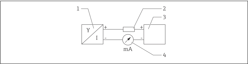
4 HART 连接功能框图 1 HART 设备 2 HART 通信电阻 3 电源 4 万用表或电流表
