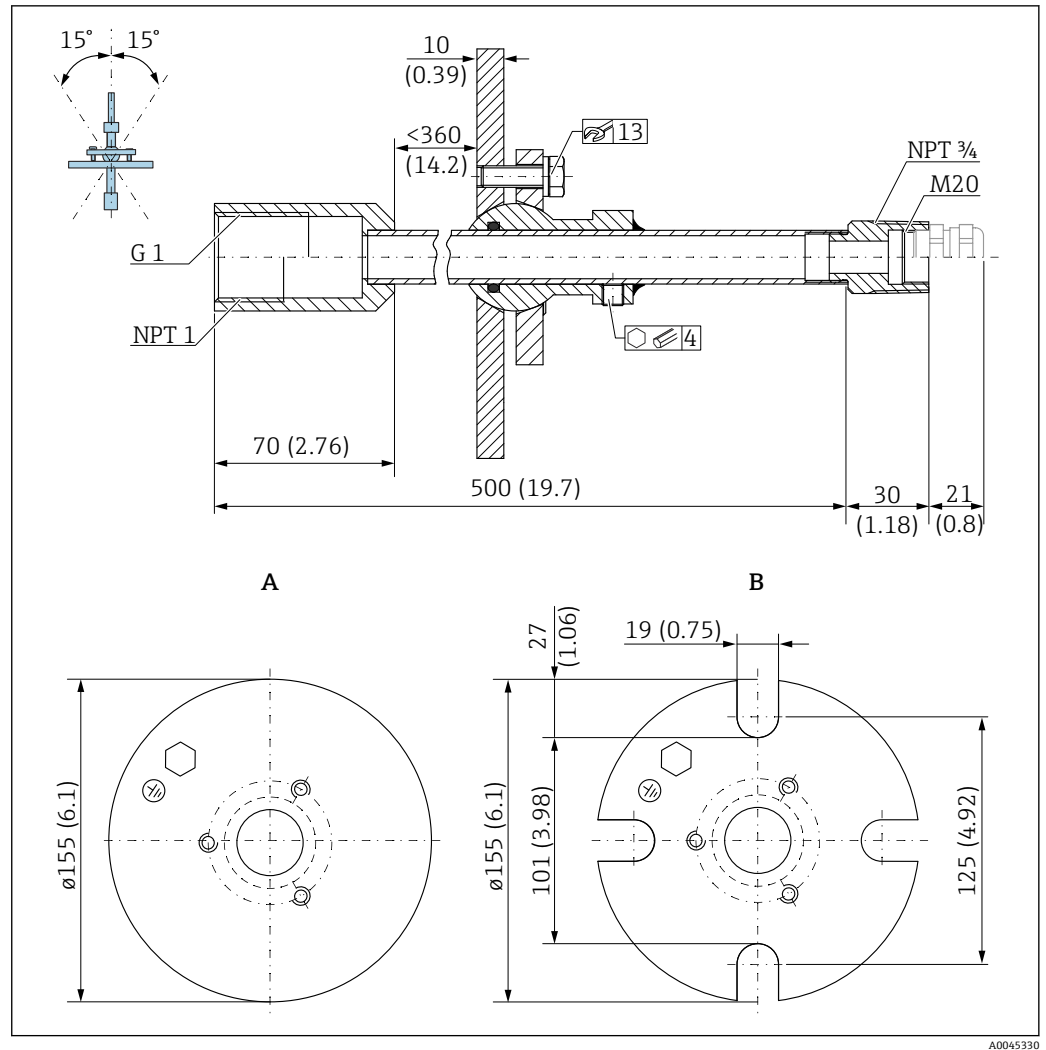
52 外形尺寸。测量单位 mm (in)
