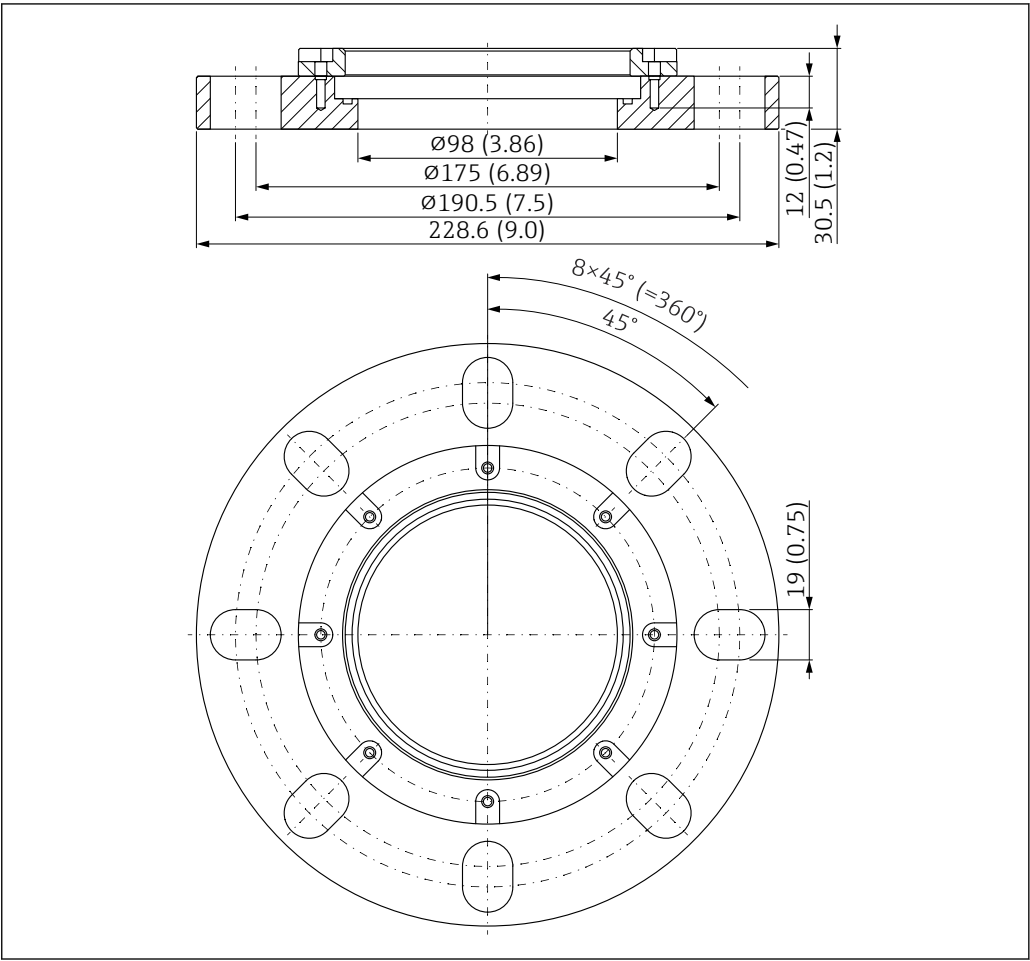
54 UNI 4"/DN100/100 松套法兰的外形尺寸示意图。测量单位 mm (in)
