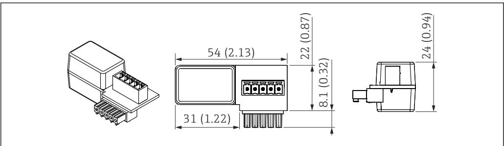
61 HART 通信电阻的外形尺寸。测量单位 mm (in)
