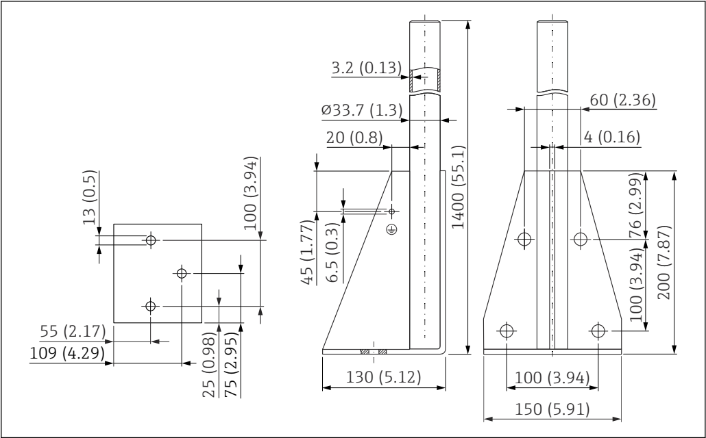
49 外形尺寸。测量单位 mm (in)
