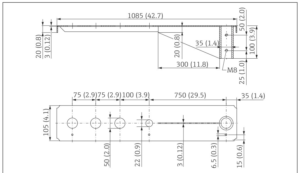
47 1000 mm 旋转悬臂的外形尺寸（安装在 G 1½"传感器天线端过程连接上）。测量单位 mm (in)
