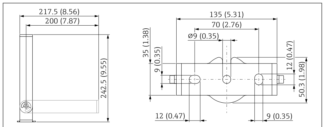
图 39 安装架的外形尺寸示意图。测量单位 mm (in)
