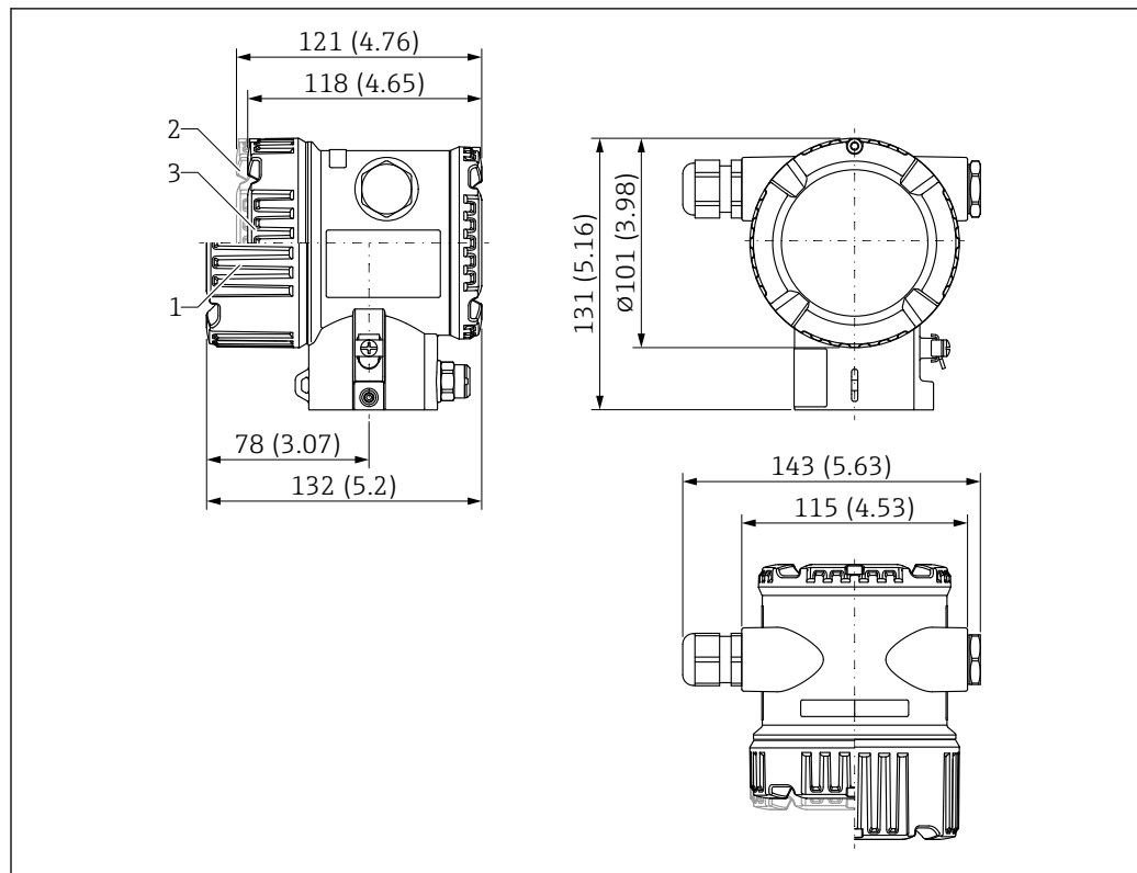
図 43 寸法 ; デュアルコンパートメントハウジング (アルミニウム、コーティング) ; M20 カップリングおよびプラグ (プラスチック) 付き。測定単位 mm (in)
