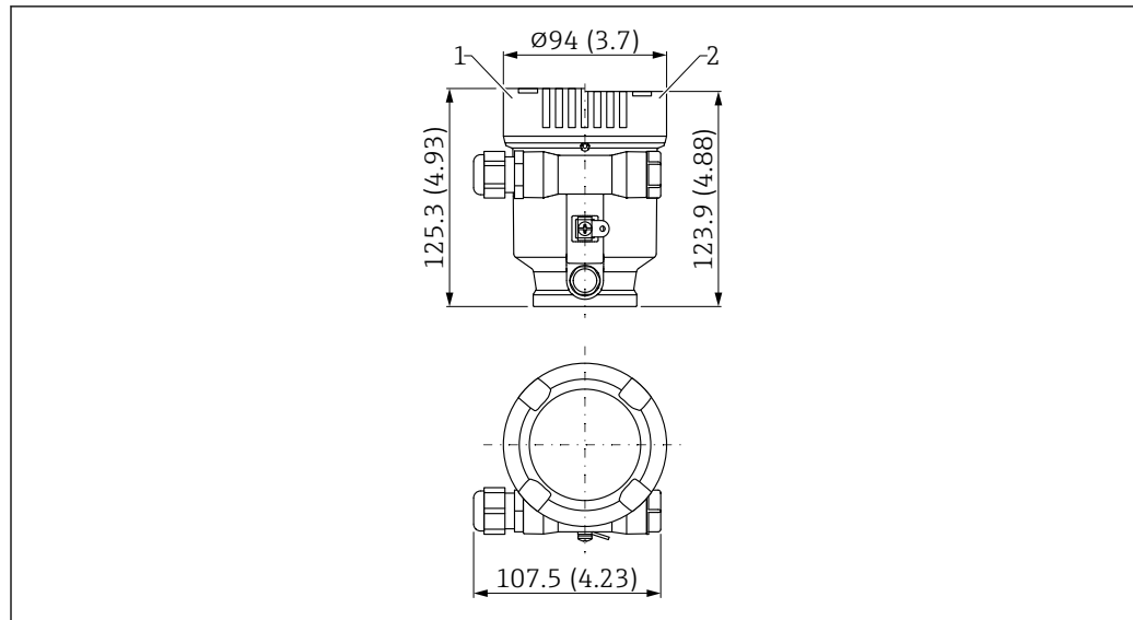
図 40 寸法 ; シングルコンパートメントハウジング (プラスチック) ; M20 カップリングおよびプラグ (プラスチック) 付き。測定単位 mm (in)
