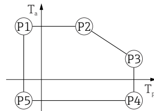
図 23 アルミニウムハウジング ; コーティング ; プロセス温度 -20 \sim +200 \text{ }^{\circ}\text{C} ( -4 \sim +392 \text{ }^{\circ}\text{F} )
