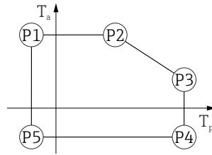
図 28 SUS 316L 相当製ハウジング ; プロセス温度 -20~+150 °C (-4~+302 °F)
