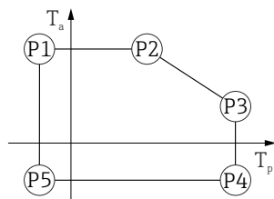
図 18 プラスチックハウジング ; プロセス温度 -40 \sim +150^{\circ}\text{C} ( -40 \sim +302^{\circ}\text{F} )
