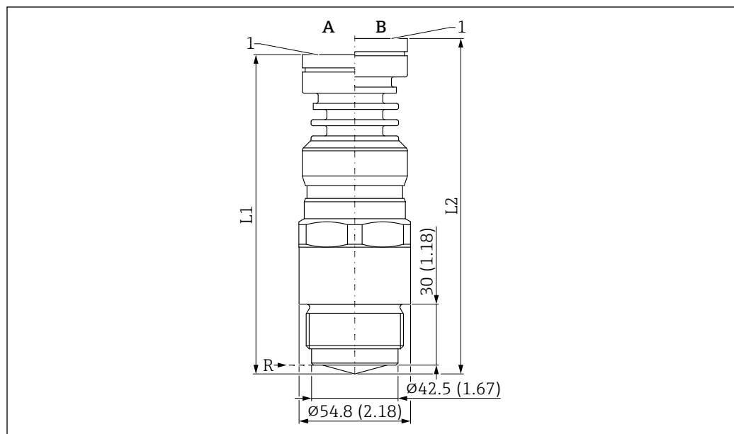
図 57 寸法 ; 内蔵アンテナ、PEEK、40 mm (1.5 in) ; プロセス接続、ネジ 1-½"。測定単位 mm (in)
