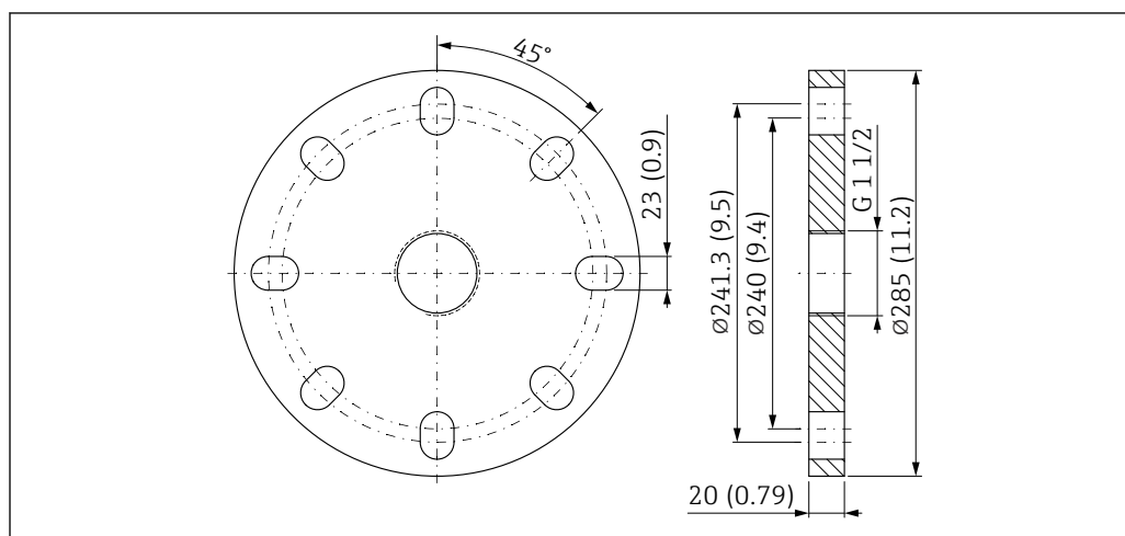
図 50 UNI フランジ 6"/DN150/150A の寸法。測定単位 mm (in)
