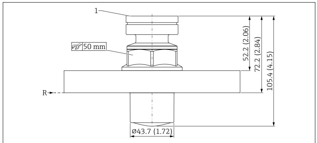
図 47 被覆アンテナ (PVDF、40 mm (1.5 in)、プロセス接続 UNI フランジ) の寸法。測定単位 mm (in)
