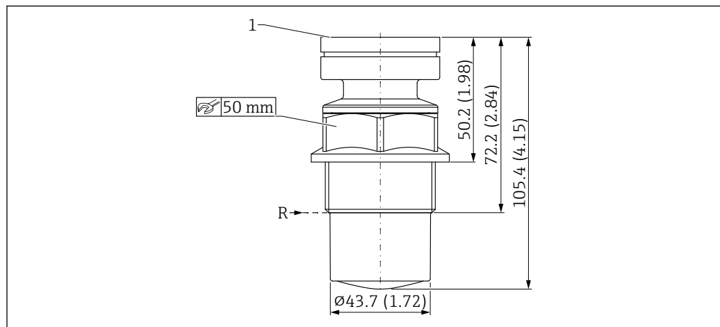
図 46 寸法 ; 被覆アンテナ、PVDF、40 mm (1.5 in)。測定単位 mm (in)
