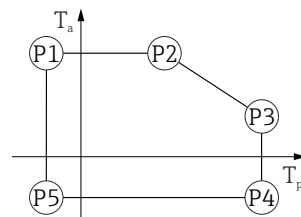
図 24 アルミニウムハウジング ; コーティング ; プロセス温度 -40 \sim +80 \text{ }^{\circ}\text{C} ( -40 \sim +176 \text{ }^{\circ}\text{F} )
