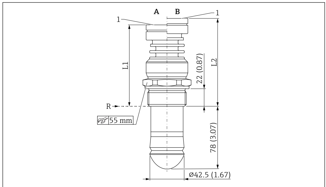
■ 51 ドリップオフアンテナ 50 mm (2 in) (ネジ込みプロセス接続) の寸法
