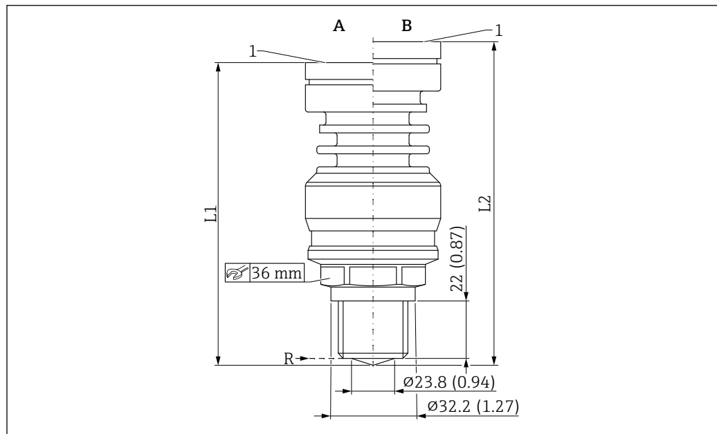
図 56 寸法 ; 内蔵アンテナ、PEEK、20 mm (0.75 in) ; プロセス接続、ネジ ¾"。測定単位 mm (in)
