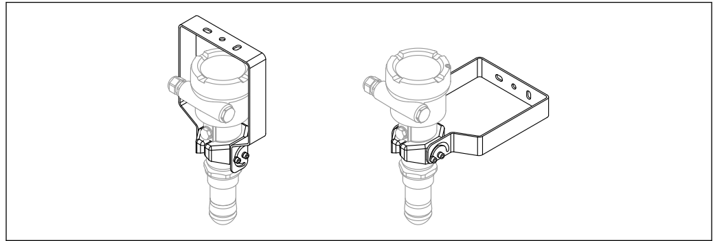
図 66 調整可能な取付ブラケット FMR6xB ; 天井または壁面取付け
