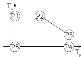
図 15 プラスチックハウジング；プロセス温度 0～+80 °C (+32～+176 °F)、CSA C/US 認定取得
