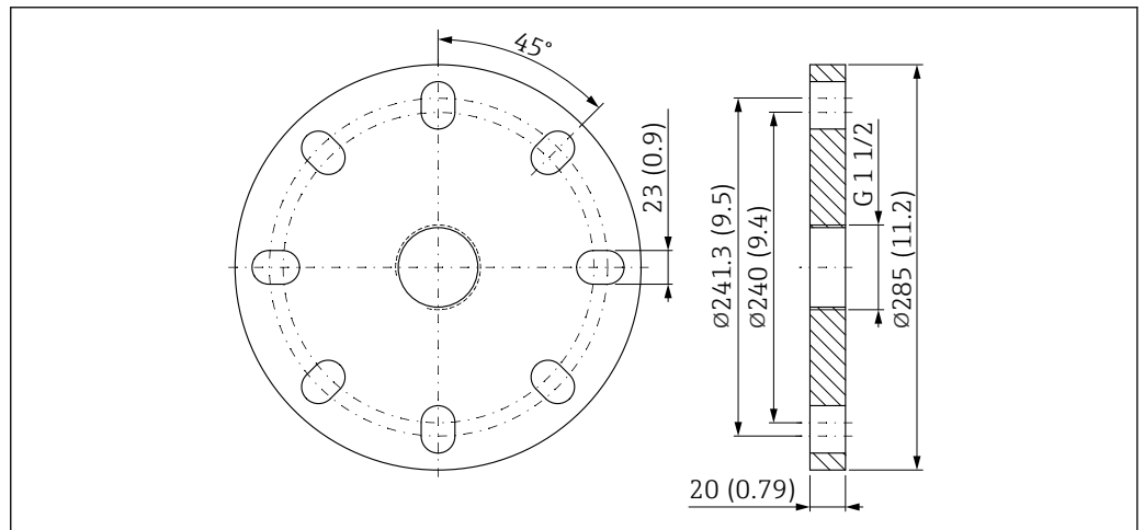
図 55 UNI フランジ 6"/DN150/150A の寸法。測定単位 mm (in)
