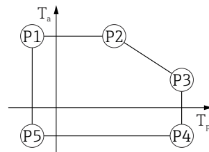
図 22 アルミニウムハウジング ; コーティング ; プロセス温度 -20 \sim +150 \text{ }^{\circ}\text{C} ( -4 \sim +302 \text{ }^{\circ}\text{F} )
