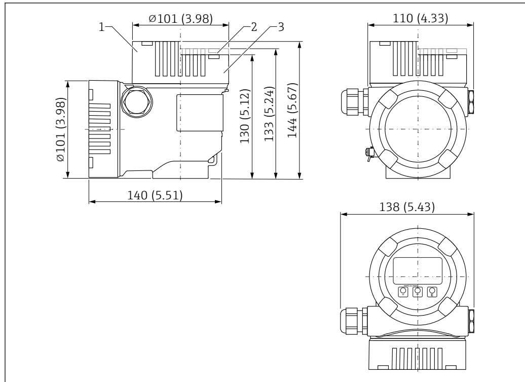
図 45 寸法 ; デュアルコンパートメントハウジング L 字型 (SUS 316 L 相当) ; M20 カップリングおよびプラグ (プラスチック) 付き。測定単位 mm (in)
