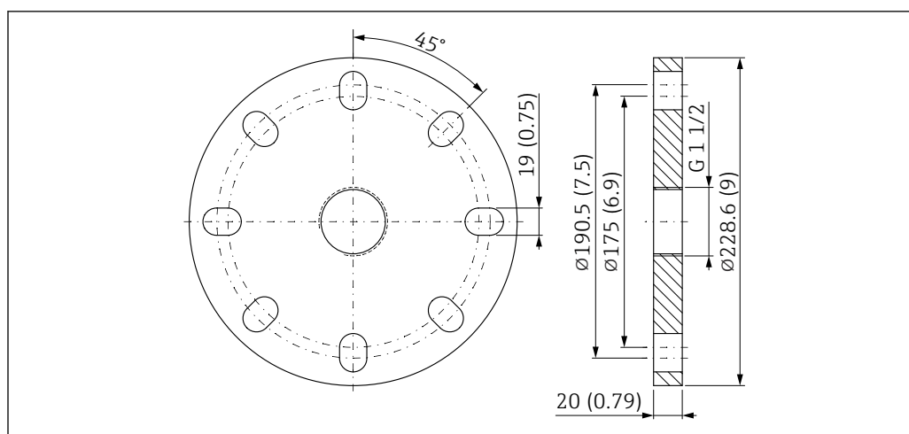
図 49 UNI フランジ 4"/DN100/100A の寸法。測定単位 mm (in)
