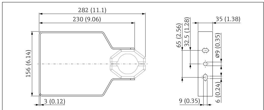
図 67 寸法 ; 調整可能な取付ブラケット FMR6xB。測定単位 mm (in)
