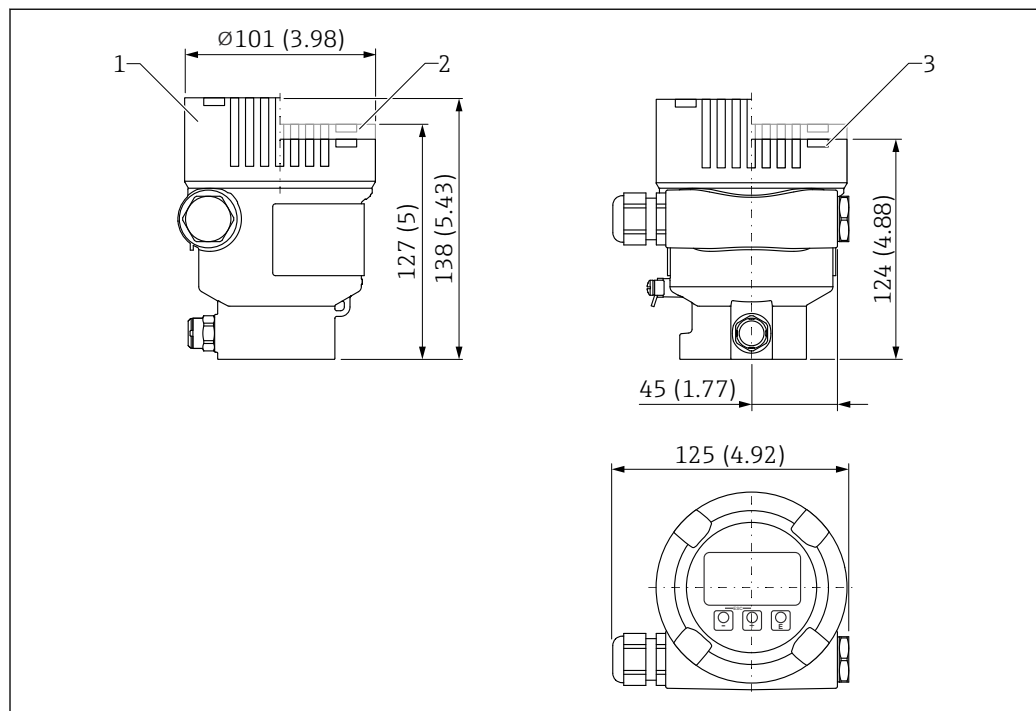
図 41 寸法 ; シングルコンパートメントハウジング (アルミニウム、コーティング) ; M20 カップリングおよびプラグ (プラスチック) 付き。測定単位 mm (in)
