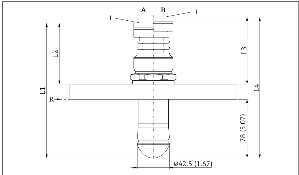
図 52 ドリップオフアンテナ 50 mm (2 in) (UNI フランジプロセス接続) の寸法。測定単位 mm (in)
