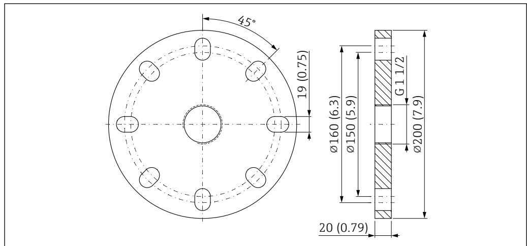
図 53 UNI フランジ 3"/DN80/80A の寸法。測定単位 mm (in)
