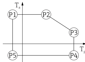
図 30 SUS 316L 相当製ハウジング ; プロセス温度 -40~+80 °C (-40~+176 °F)
