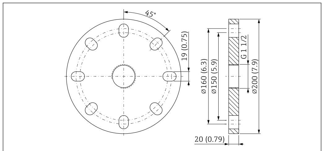
図 48 UNI フランジ 3"/DN80/80A の寸法。測定単位 mm (in)
