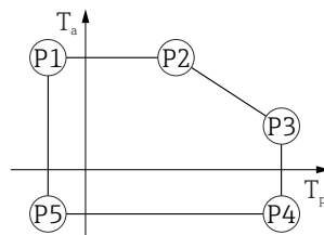
図 36 SUS 316L 相当製ハウジング、サニタリ仕様；プロセス温度 -40\sim+80\text{ }^{\circ}\text{C} ( -40\sim+176\text{ }^{\circ}\text{F} )
