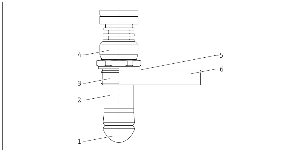
図 59 材質；ドリップオフアンテナ 50 mm (2 in)
