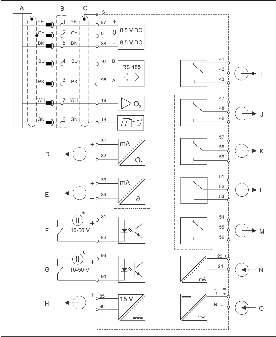
10 Raccordement électrique de l'Liquisys M COM223/253 dans la version WX ou WS
