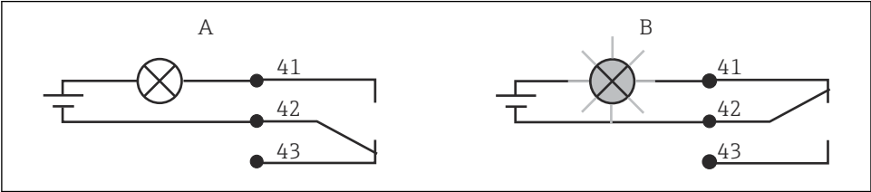
14 Commutation de sécurité recommandée pour le contact d'alarme
