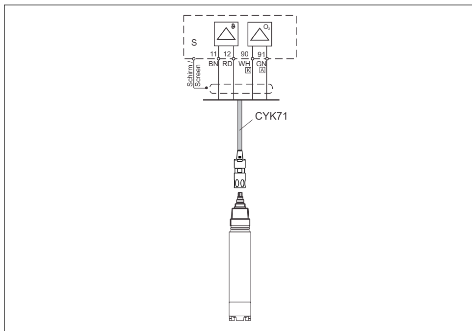
9 Exemple de raccordement : COS41 avec câble CYK71
