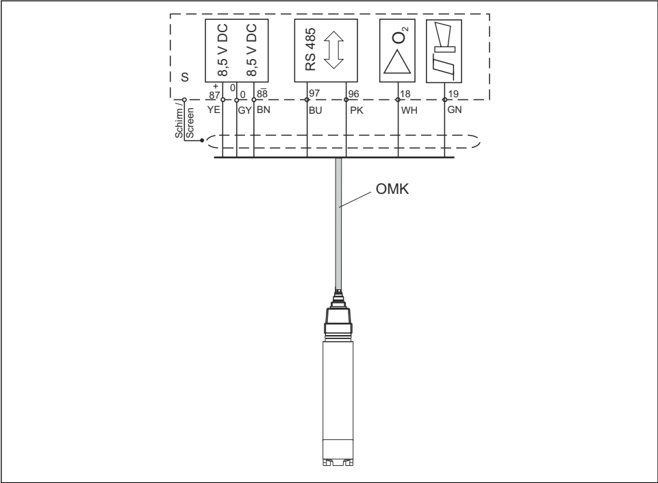
13 Exemple de raccordement : COS31/71 avec câble OMK
