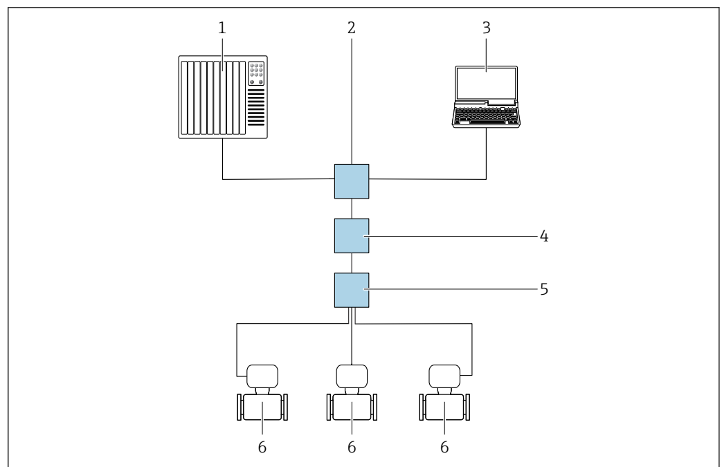
23 Opzioni per il funzionamento a distanza mediante rete APL
