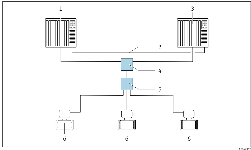
25 Esempio della struttura di un sistema ridondante (S2): topologia a stella
