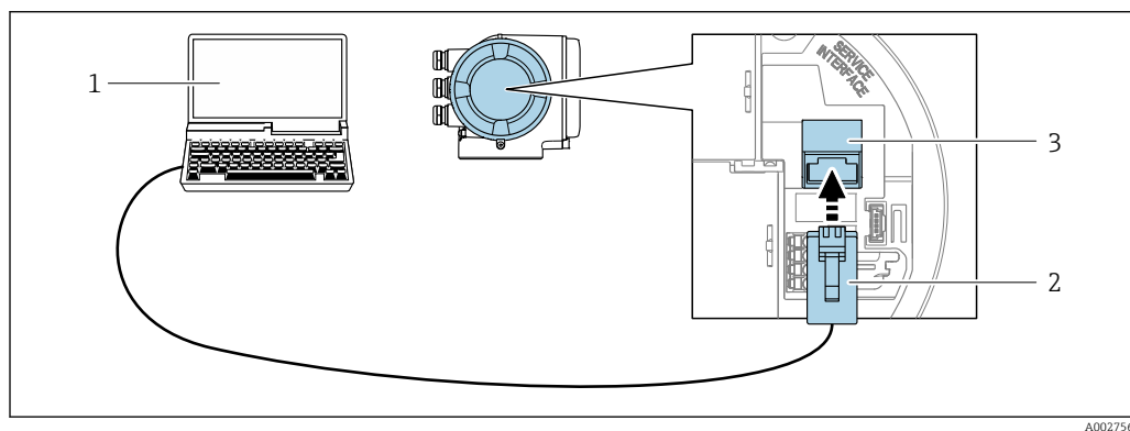
24 Connessione mediante interfaccia service (CDI-RJ45)
