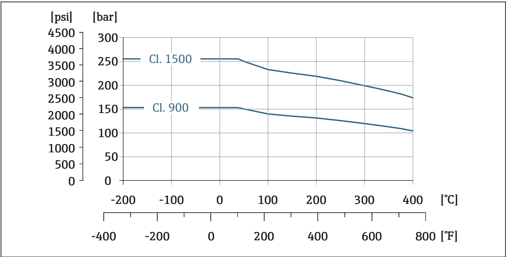
图 17 连接法兰的材质：不锈钢 1.4404/F316/F316L，多种材料认证
