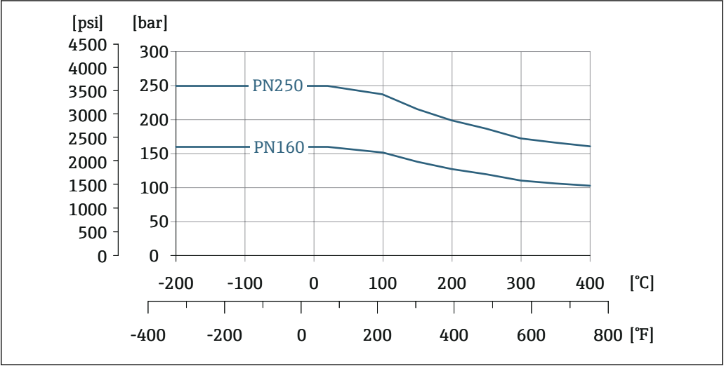
16 连接法兰和焊接连接的材质：铸造不锈钢 1.4404/F316/F316L，多种材料认证
