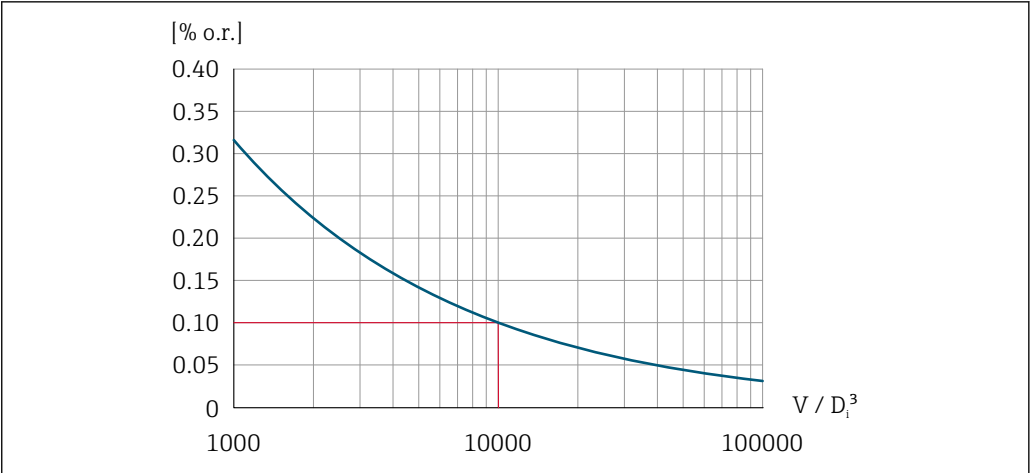
图 11 重复性 = 0.1 % o.r., 体积流量测量值[m³] of V = 10000 \cdot D_i^3
