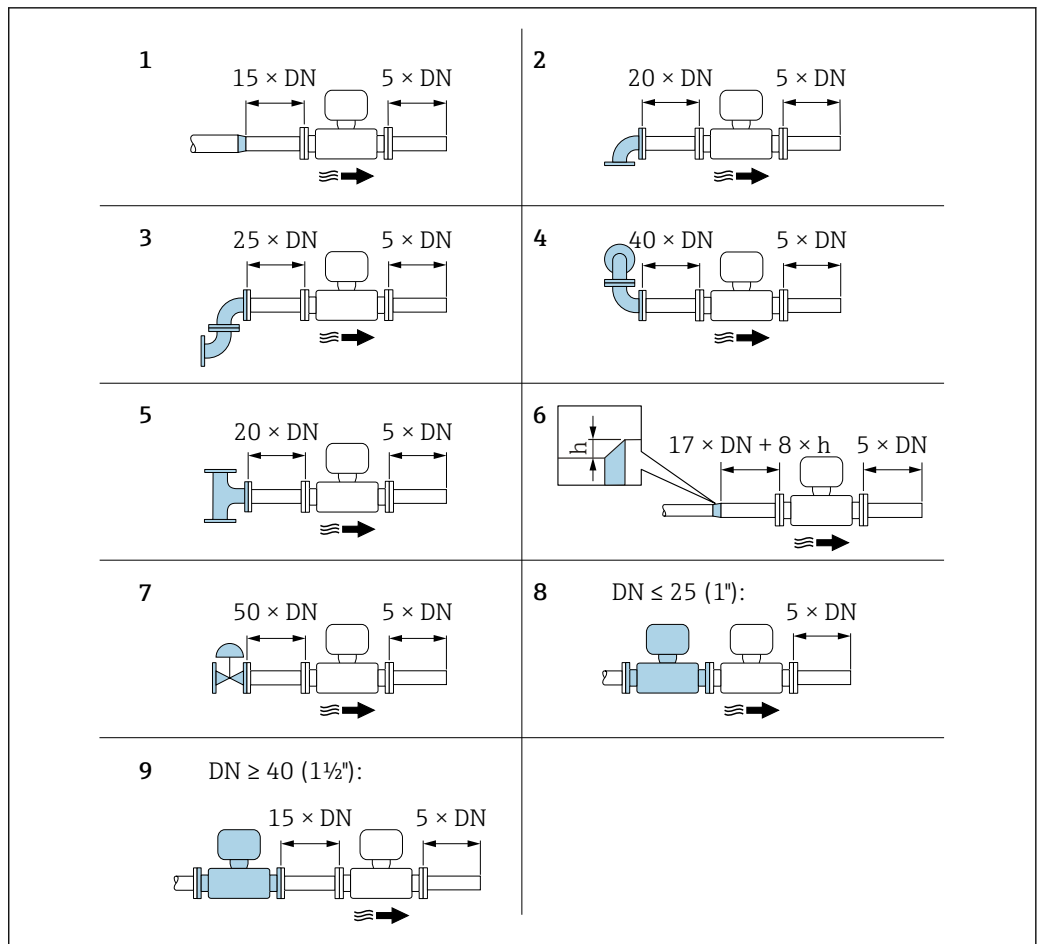
12 使用不同节流装置时的最小前后直管段长度
