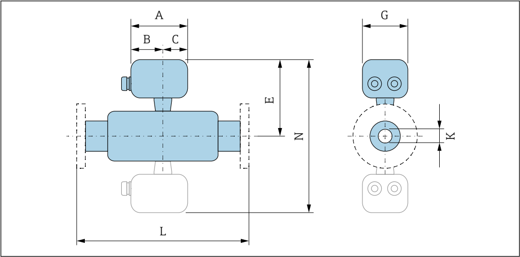
图 20 灰色区域: 双传感器型
